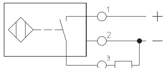
Klemmenraum
