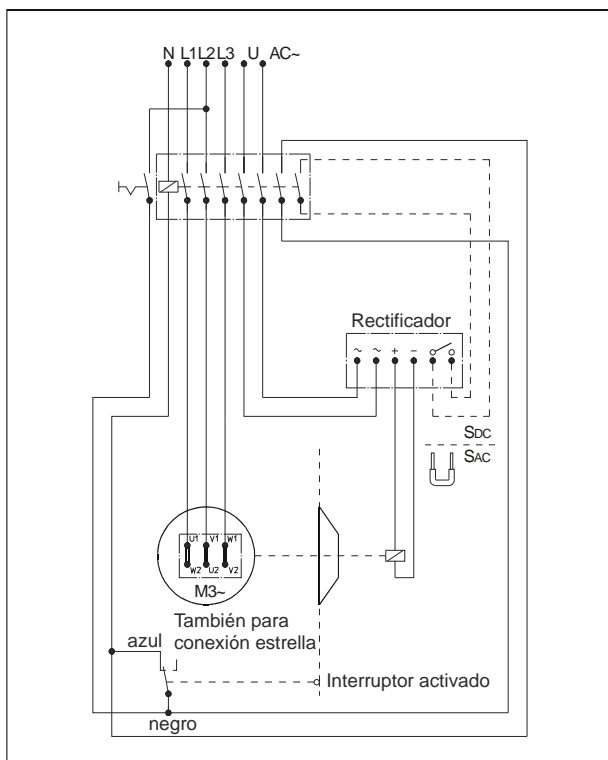
Fig. 3-2: Control de desgaste
