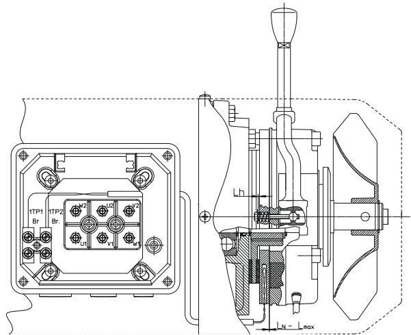
Fig. 1-1: Ventilación manual y control de temperatura
