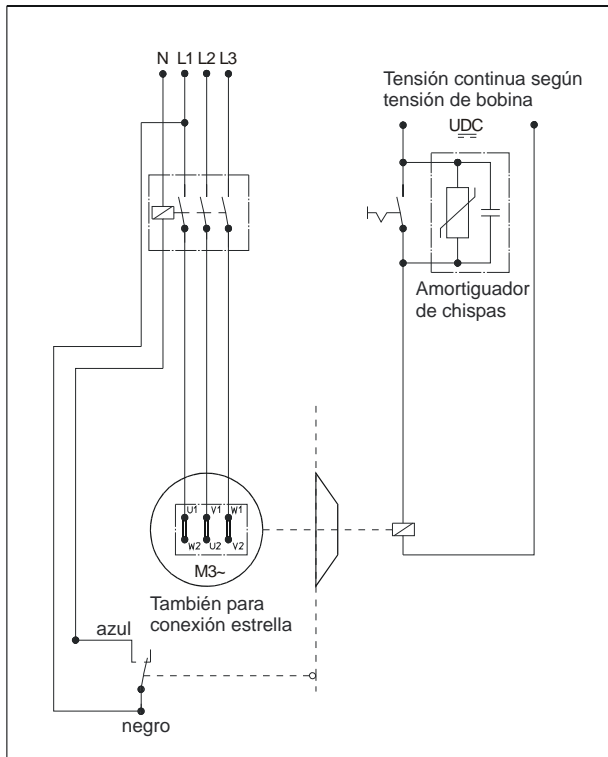
Fig. 3-1: Control de liberación
