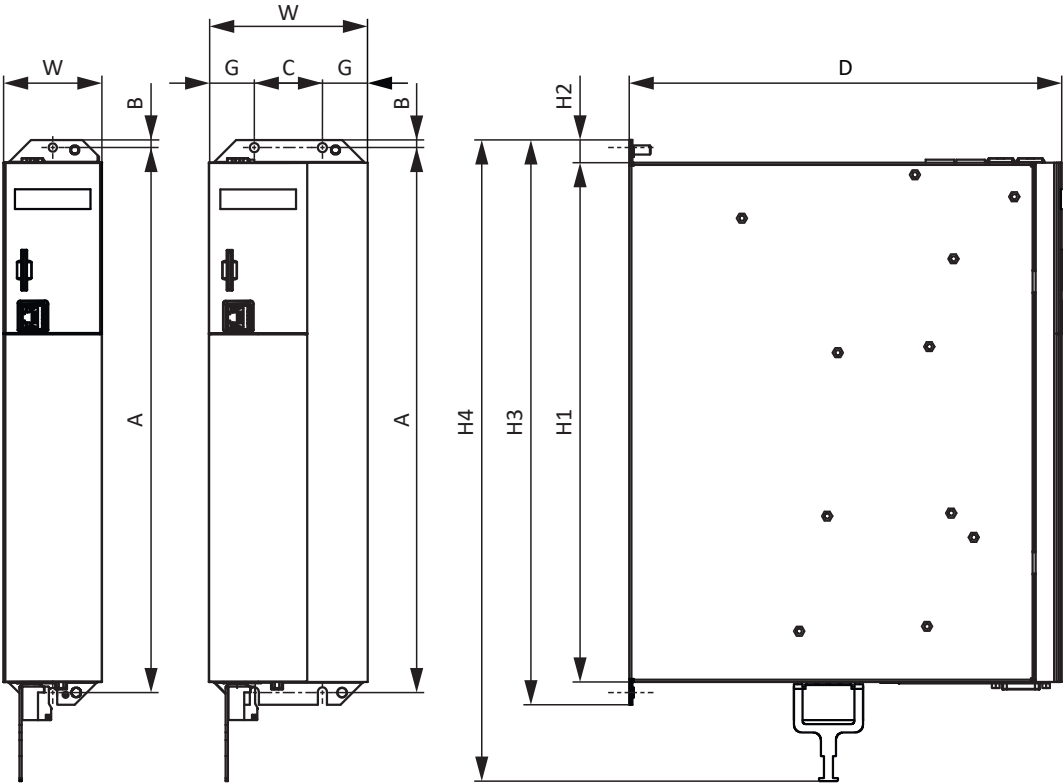
图 2: SI6 尺寸图
