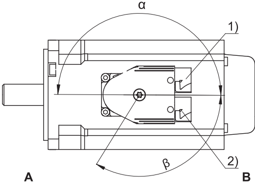
插头连接器的旋转范围 (EZ2 – EZ3 电机)
