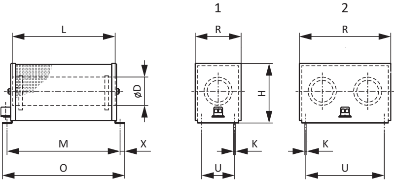
图 3: FZMU (1)、FZZMU (2) 尺寸图
