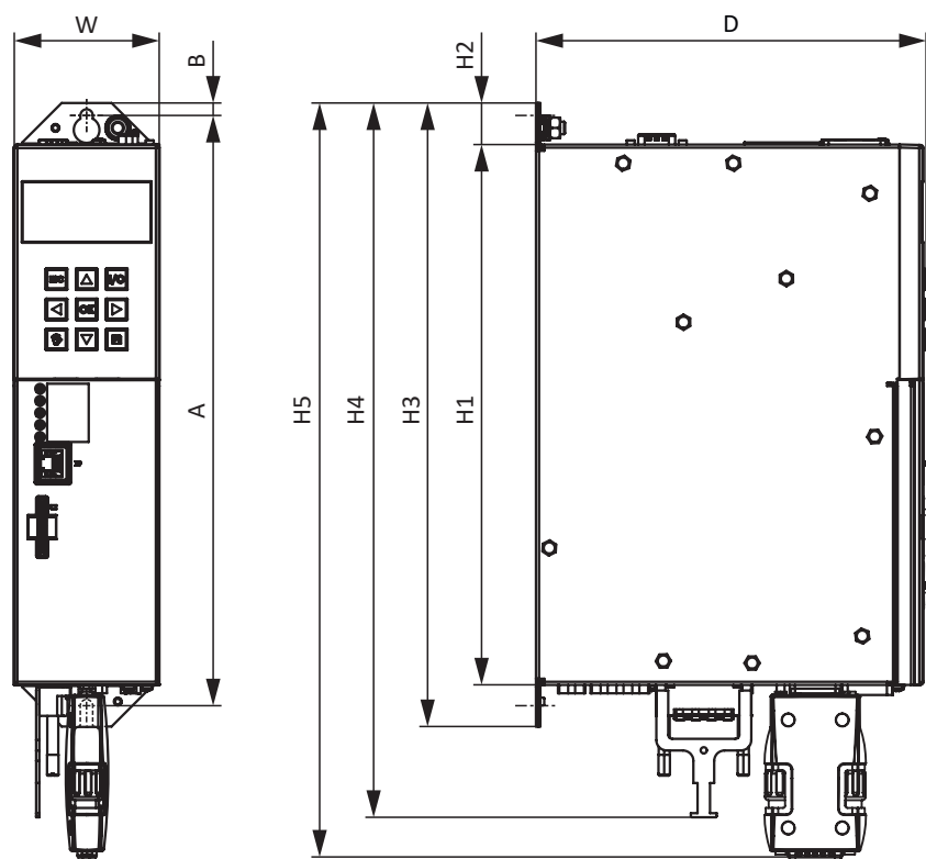
图 1: SB6 尺寸图
