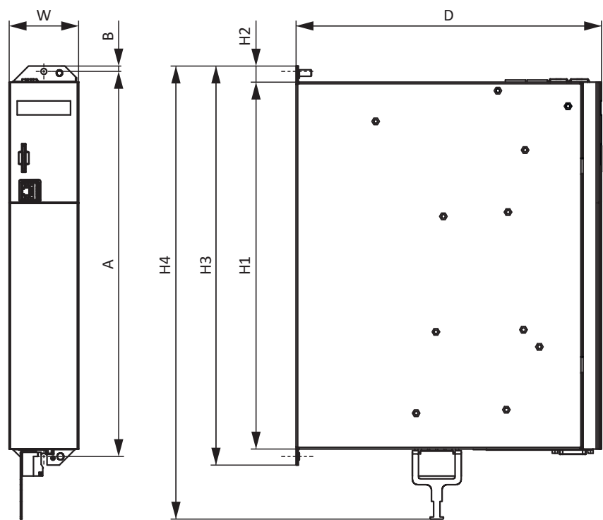
图 2: SC6 尺寸图
