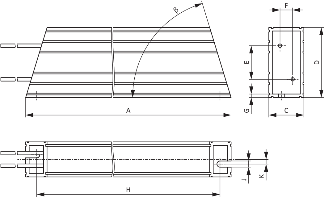
图 5: GVADU、GBADU 尺寸图
