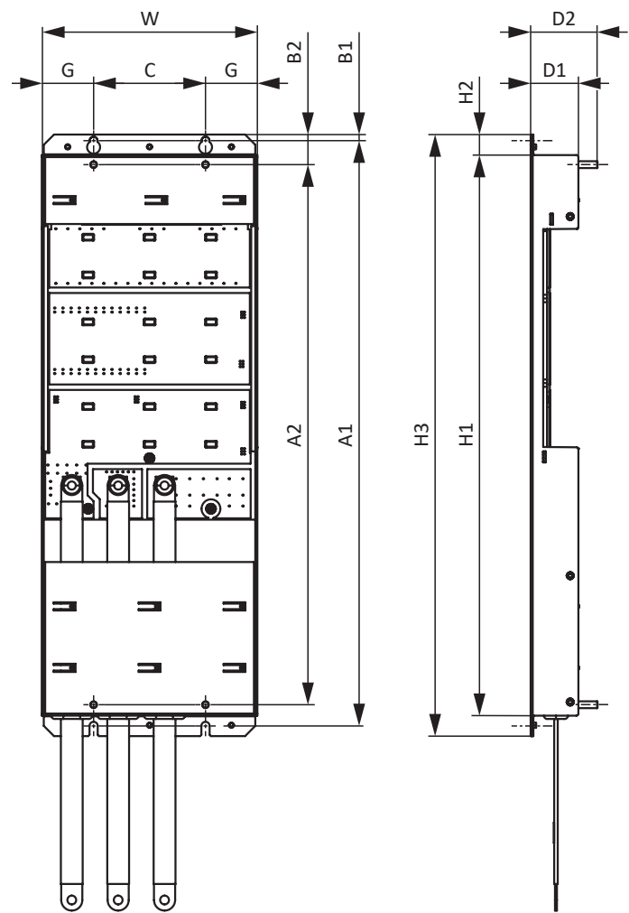
图 6: DL6B22 尺寸图
