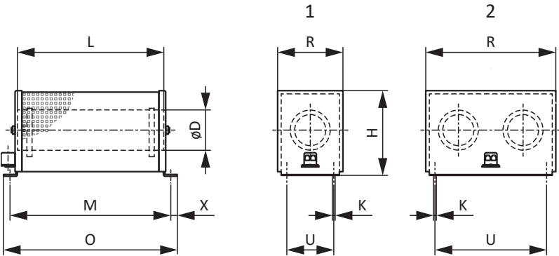
图 4: FZMU (1)、FZZMU (2) 尺寸图
