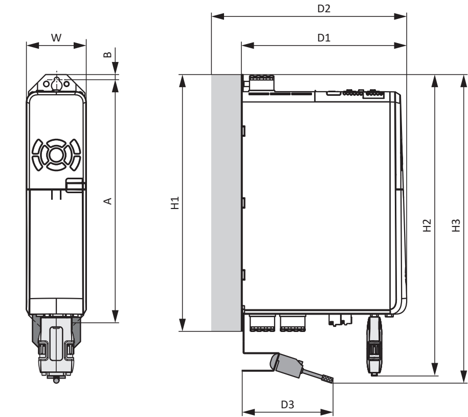
图 1: SD6 尺寸，规格 0 至 2
