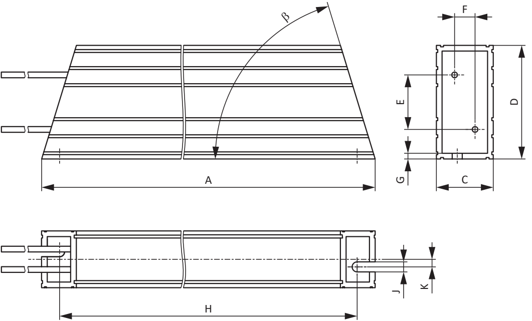
图 5: GVADU、GBADU 尺寸图
