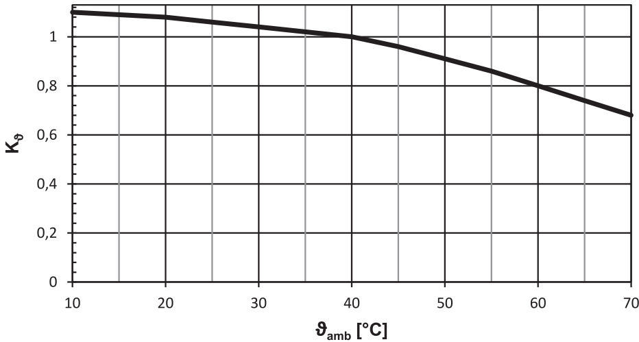
图 5: 取决于环境温度的降额
