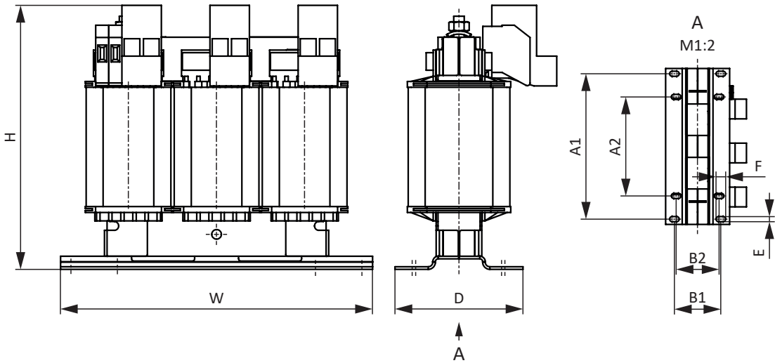
图 6: TEP 尺寸图
