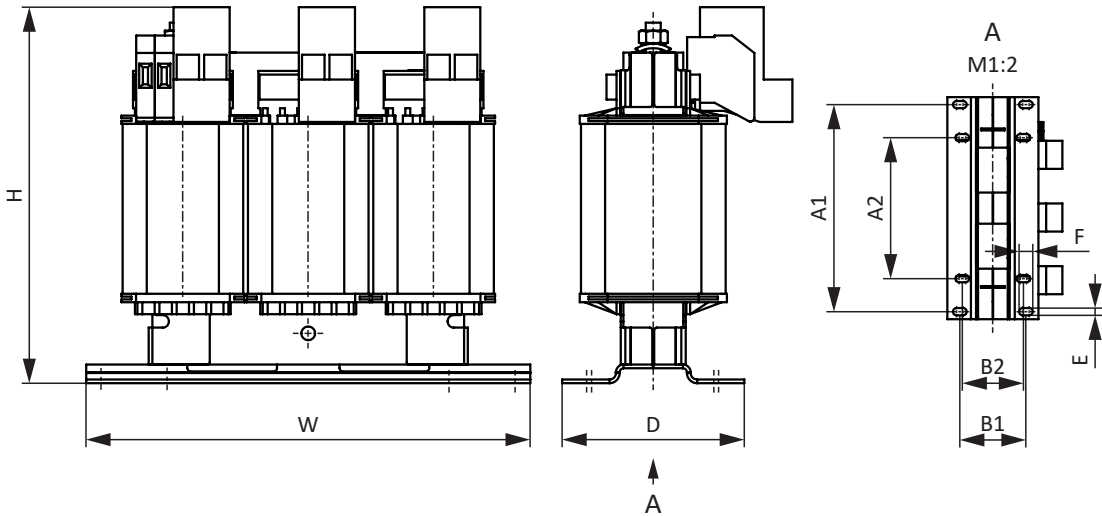
图 5: TEP 尺寸图
