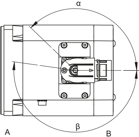
插头连接器的旋转范围 (EZ4 – EZ7 电机)
