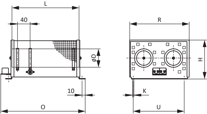
图 11: FZZMQU 尺寸图
