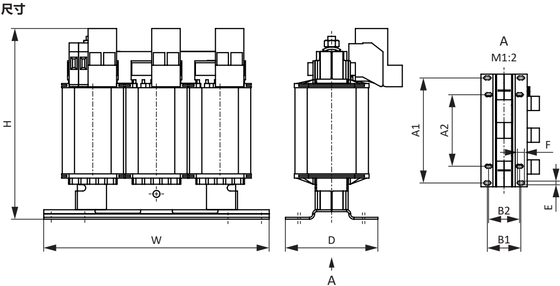
图 8: TEP 尺寸图
