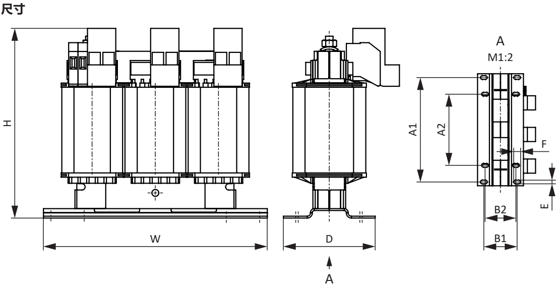
图 14: TEP 尺寸图
