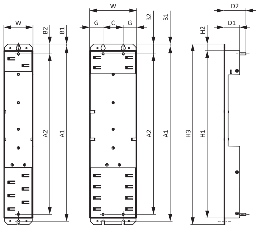
图 5: DL6B10 至 DL6B21 尺寸图
