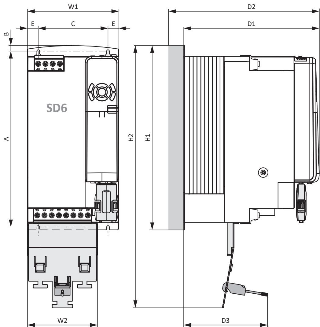
图 2: SD6 尺寸，规格 3
