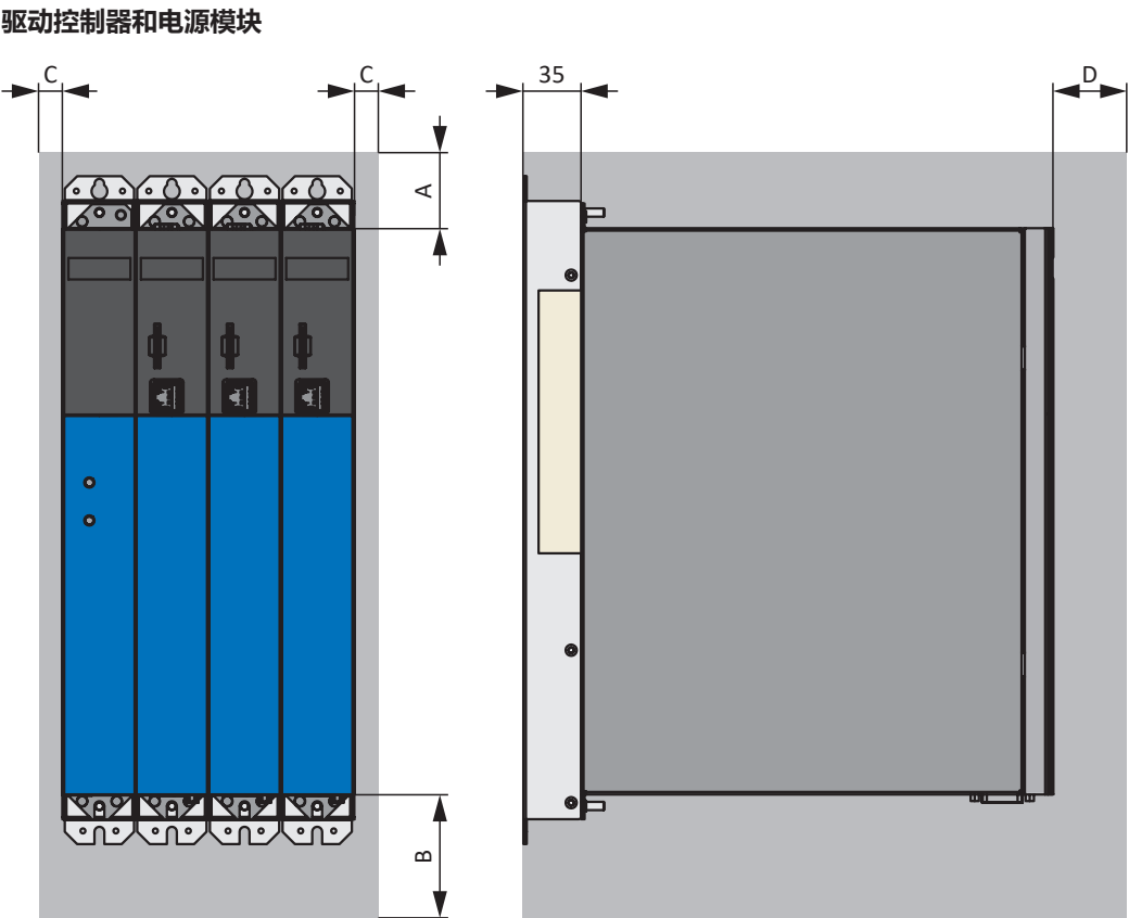
图 7: 驱动控制器与 PS6A24 或 PS6A34 电源模块组合的最小自由空间
