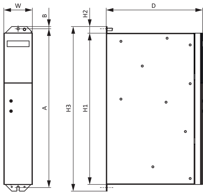
图 3: PS6A24、PS6A34 尺寸图
