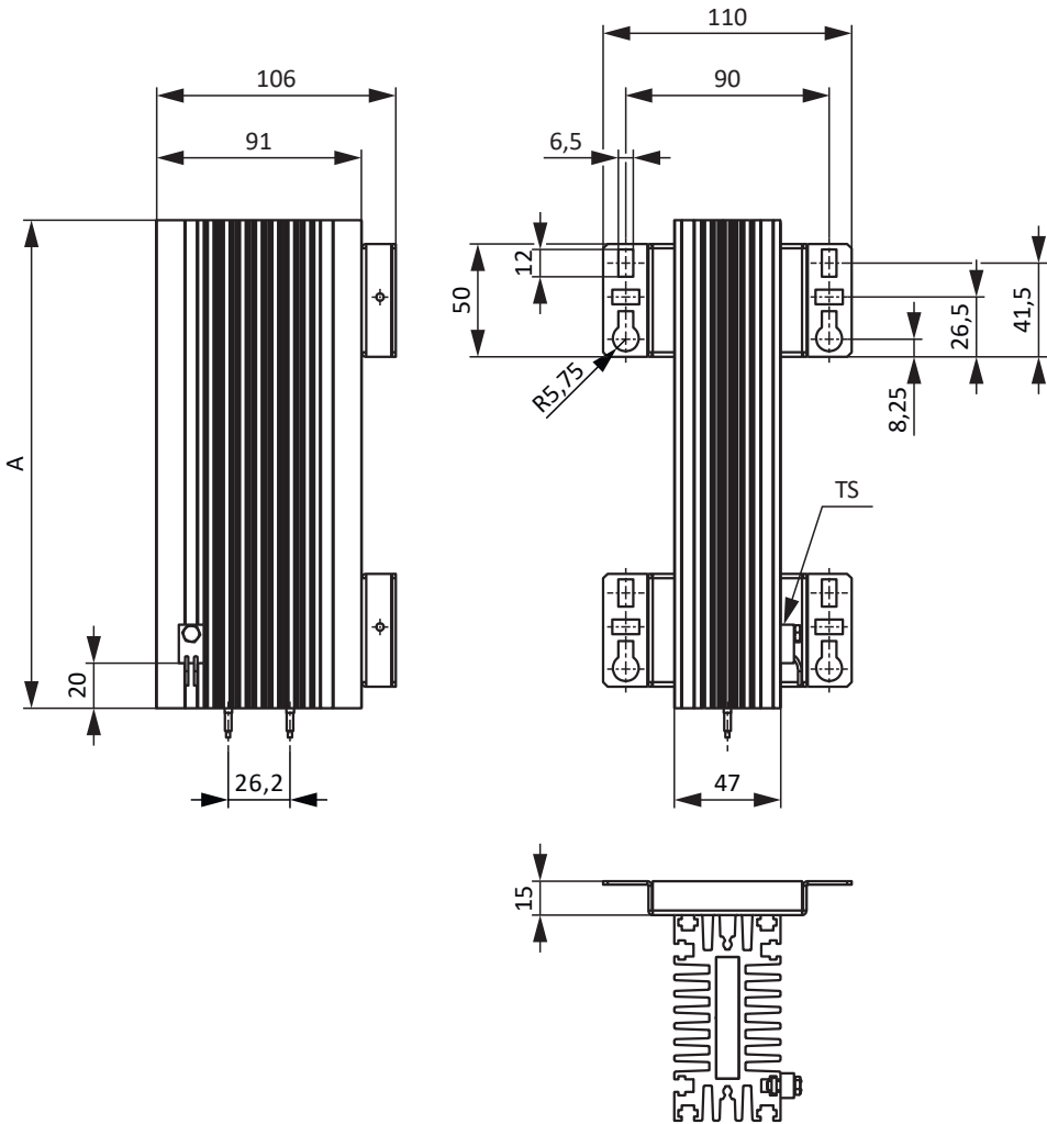
图 10: 带 MWS310L 的KWADQU 尺寸图
