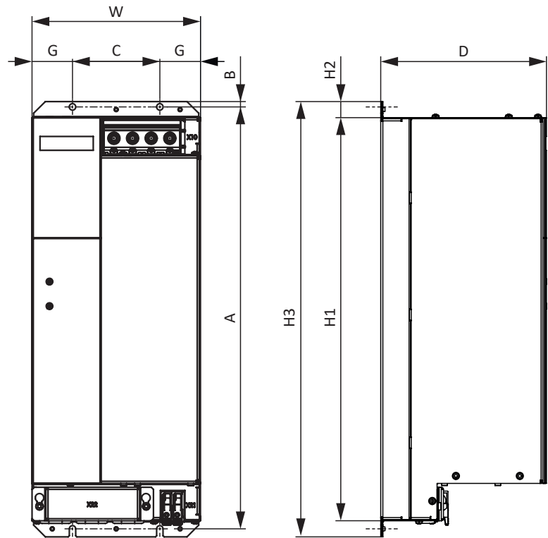
图 4: PS6A44 尺寸图
