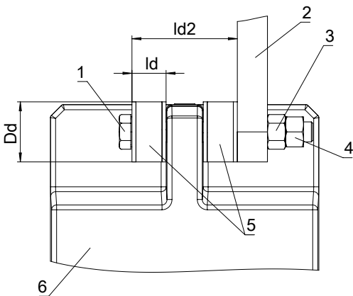
Fig. 5: Montage d'un support de couple sur le réducteur F (exemple)
