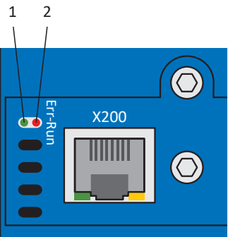
Abb. 6: Leuchtdioden für den EtherCAT-Zustand
