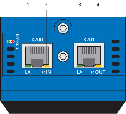
Abb. 7: Leuchtdioden für den Zustand der EtherCAT-Netzwerkverbindung
