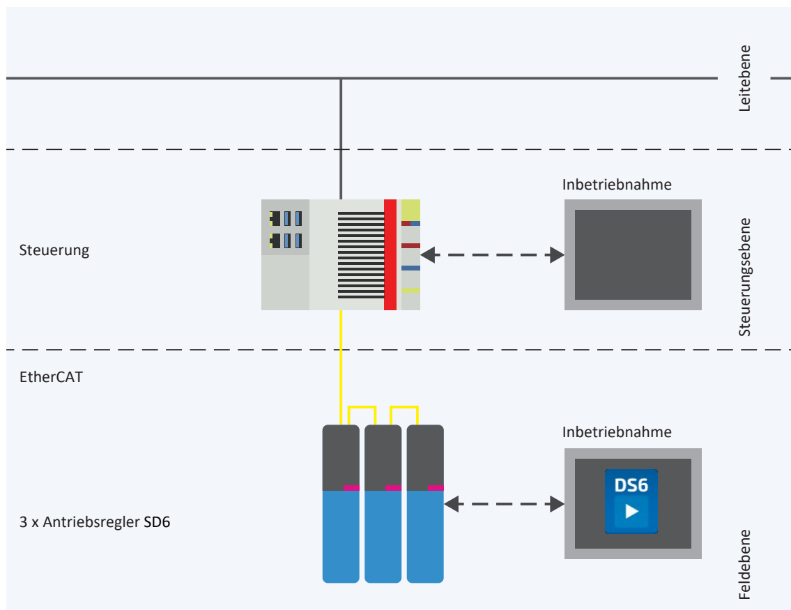
Abb. 1: EtherCAT: Netzwerkaufbau
