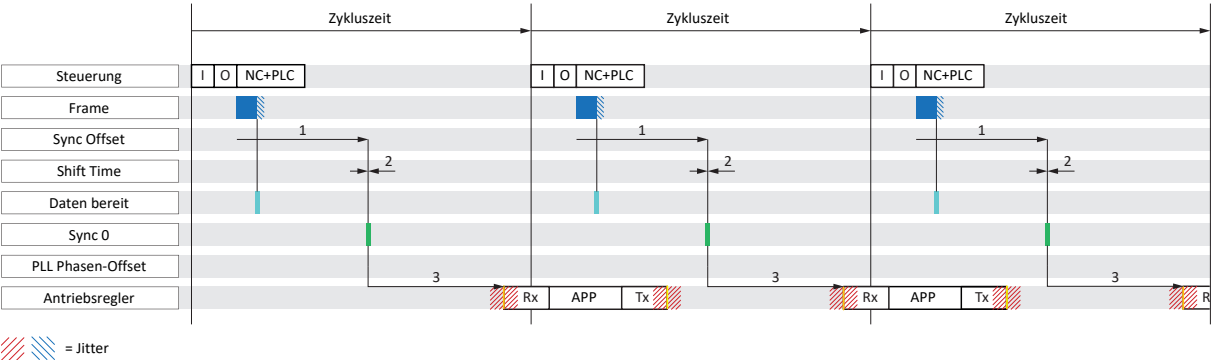
Abb. 15: CODESYS V3: DC-Sync – Einstellungen
