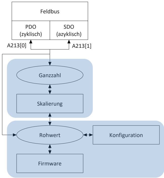
Abb. 16: Feldbusskalierung im Überblick
