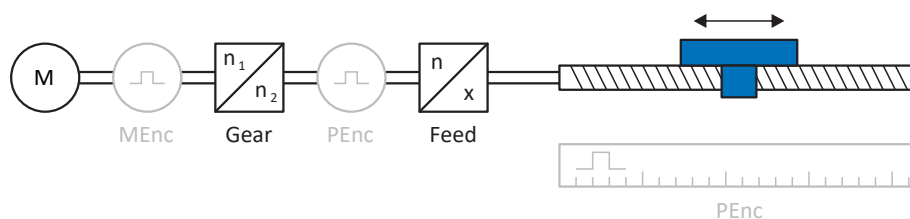
Fig. 9: Mouvement translatatoire limité : chariot porte-outils
