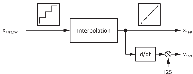
Fig. 26: Commande pilote interne générée par l'entraînement
