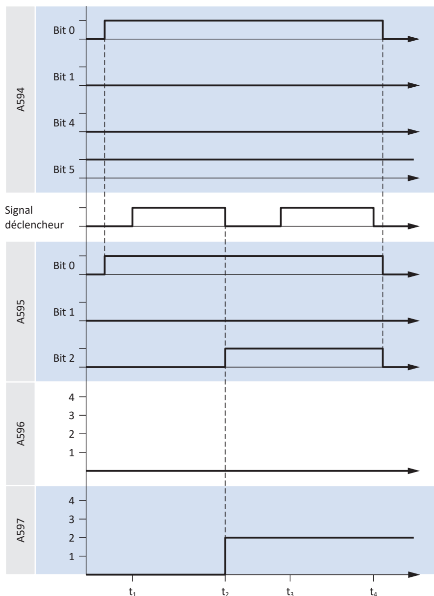
Fig. 31: Touch probe : exemple 2
