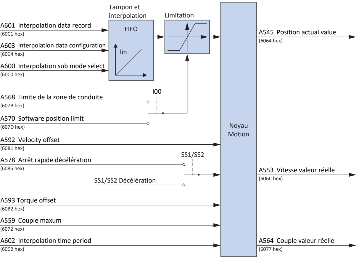
Fig. 13: Interpolated position mode : signaux d'entrée et de sortie
