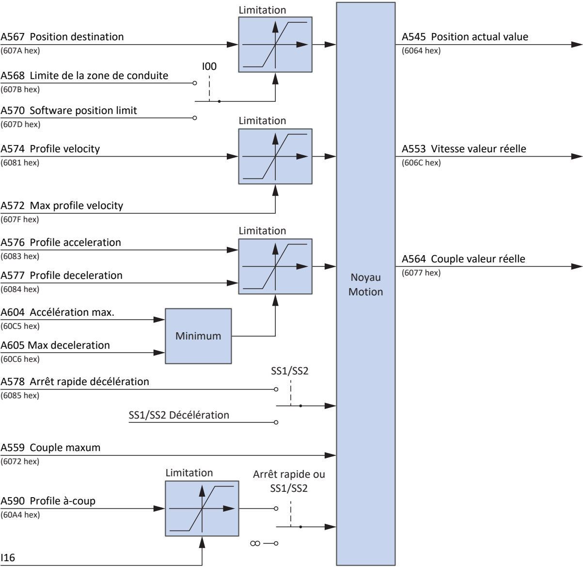
Fig. 17: Profile position mode : signaux d'entrée et de sortie
