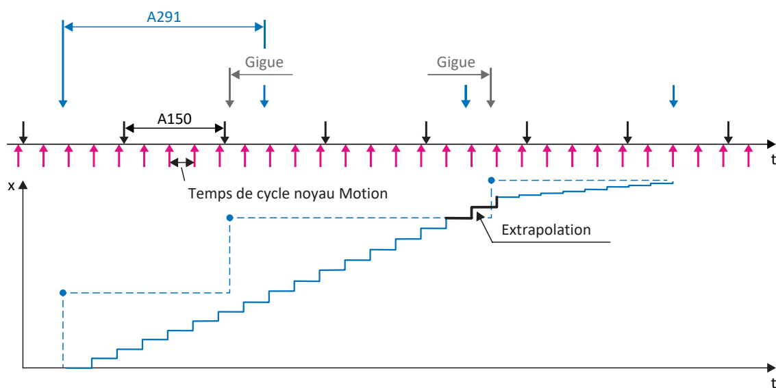
Fig. 29: Interpolation : gigue temporelle de la commande
