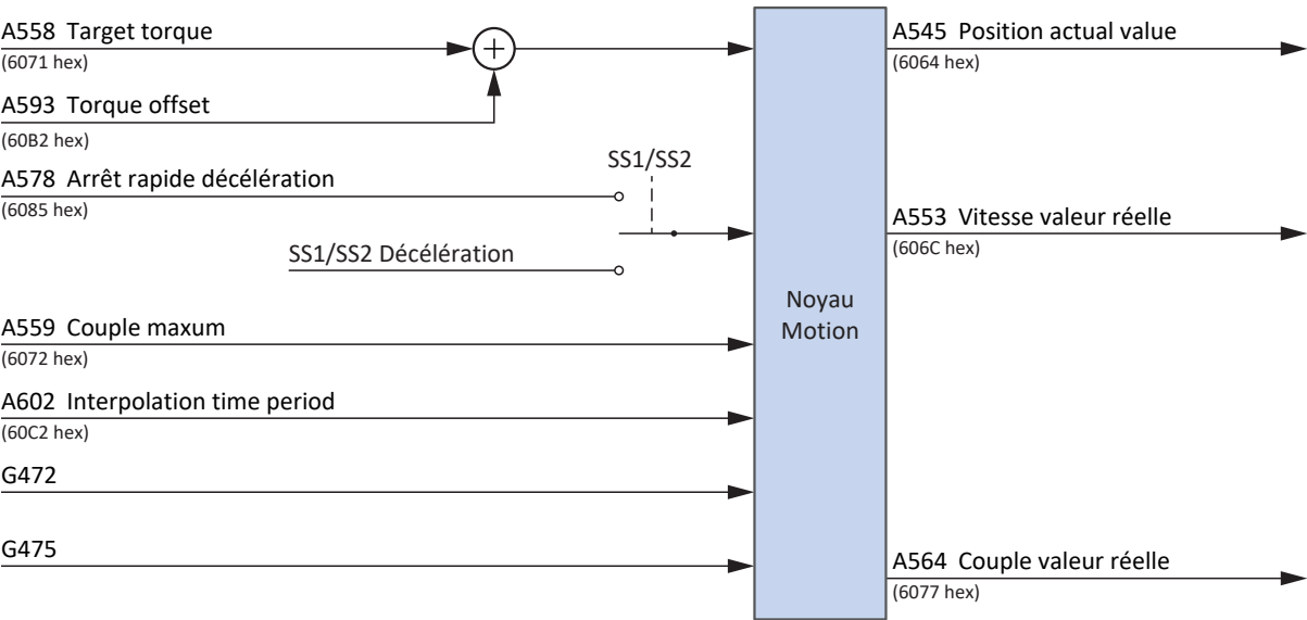
Fig. 16: Cyclic synchronous torque mode : signaux d'entrée et de sortie
