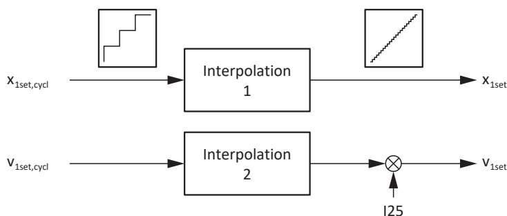
Fig. 25: Commande pilote externe générée par la commande
