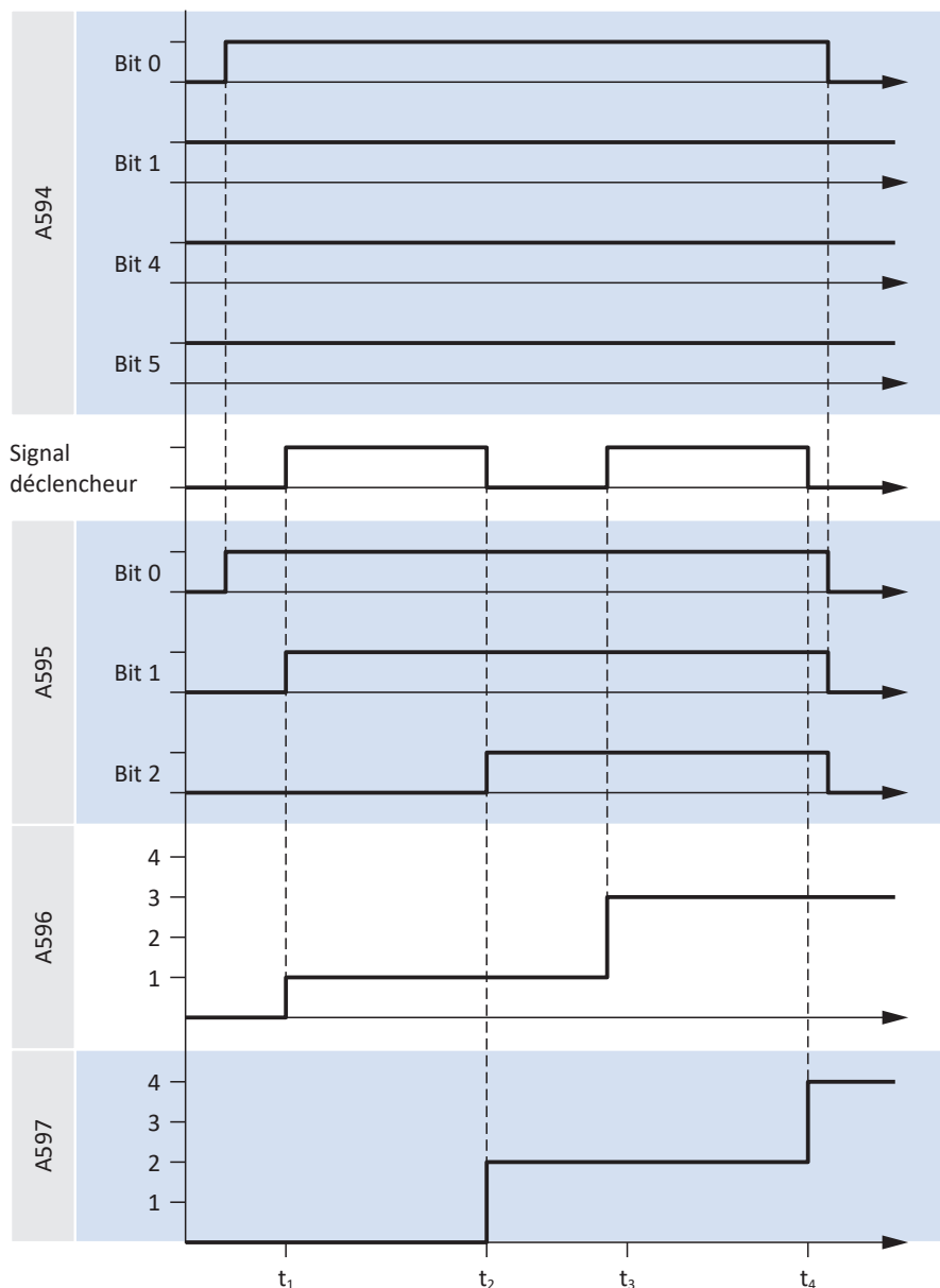
Fig. 30: Touch probe : exemple 1
