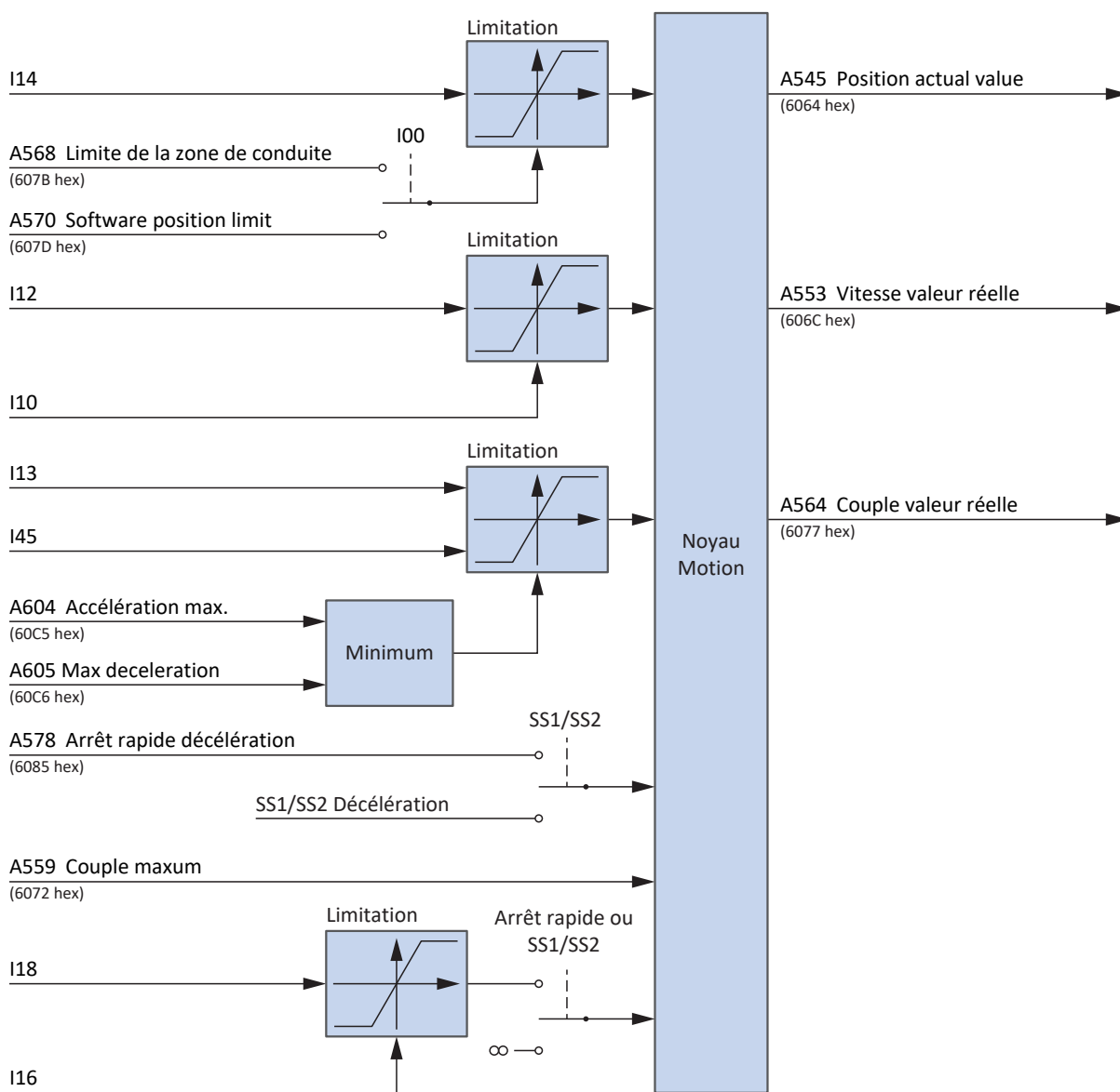
Fig. 22: Pas à pas : signaux d'entrée et de sortie
