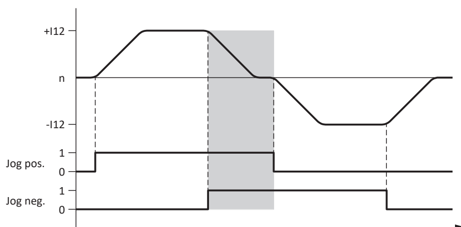
Fig. 24: Pas à pas – Réaction aux signaux contradictoires
