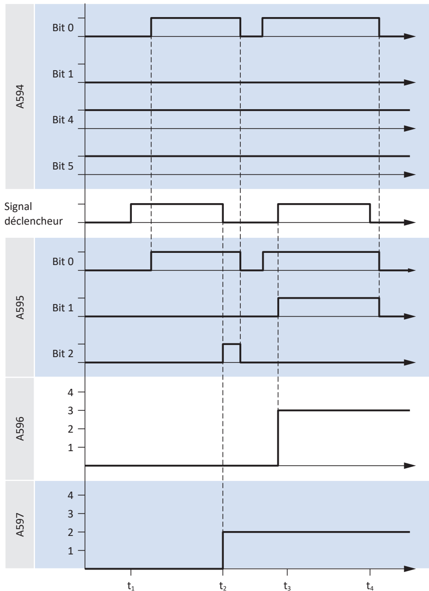
Fig. 32: Touch probe : exemple 3
