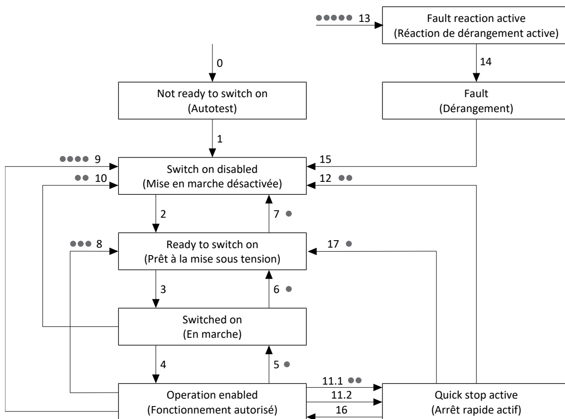
Fig. 12: Machine d'état CiA 402 : états de l'appareil et changement d'état
