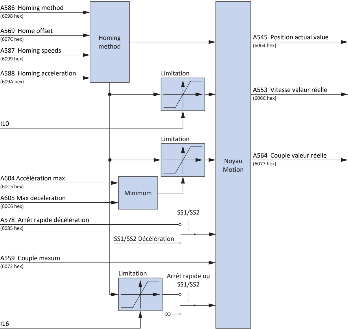
Fig. 21: Homing mode : signaux d'entrée et de sortie
