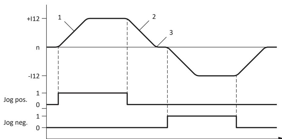
Fig. 23: Pas à pas – Accélération et freinage
