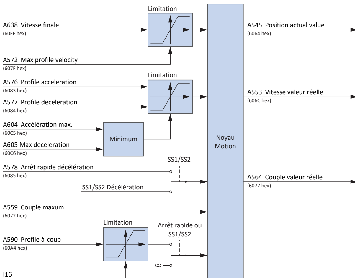
Fig. 19: Profile velocity mode : signaux d'entrée et de sortie
