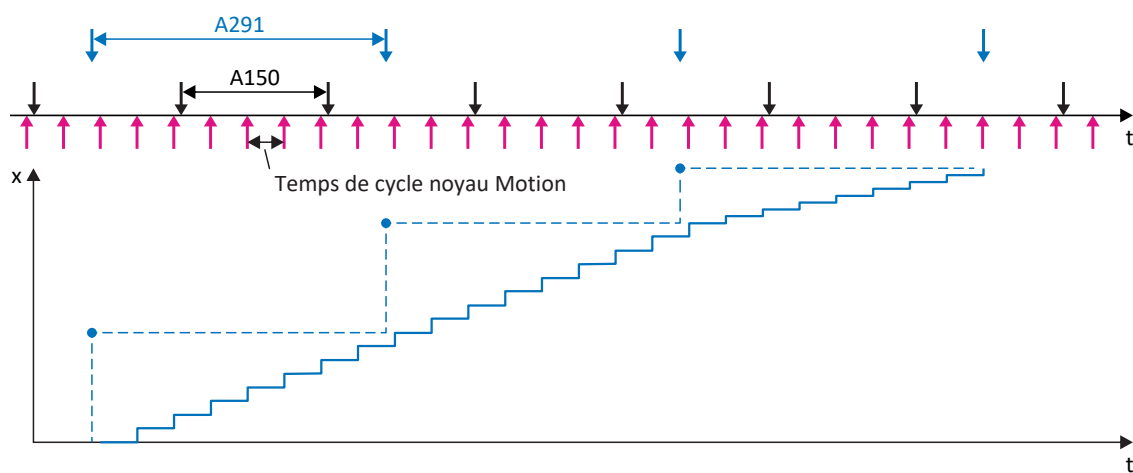
Fig. 28: Interpolation : comportement temporel idéal, pas de gigue
