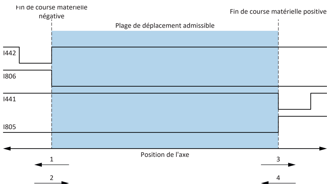
Fig. 11: Fins de course matérielles : mémoire des fins de course
