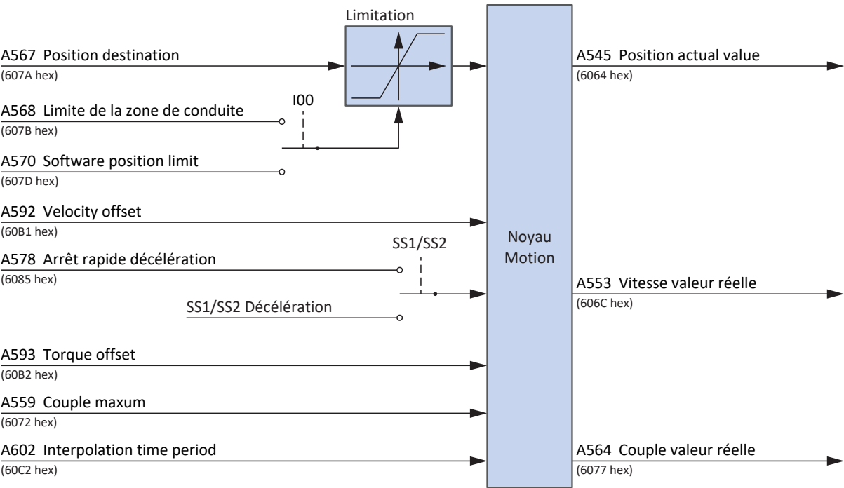
Fig. 14: Cyclic synchronous position mode : signaux d'entrée et de sortie
