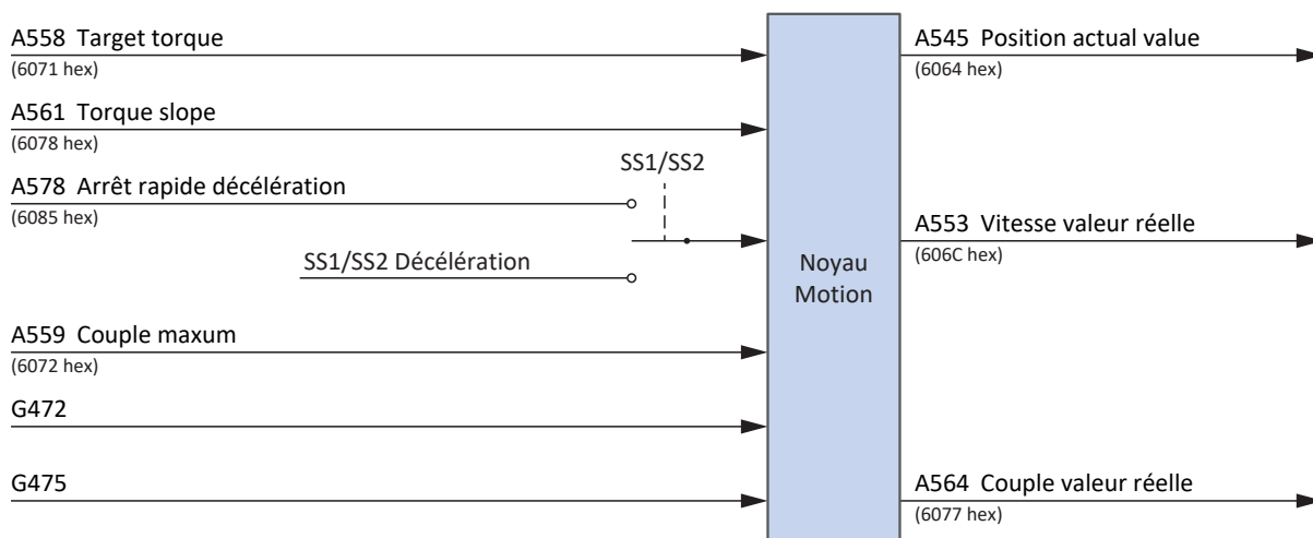
Fig. 20: Profile torque mode : signaux d'entrée et de sortie
