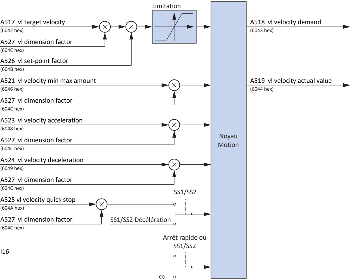
Fig. 18: Velocity mode : signaux d'entrée et de sortie
