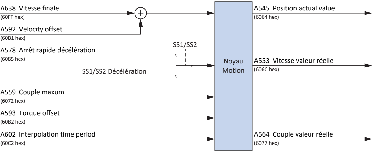
Fig. 15: Cyclic synchronous velocity mode : signaux d'entrée et de sortie
