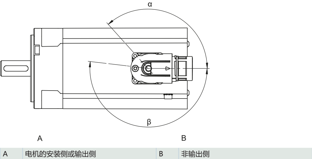
插头连接器的旋转范围（EZ2 – EZ3 电机）
