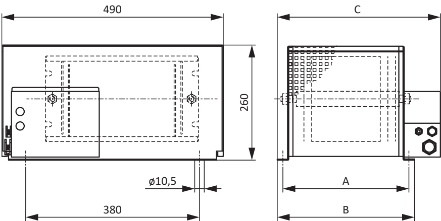
图 6: FGFKU 尺寸图
