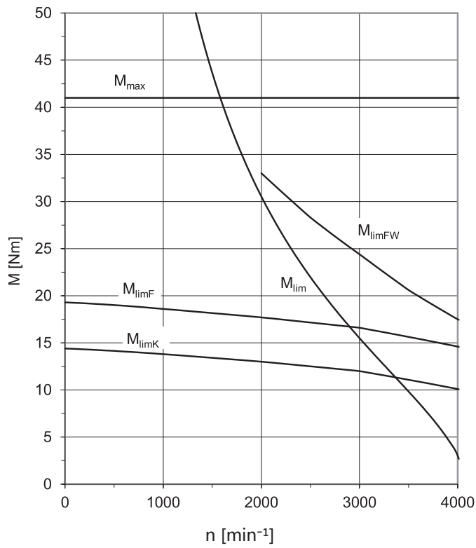
EZ702 ( n_N=3000 \text{ min}^{-1} )
