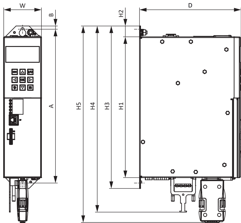
图 1: SB6 尺寸图
