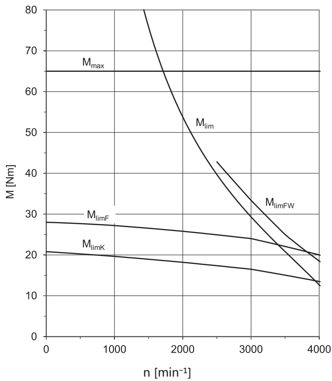
EZ703 ( n_N=3000 \text{ min}^{-1} )
