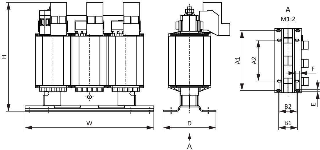
图 14: TEP 尺寸图
