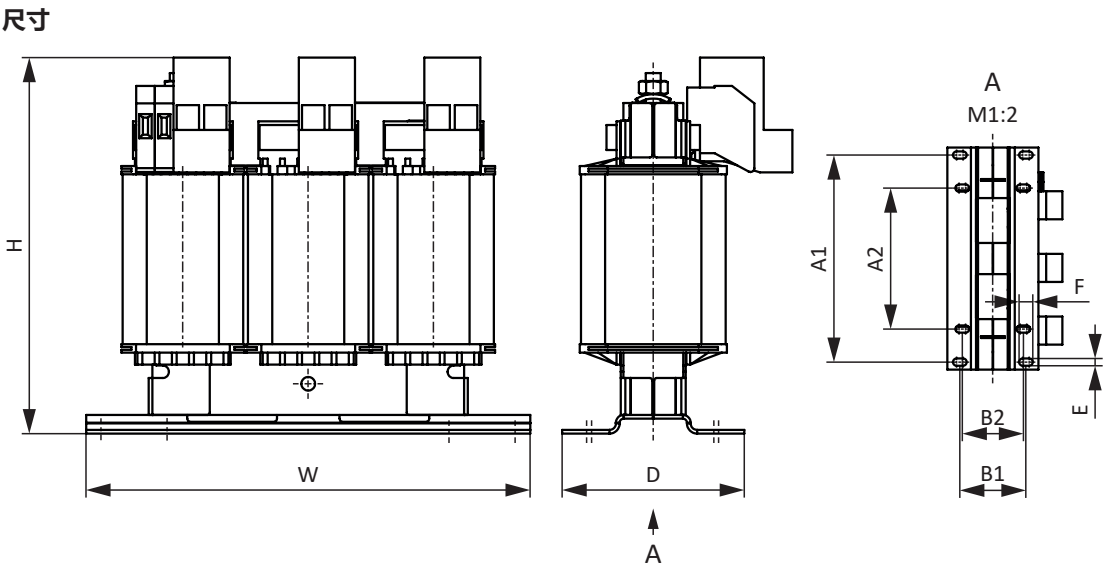
图 6: TEP 尺寸图
