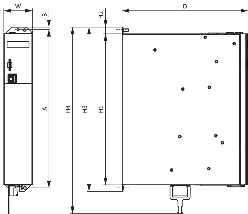
图 2: SC6 尺寸图
