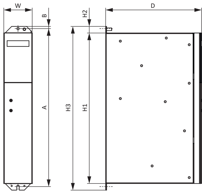
图 3: PS6A24、 PS6A34 尺寸图
