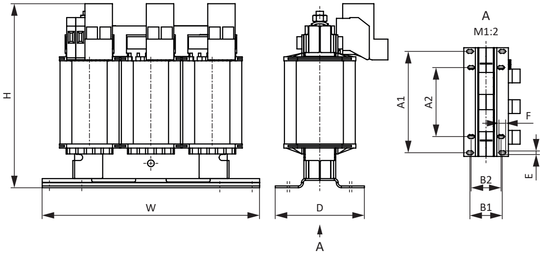
图 8: TEP 尺寸图
