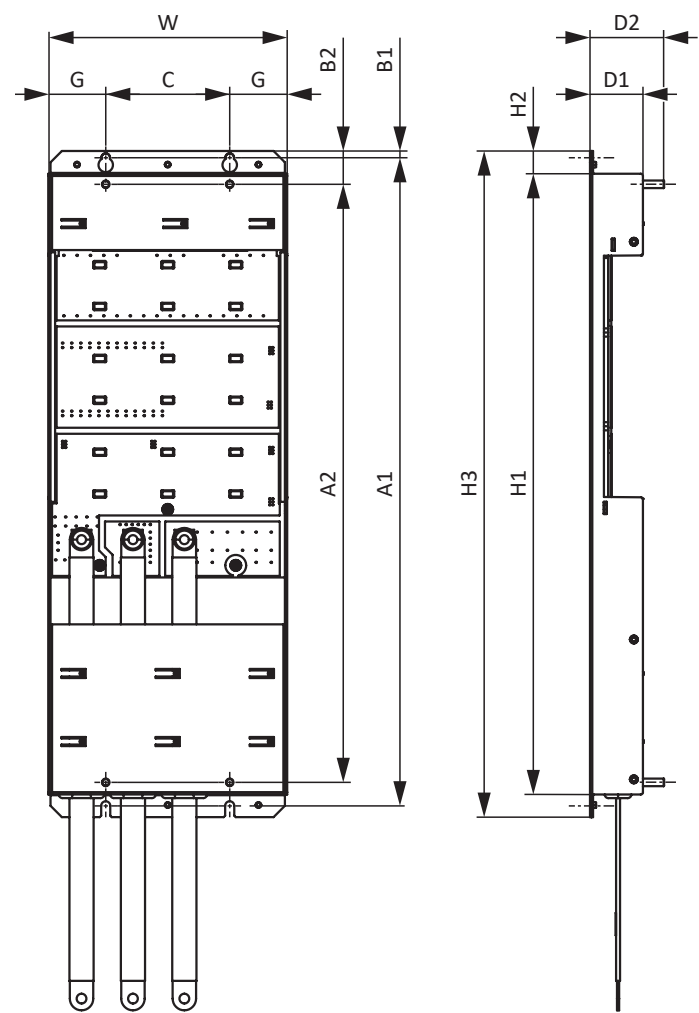
图 6: DL6B22 尺寸图
