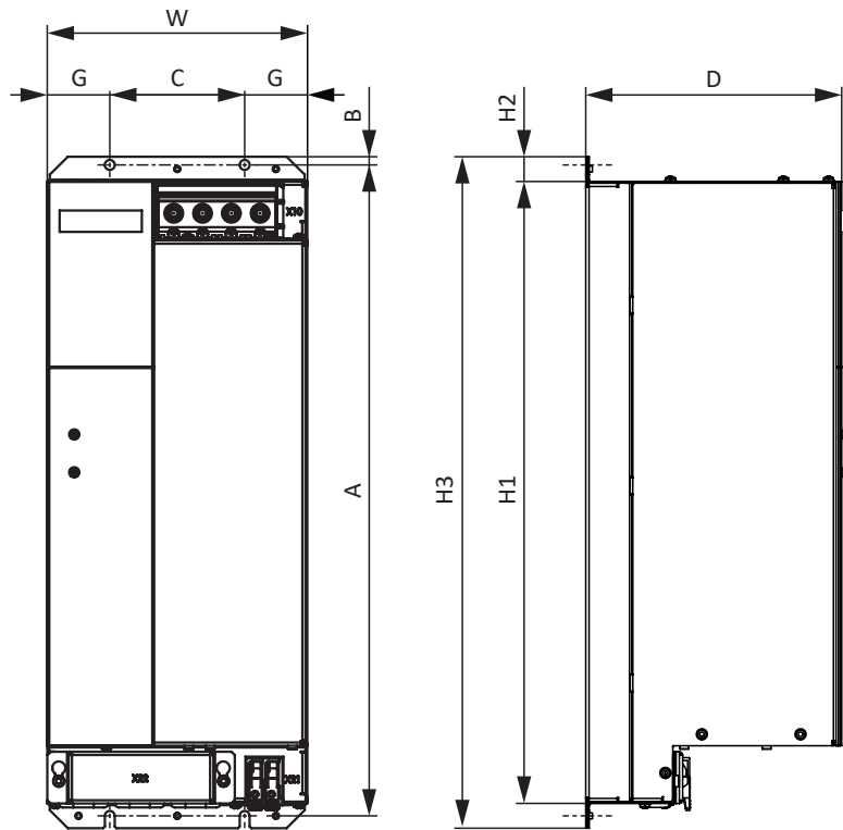
图 4: PS6A44 尺寸图
