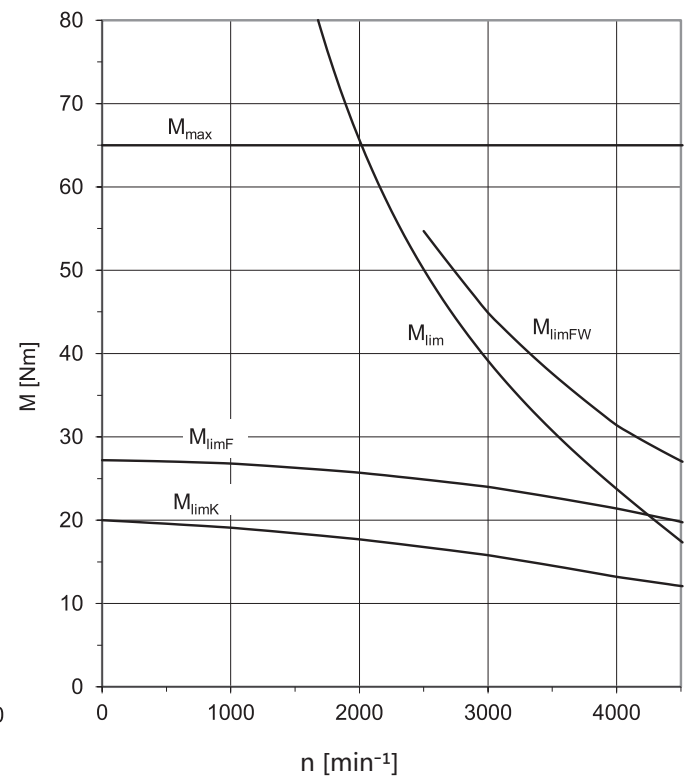
EZ703 ( n_N=4500 \text{ min}^{-1} )
