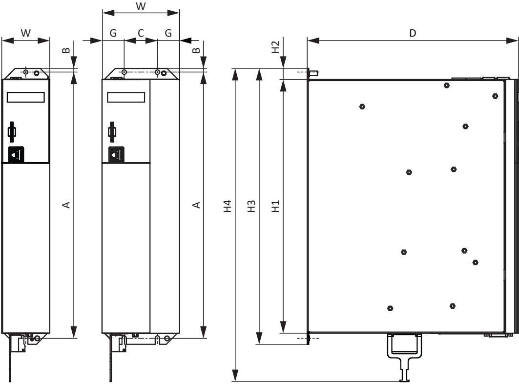
图 2: SI6 尺寸图
