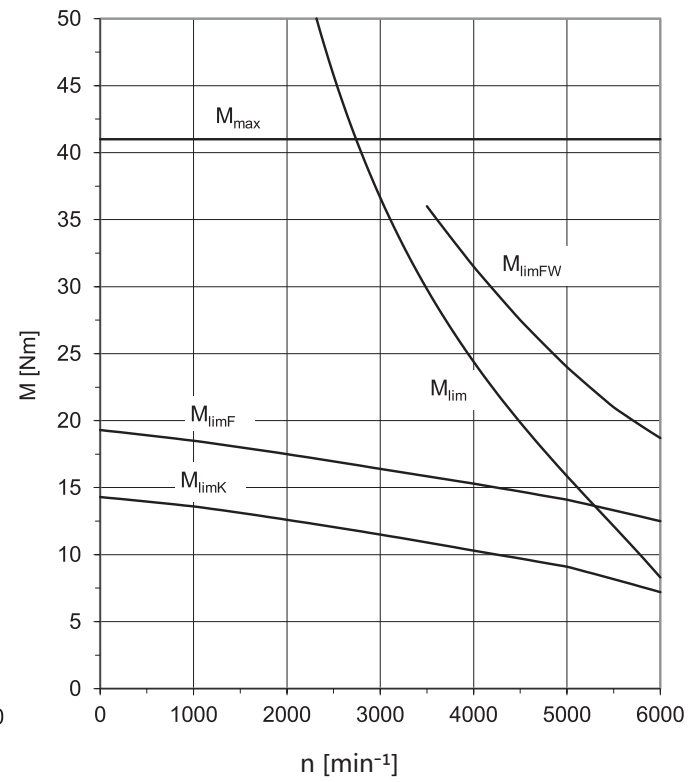
EZ702 ( n_N=6000 \text{ min}^{-1} )
