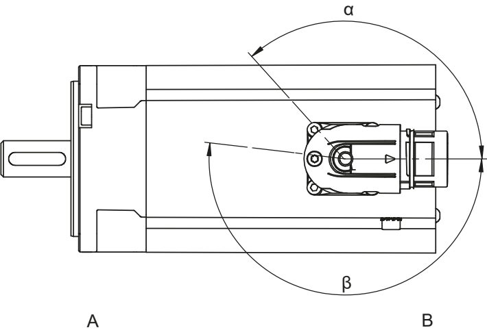
插头连接器的旋转范围（EZ2 – EZ3 电机）
