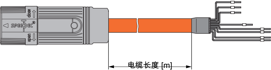
图 2: 预制电源线的长度定义 – SB6、SC6、SI6
