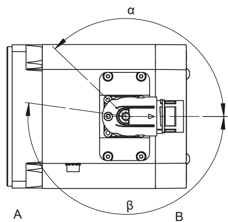
插头连接器的旋转范围 (EZ4 – EZ7 电机)
