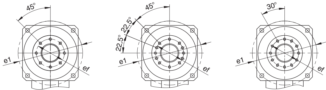
减速器尺寸
