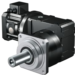
加装同步伺服电机的带有抱闸的电机适配器 MB
