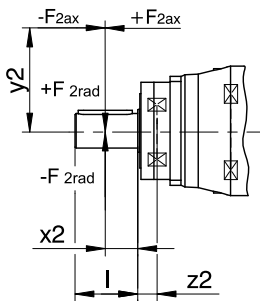
图 5: 受力点
