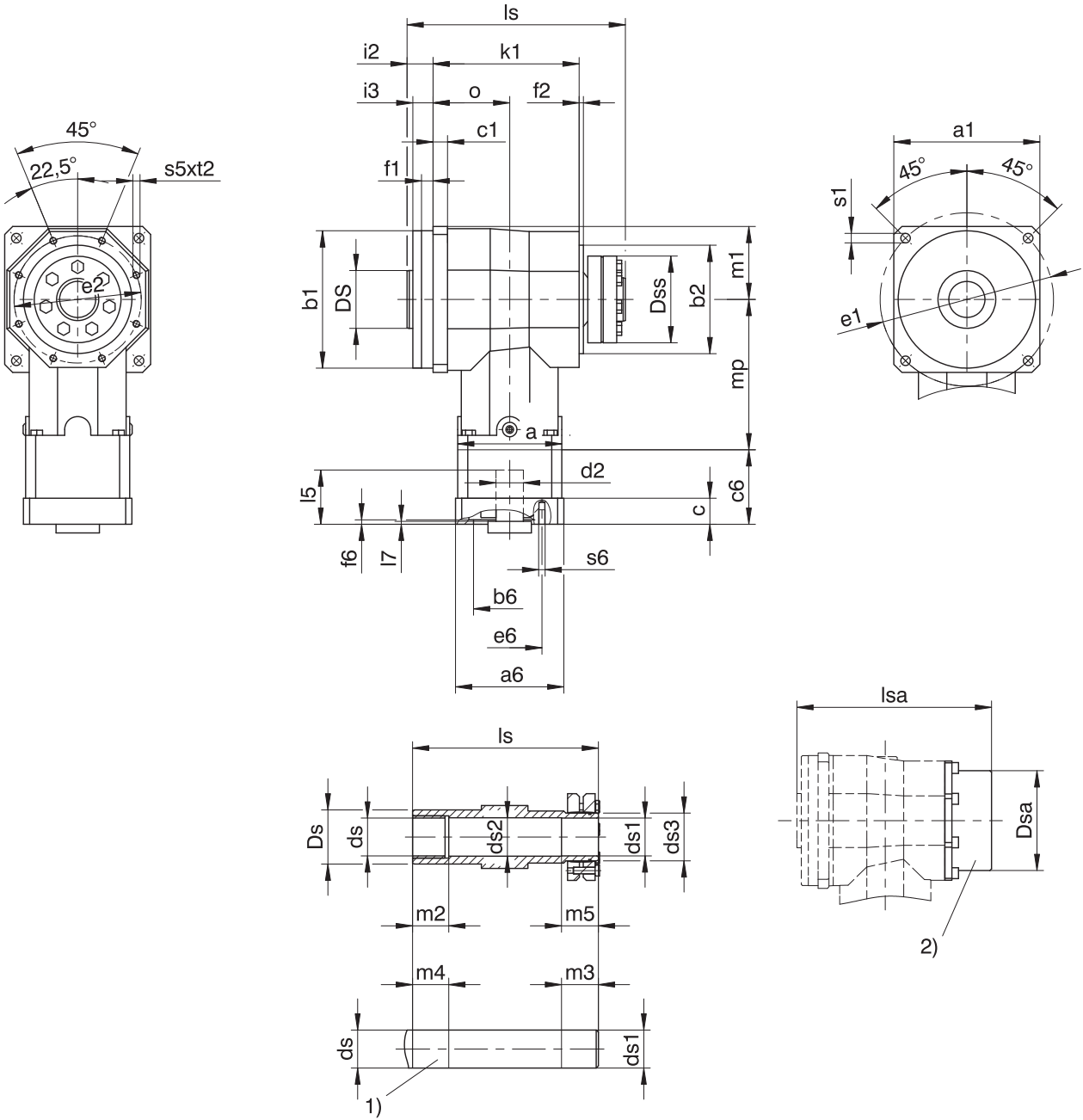
1) 机器轴：不得低于尺寸 ls。 2) 保护罩（选配）
