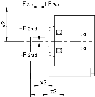
图 3: 受力点
