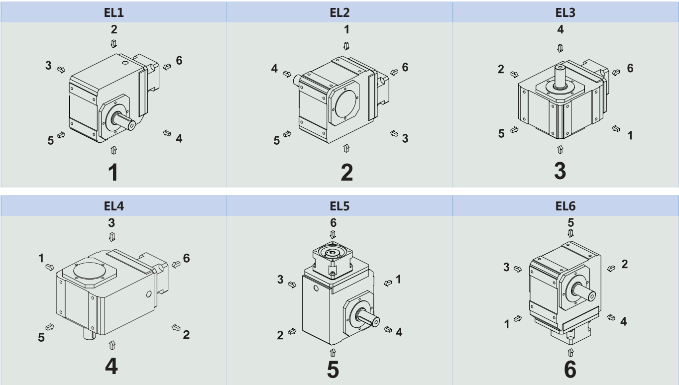
减速器规格 K5 – K10 安装位置
