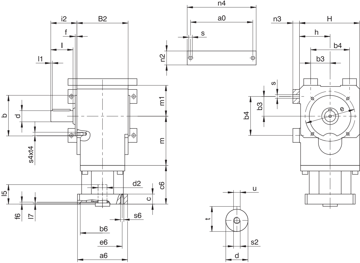
减速器尺寸
