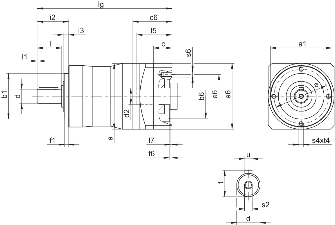
减速器尺寸
