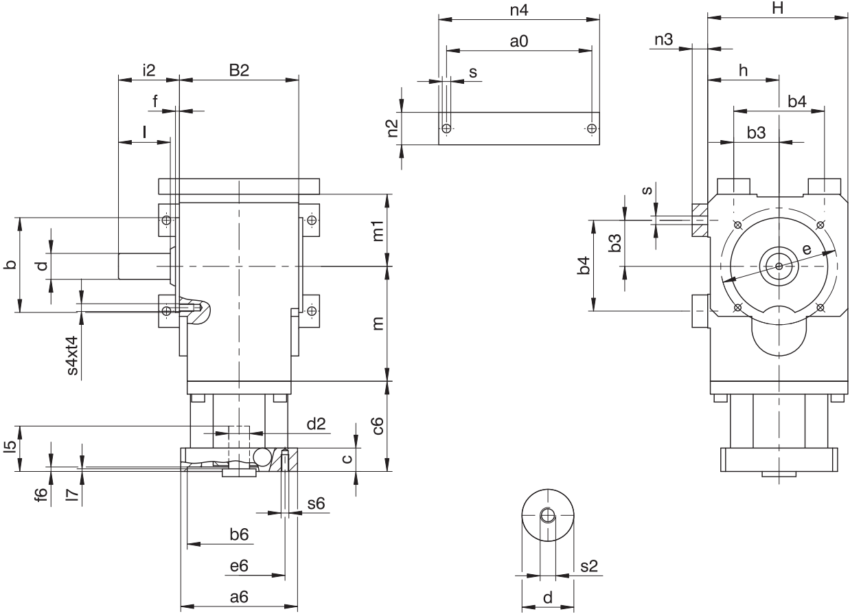
减速器尺寸
