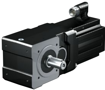
精益电机 LM
