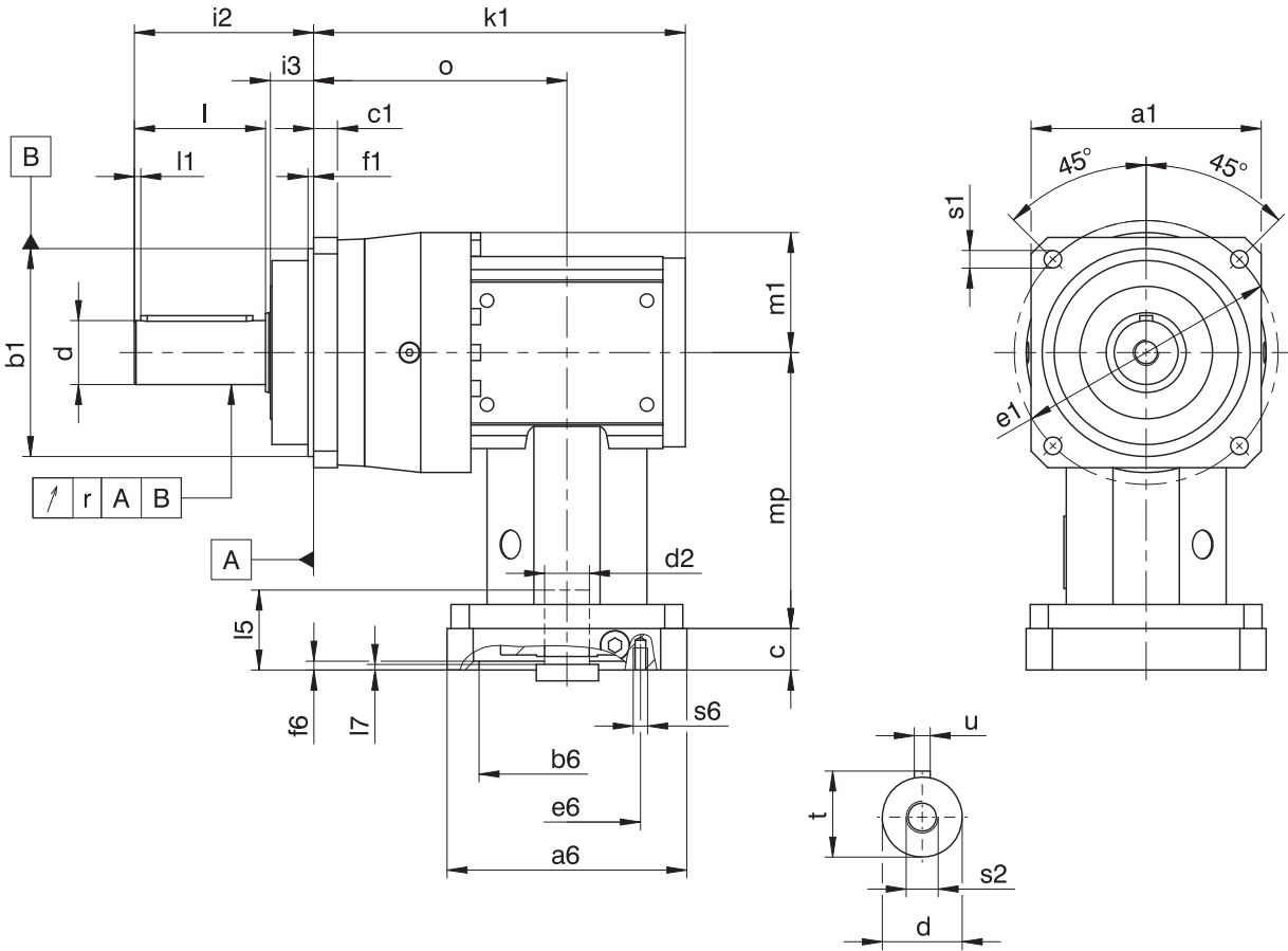
减速器尺寸
