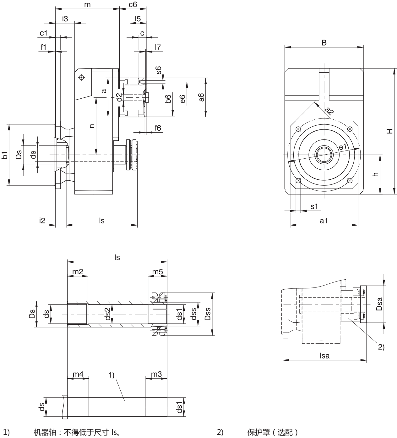
减速器尺寸
