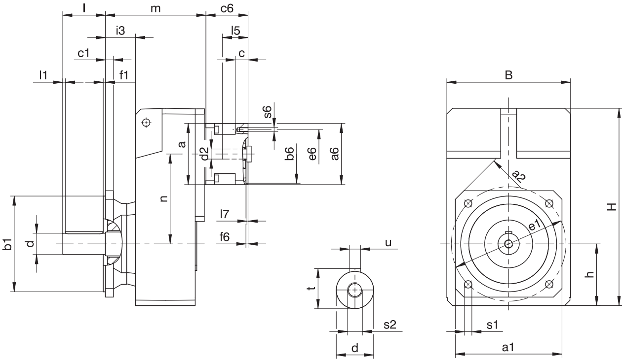
减速器尺寸
