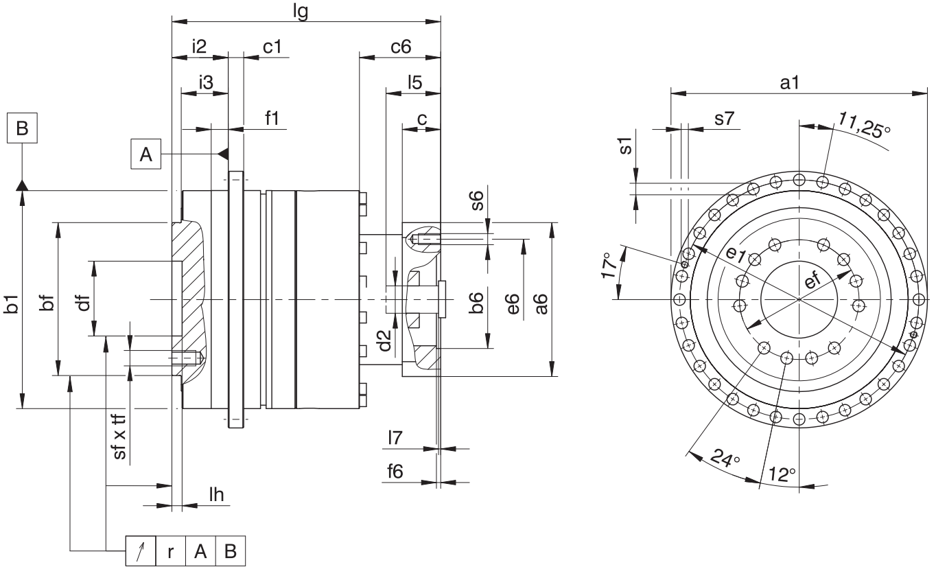
减速器尺寸
