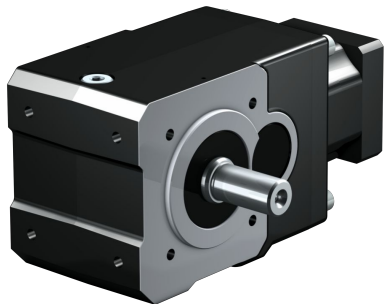
加装同步伺服电机的电机适配器 MQ
