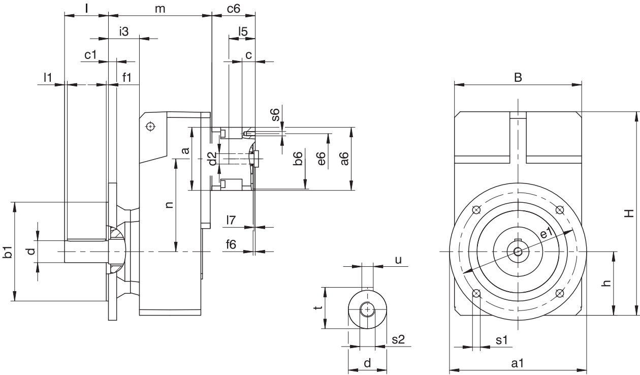
减速器尺寸
