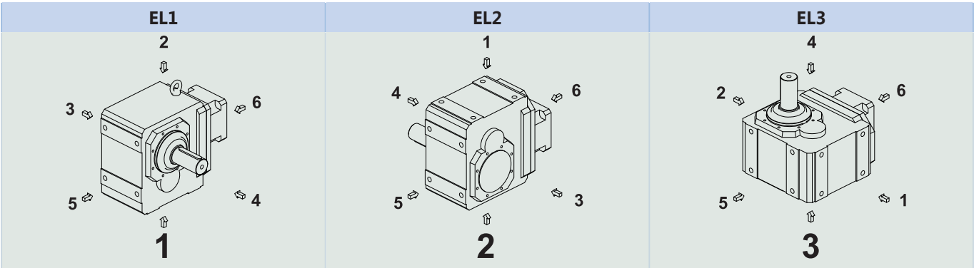
减速器规格 K5 – K10 安装位置
