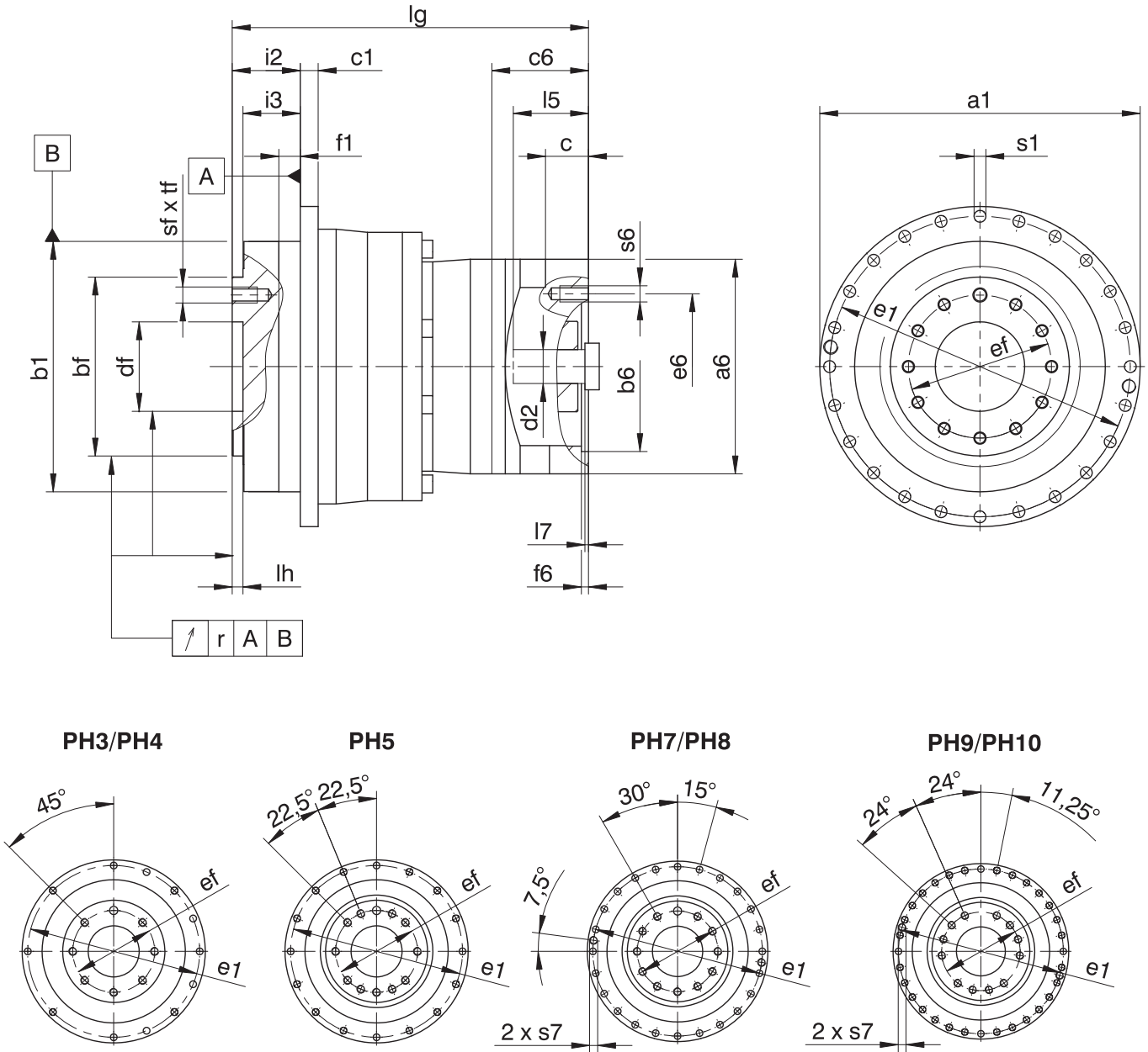
减速器尺寸
