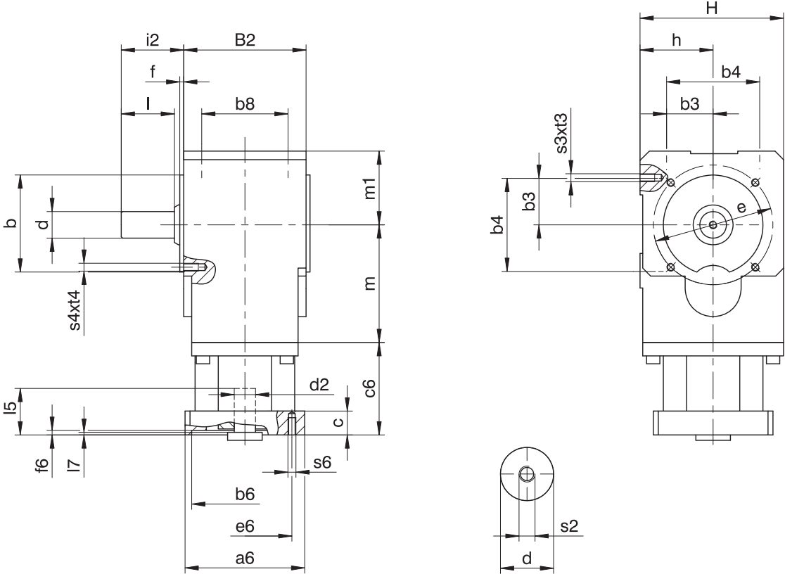
减速器尺寸
