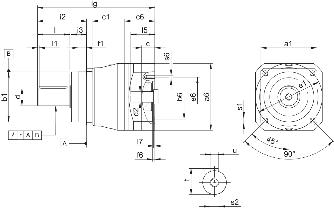
减速机尺寸
