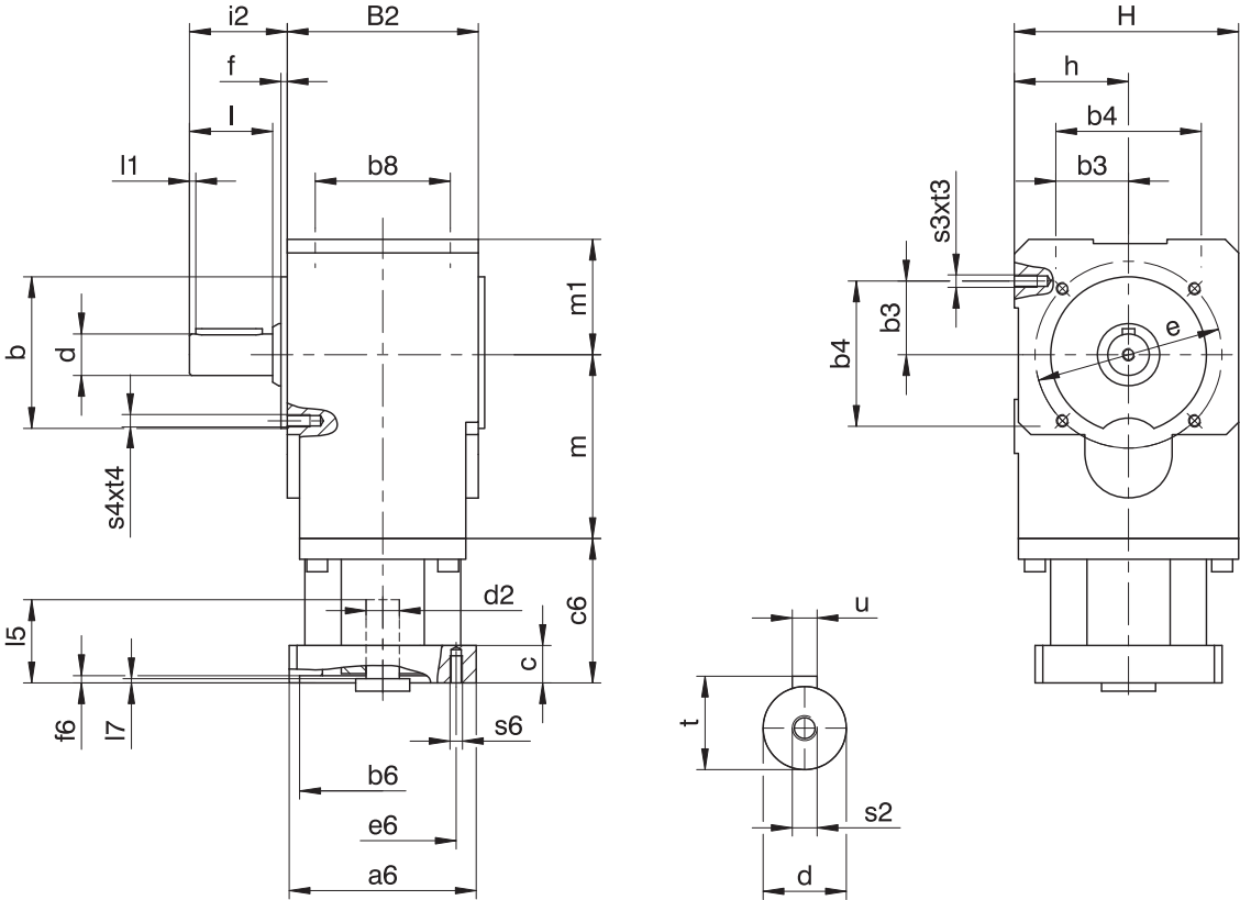
减速器尺寸
