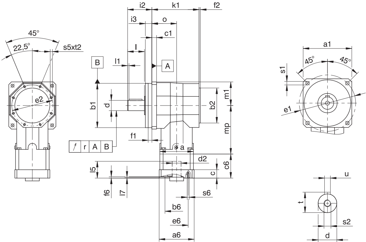
减速器尺寸
