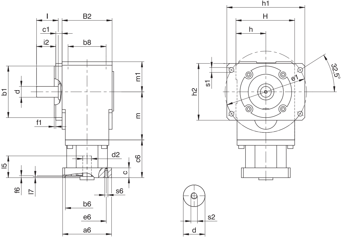
减速器尺寸
