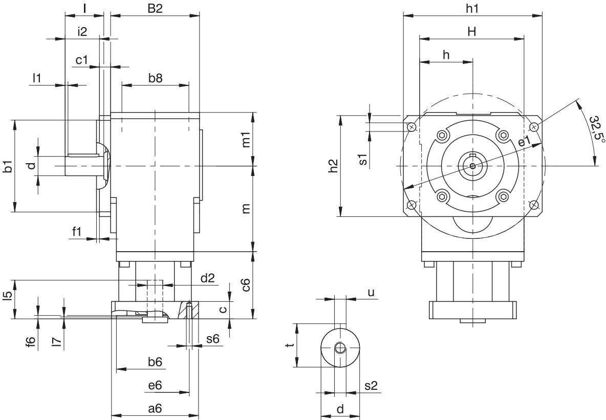
减速器尺寸
