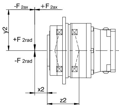
图 3: 受力点
