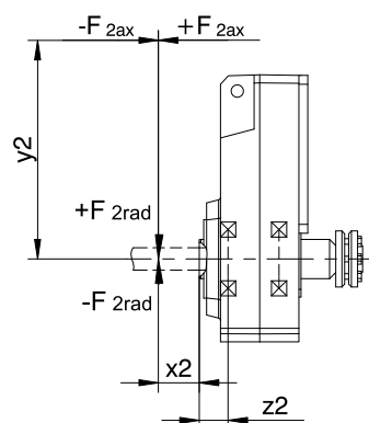
图 4: 空心轴受力点
