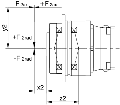
图 2: 受力点
