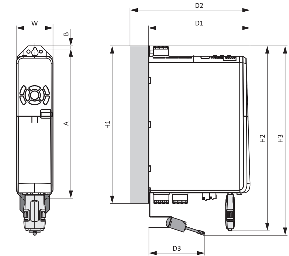
Abb. 1: Maßzeichnung SD6, Baugrößen 0 bis 2
