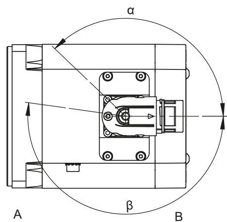
Verdrehbereiche der Steckverbinder (Motoren EZ4 – EZ7)
