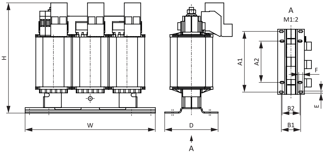
Abb. 5: Maßzeichnung TEP
