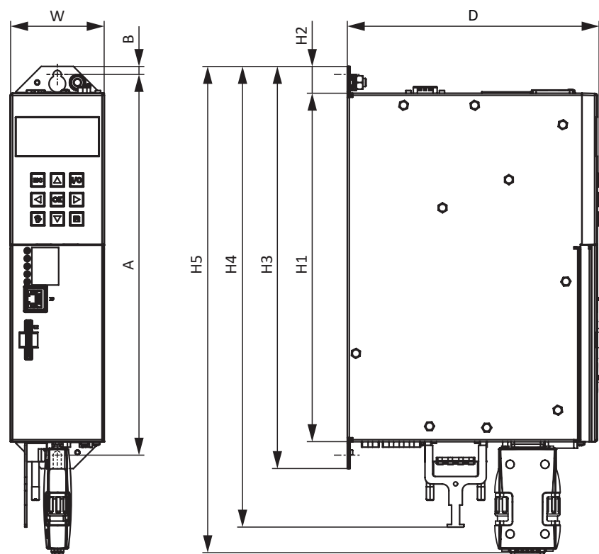
Abb. 1: Maßzeichnung SB6
