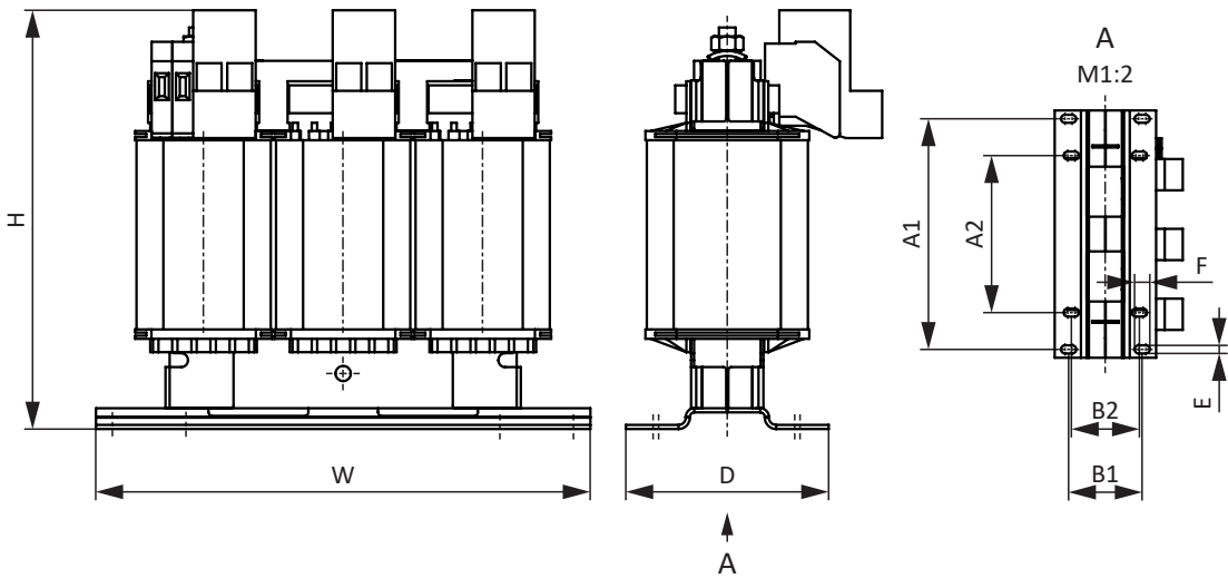
Abb. 14: Maßzeichnung TEP
