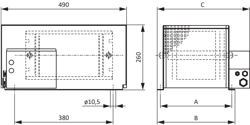
Abb. 6: Maßzeichnung FGFKU
