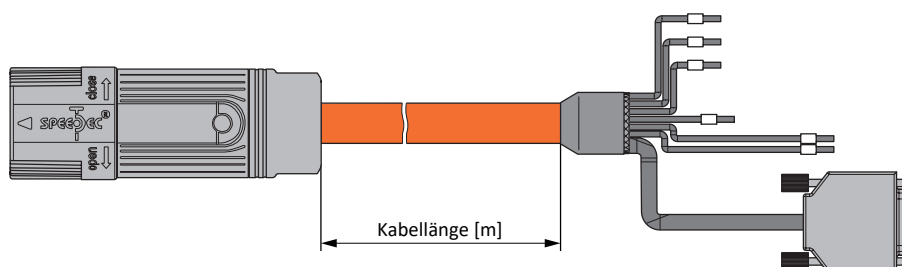
Abb. 4: Längendefinition für konfektionierte Hybridkabel
