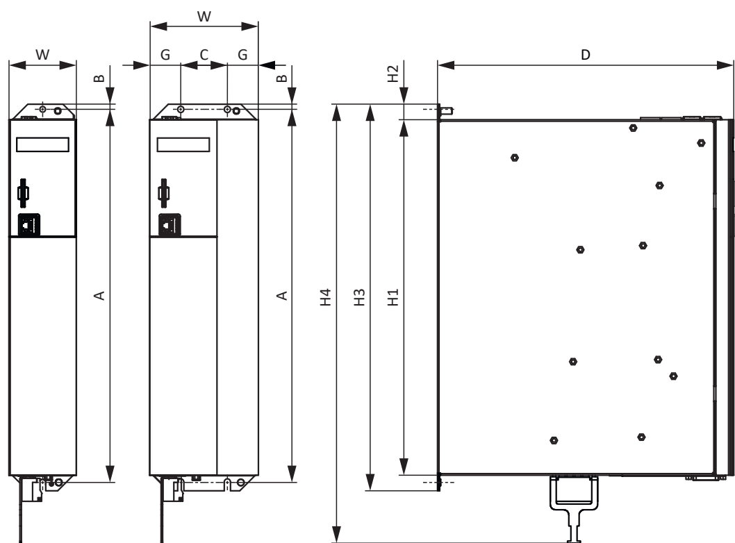
Abb. 2: Maßzeichnung SI6
