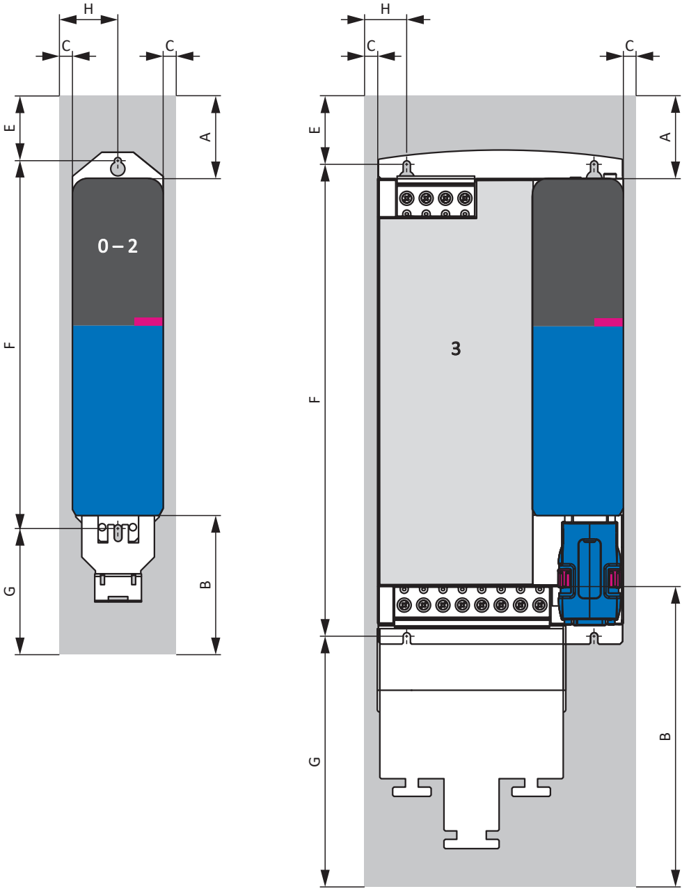
Abb. 3: Mindestfreiräume
