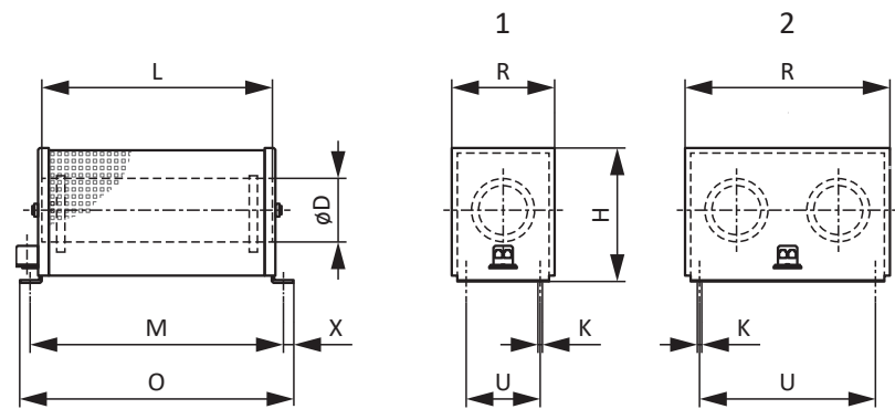
Abb. 3: Maßzeichnung FZMU (1), FZZMU (2)
