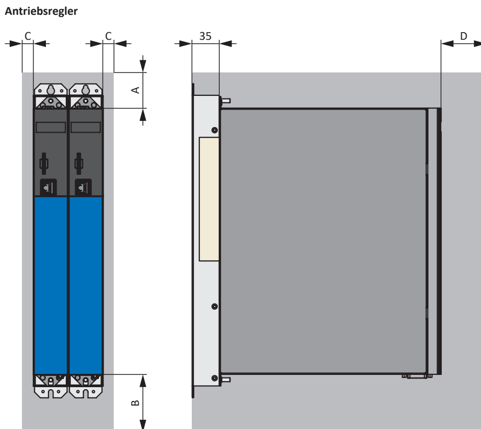
Abb. 3: Mindestfreiräume
