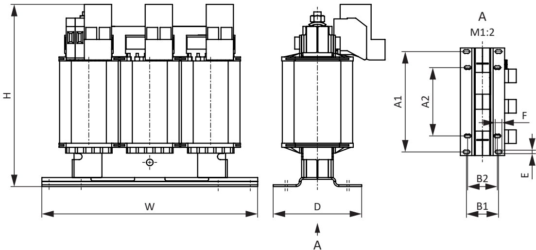
Abb. 8: Maßzeichnung TEP
