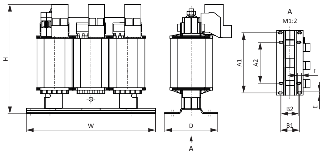
Abb. 6: Maßzeichnung TEP
