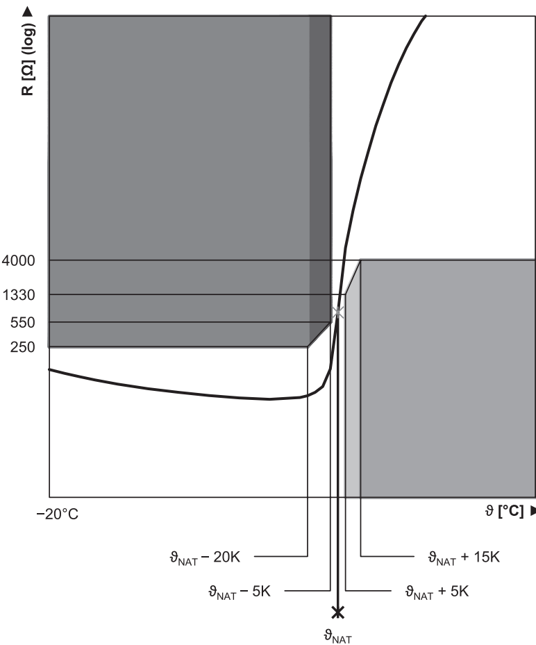
Abb. 2: Kennlinie PTC-Thermistor (einzelner Kaltleiter)
