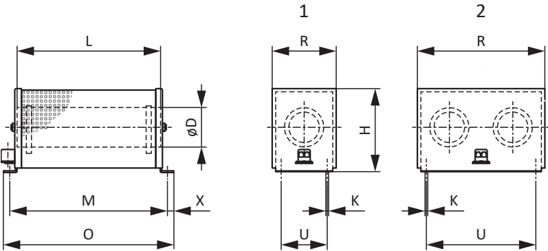
Abb. 4: Maßzeichnung FZMU (1), FZZMU (2)
