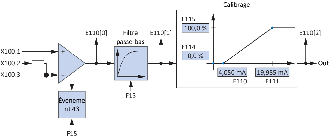
Fig. 12: Organigramme des signaux : entrée analogique AI1 (F116 = 2: De 4 à 20mA)
