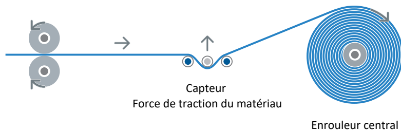
Fig. 21: Structure : enrouleur central avec régulation de la force de traction
