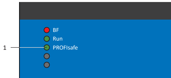
Abb. 70: Leuchtdiode für den PROFIsafe-Zustand
