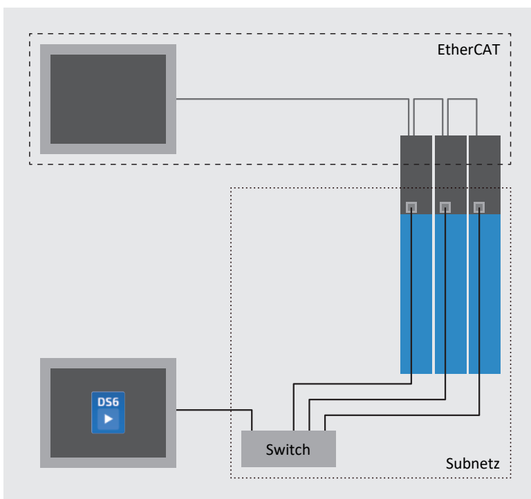
Abb. 76: Multiachs-Scope: Netzwerkaufbau
