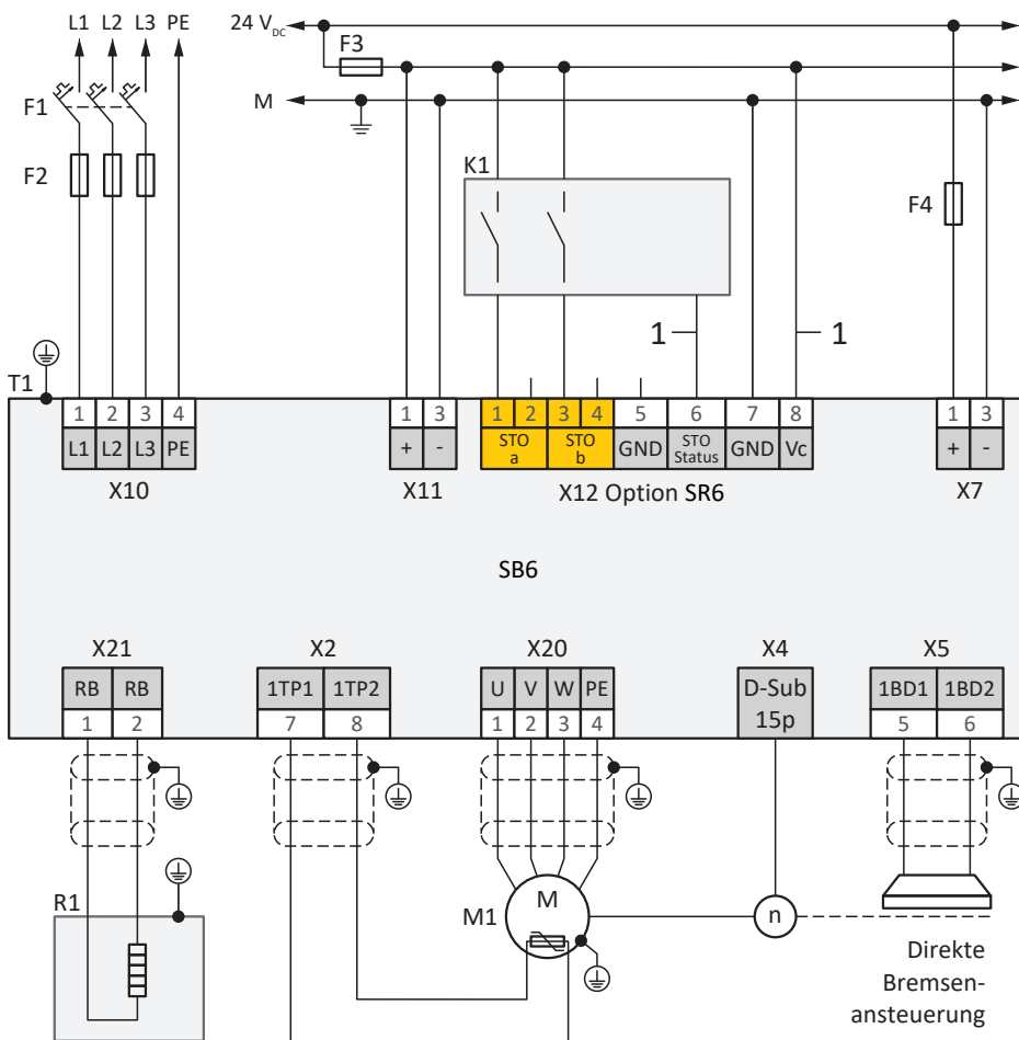
Abb. 77: Verschaltungsbeispiel mit direkter Bremsenansteuerung
