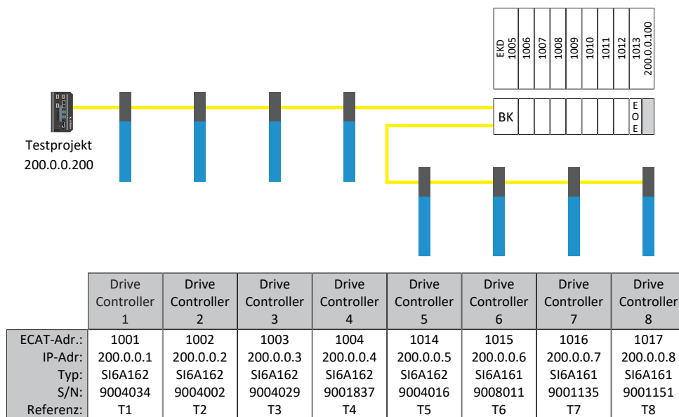
Abb. 80: Testaufbau der Anwendungsbeispiele
