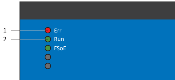
Abb. 67: Leuchtdioden für den EtherCAT-Zustand
