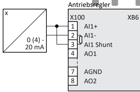
Abb. 26: X100: Anschlussbeispiel Sensor 1
