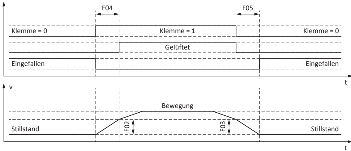
Abb. 55: Bremsenansteuerung bei Steuerart B20 = 0: ASM - U/f-Steuerung oder 1: ASM - U/f-Schlupfkompenziert
