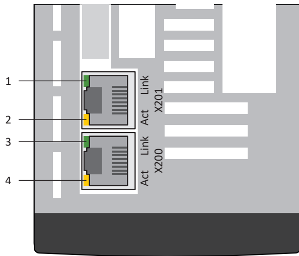
Abb. 73: Leuchtdioden für den Zustand der PROFINET-Netzwerkverbindung
