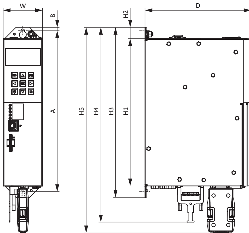
Abb. 5: Maßzeichnung SB6
