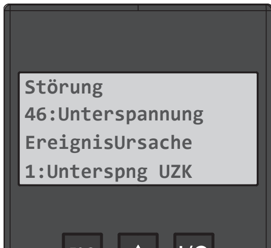
Abb. 66: Anzeige einer Störung am Display
