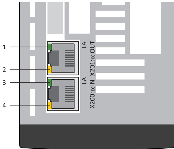
Abb. 72: Leuchtdioden für den Zustand der EtherCAT-Netzwerkverbindung
