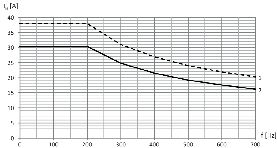
Abb. 11: Derating des Nennstroms in Abhängigkeit von der Taktfrequenz, TEP4020-0RS41
