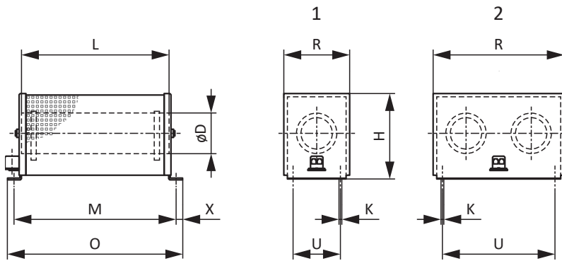
Abb. 6: Maßzeichnung FZMU (1), FZMU (2)
