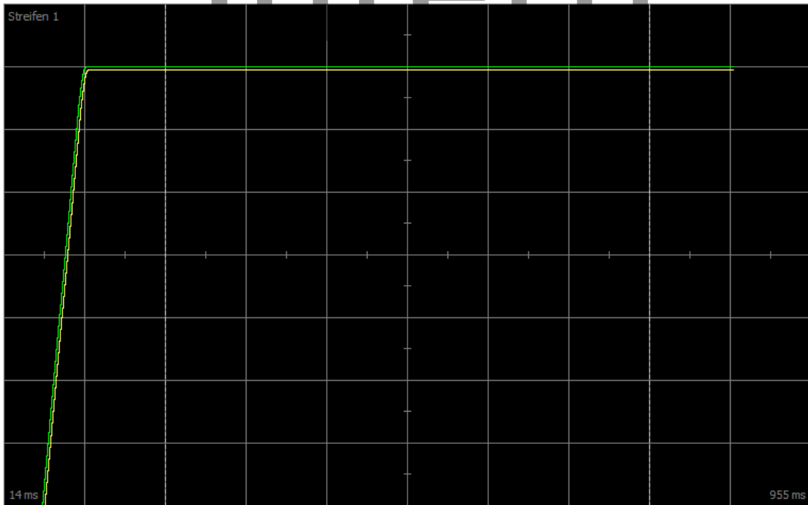
Abb. 44: Scope – Proportionalbeiwert des Geschwindigkeitsreglers (C31), optimierter Wert
