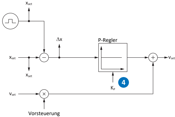
Abb. 48: Positionsregler – Proportionalbeiwert
