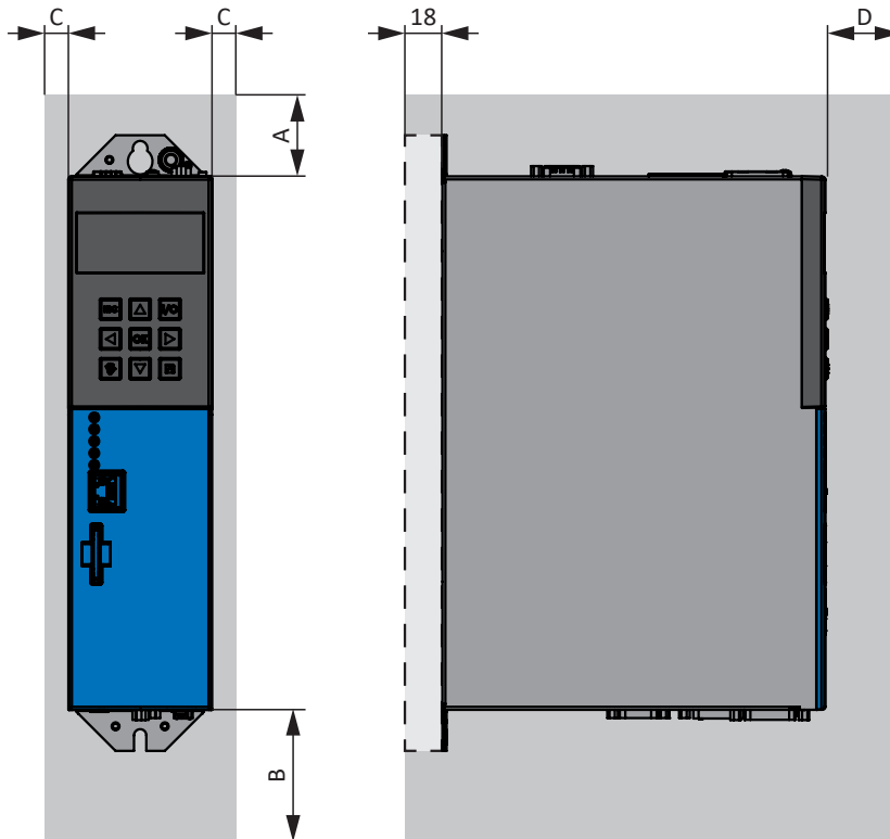
Abb. 16: Mindestfreiräume
