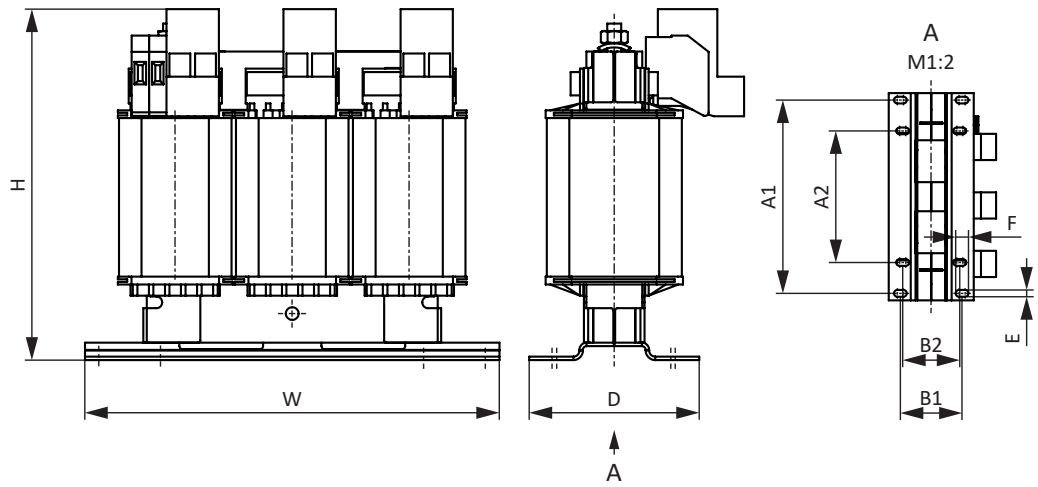
Abb. 5: Maßzeichnung TEP
