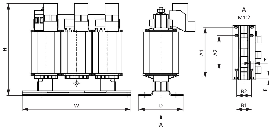
Abb. 14: Maßzeichnung TEP
