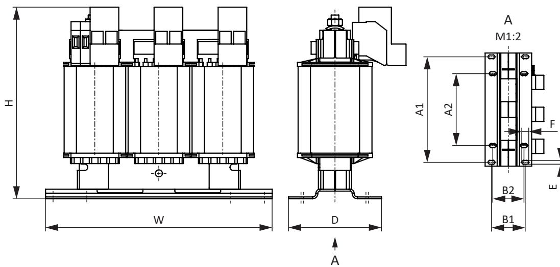
Abb. 8: Maßzeichnung TEP
