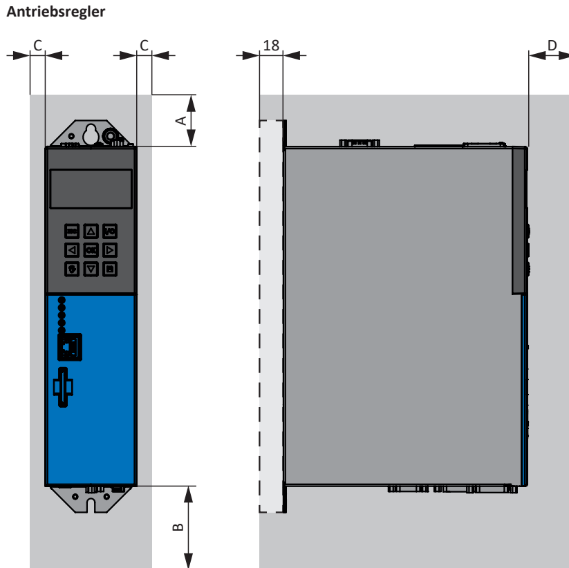
Abb. 2: Mindestfreiräume
