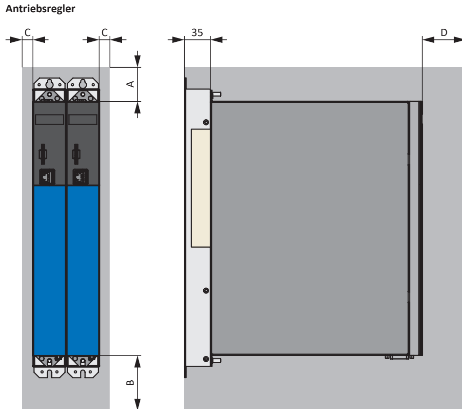
Abb. 3: Mindestfreiräume
