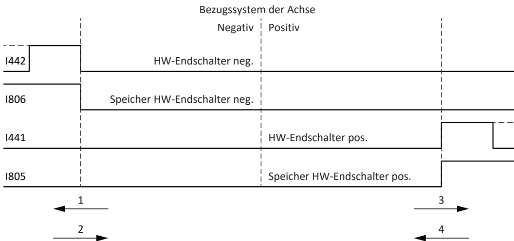
Abb. 43: HW-Endschalterspeicher
