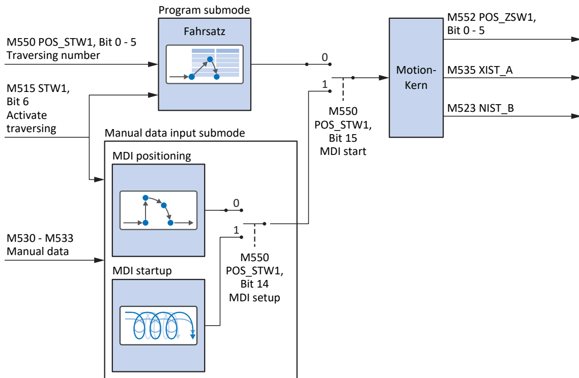
Abb. 32: Siemens Telegramm 111 in AC3: Ein- und Ausgangssignale
