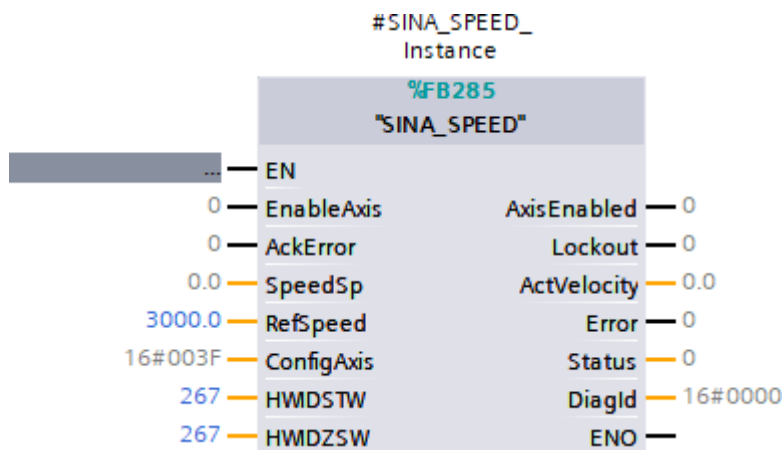
Abb. 24: Funktionsbaustein SINA_SPEED
