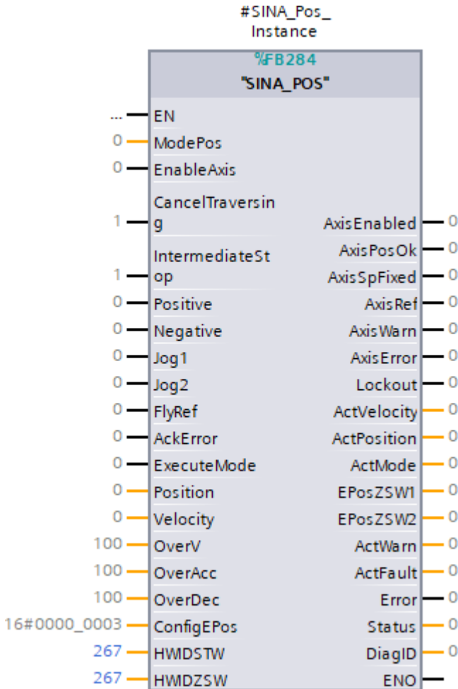
Abb. 25: Funktionsbaustein SINA_POS
