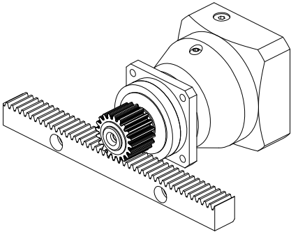
Fig. 3: Asignación recomendada de los rodamientos S (p. ej., con dentado recto)
