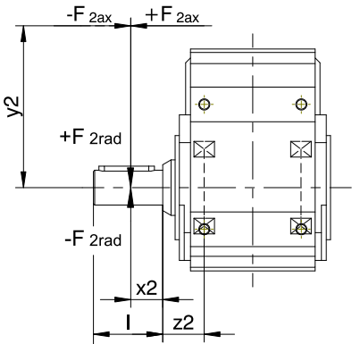
Fig. 3: Puntos de incisión de la fuerza para el eje macizo
