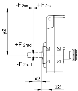
Fig. 4: Puntos de incisión de la fuerza para el eje hueco
