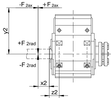
Fig. 4: Puntos de incisión de la fuerza para el eje hueco
