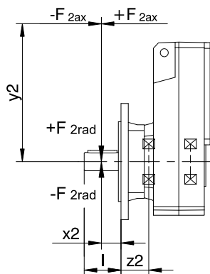
Fig. 3: Puntos de incisión de la fuerza para el eje macizo
