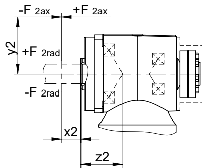
Fig. 4: Puntos de incisión de la fuerza para el eje hueco con anillo de contracción
