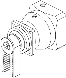
Fig. 4: Asignación recomendada de los rodamientos Z (p. ej., con accionamientos de correa)
