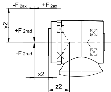
Fig. 3: Puntos de incisión de la fuerza para el eje hueco con brida
