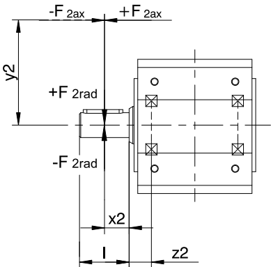
Fig. 2: Puntos de incisión de la fuerza para el eje macizo
