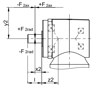
Fig. 5: Puntos de incisión de la fuerza para el eje macizo
