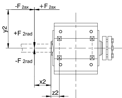
Fig. 3: Puntos de incisión de la fuerza para el eje hueco
