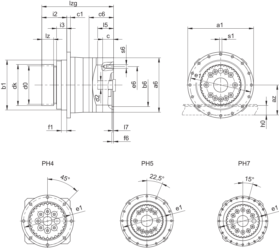
出力寸法
