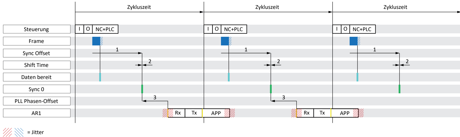
Abb. 18: CODESYS V3: DC-Sync – stabile Synchronisation, Zykluszeit < 1 ms
