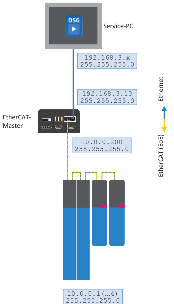
Abb. 9: Netzwerkübersicht: Topologie 2
