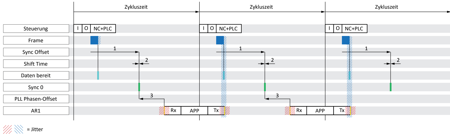
Abb. 17: CODESYS V3: DC-Sync – instabile Synchronisation, Zykluszeit < 1 ms
