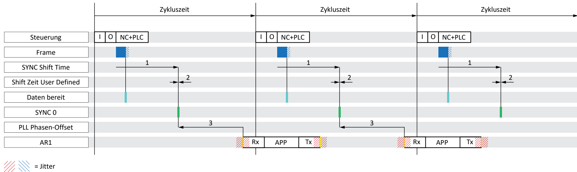
Abb. 13: TwinCAT 3: DC-Sync – Einstellungen
