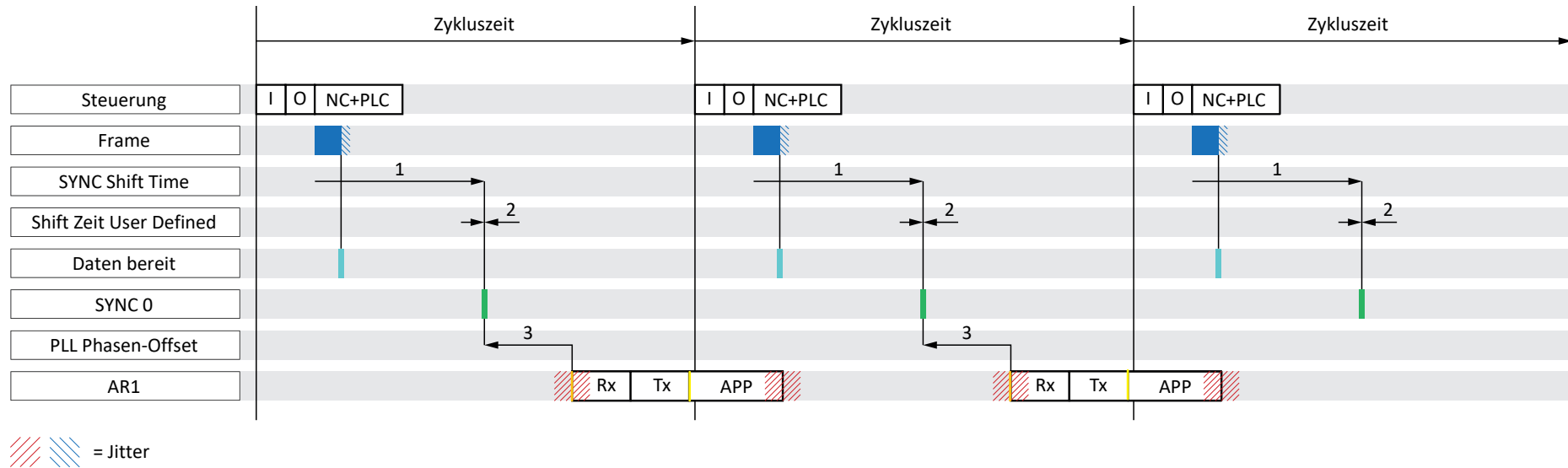
Abb. 15: TwinCAT 3: DC-Sync – stabile Synchronisation, Zykluszeit < 1 ms
