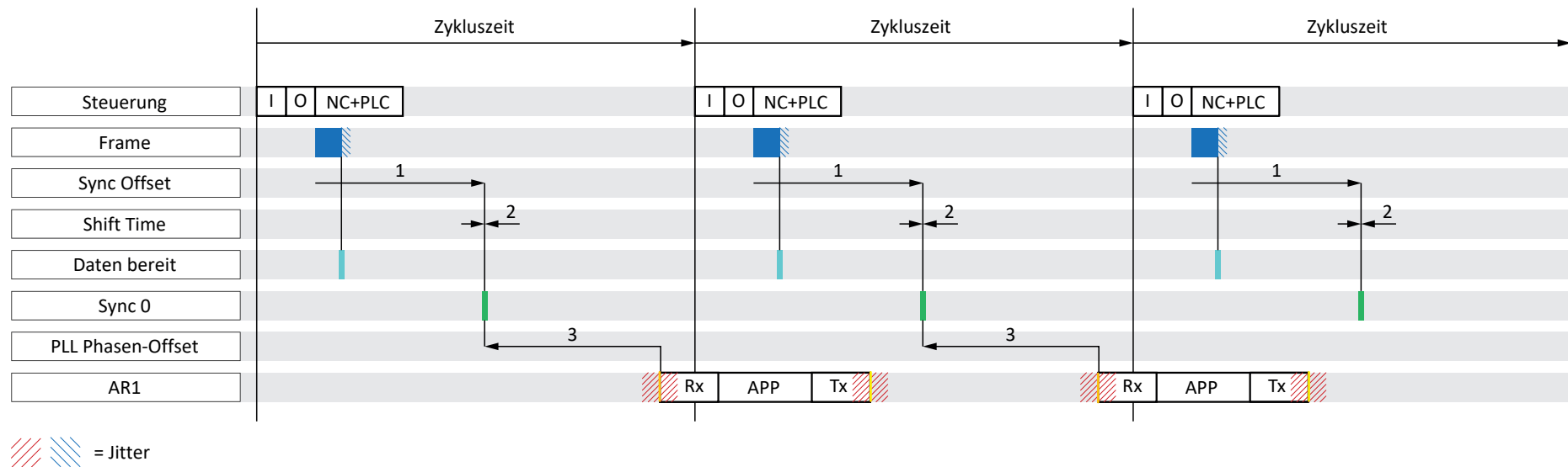
Abb. 16: CODESYS V3: DC-Sync – Einstellungen
