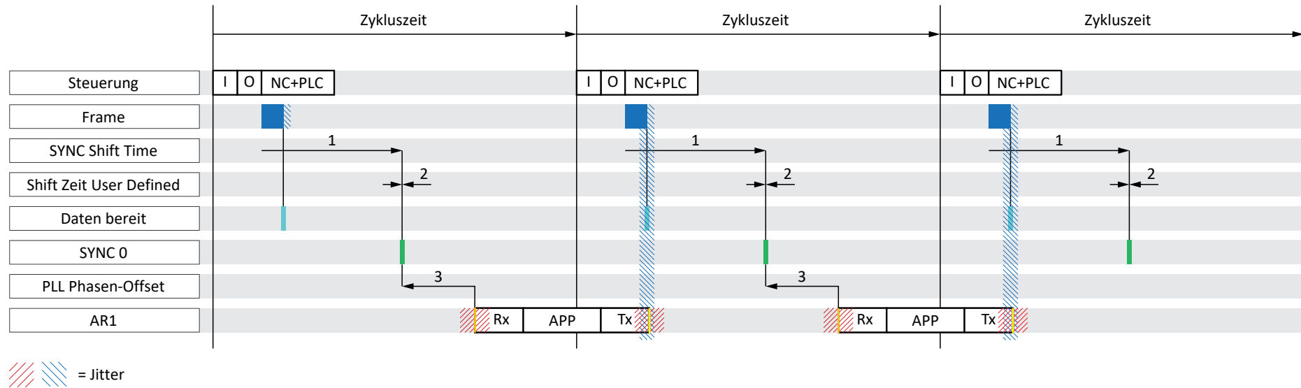
Abb. 14: TwinCAT 3: DC-Sync – instabile Synchronisation, Zykluszeit < 1 ms
