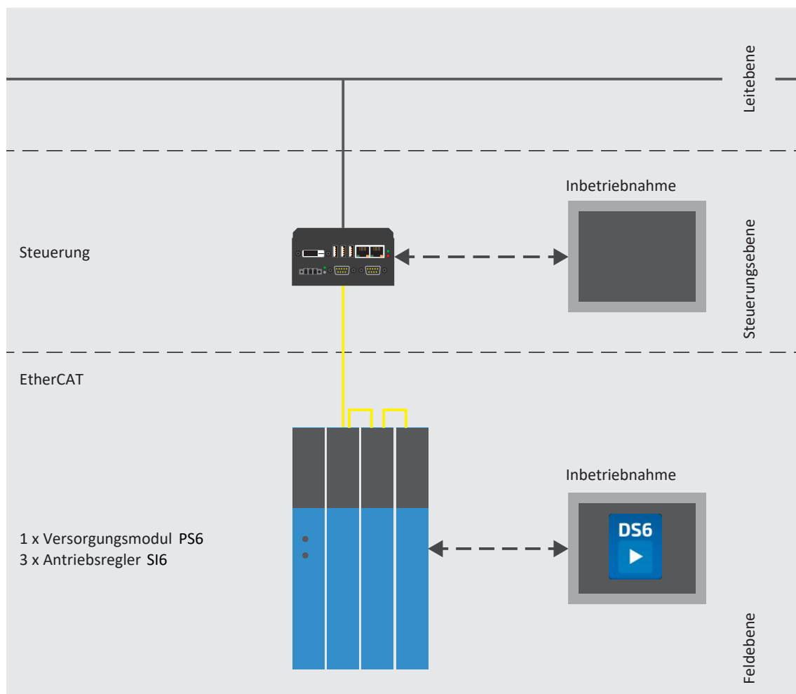
Abb. 1: EtherCAT: Netzwerkaufbau am Beispiel der Baureihe SI6
