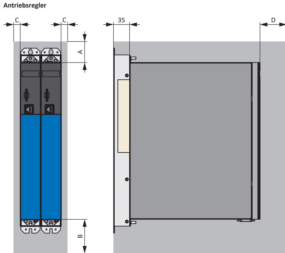
Abb. 3: Mindestfreiräume
