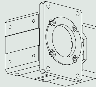
Gewindelochkreis + Drehmomentstütze GD
