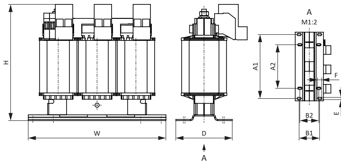
Abb. 5: Maßzeichnung TEP
