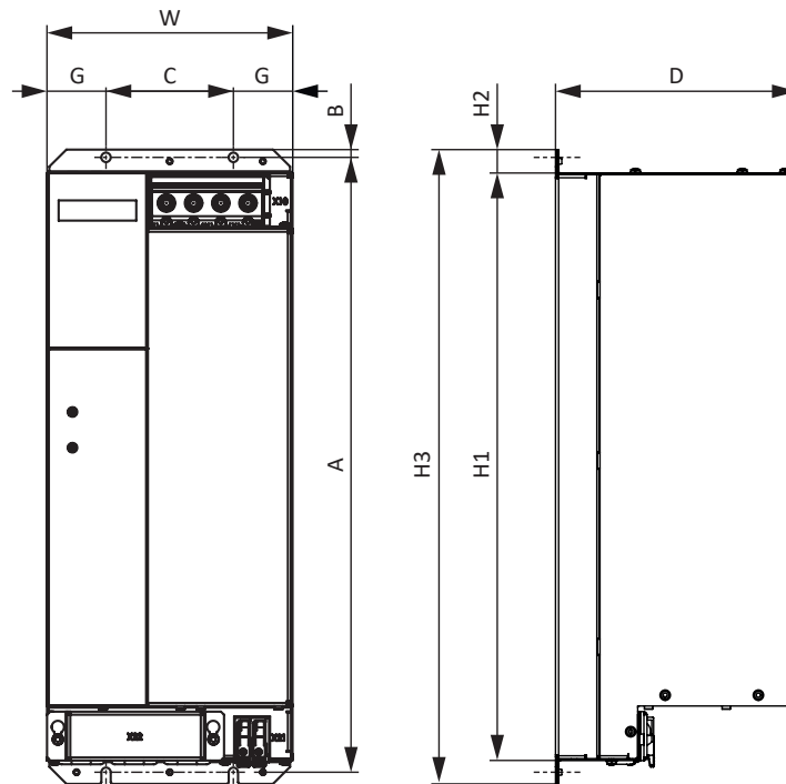
Abb. 2: Maßzeichnung PS6A44
