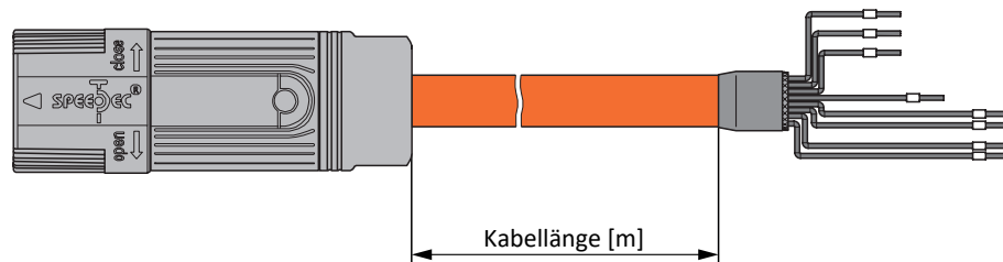
Abb. 1: Längendefinition für konfektionierte Leistungskabel
