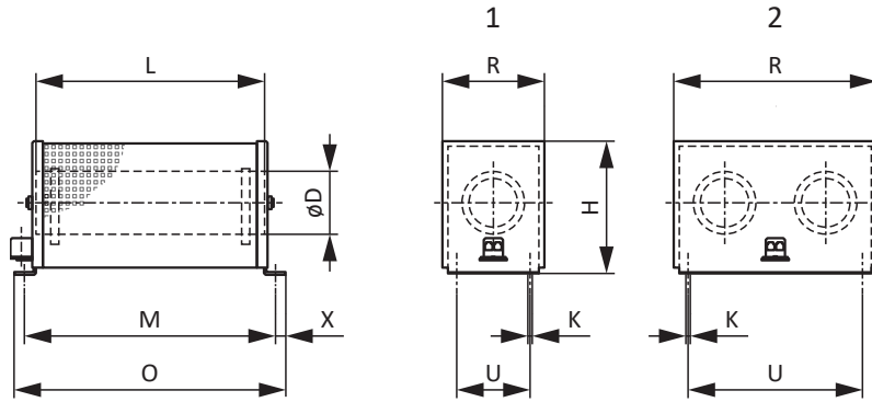
Abb. 3: Maßzeichnung FZMU (1), FZZMU (2)
