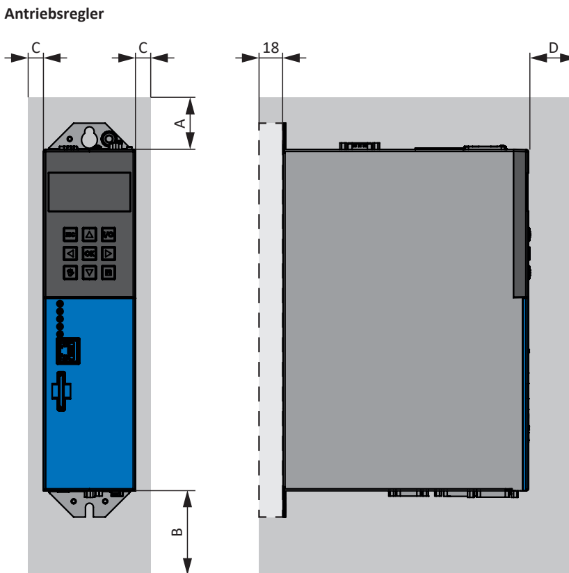
Abb. 2: Mindestfreiräume
