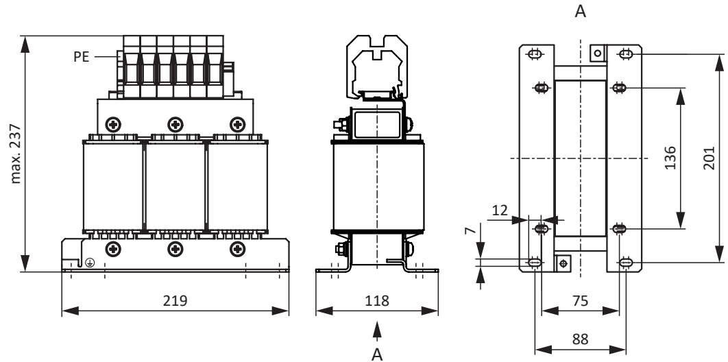
Abb. 13: Maßzeichnung Netzdressel
