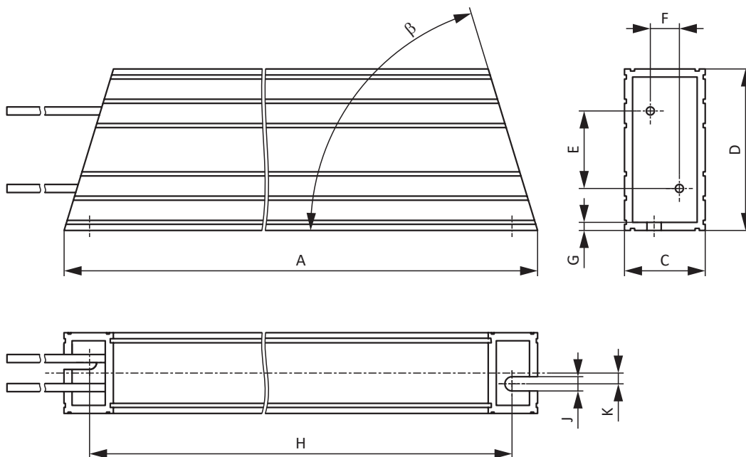
Abb. 4: Maßzeichnung GVADU, GBADU
