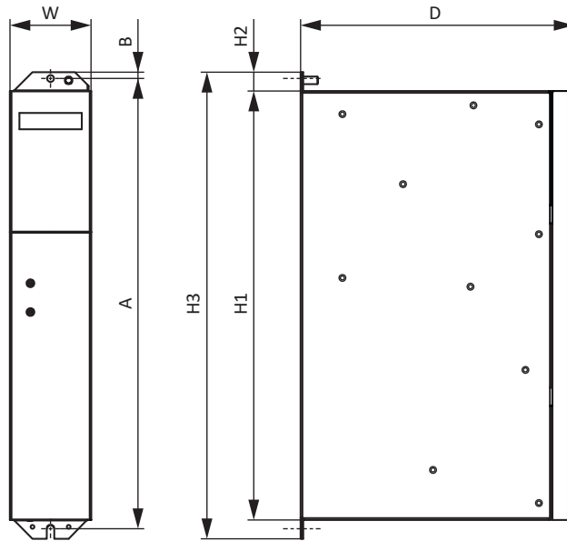
Abb. 1: Maßzeichnung PS6A24, PS6A34
