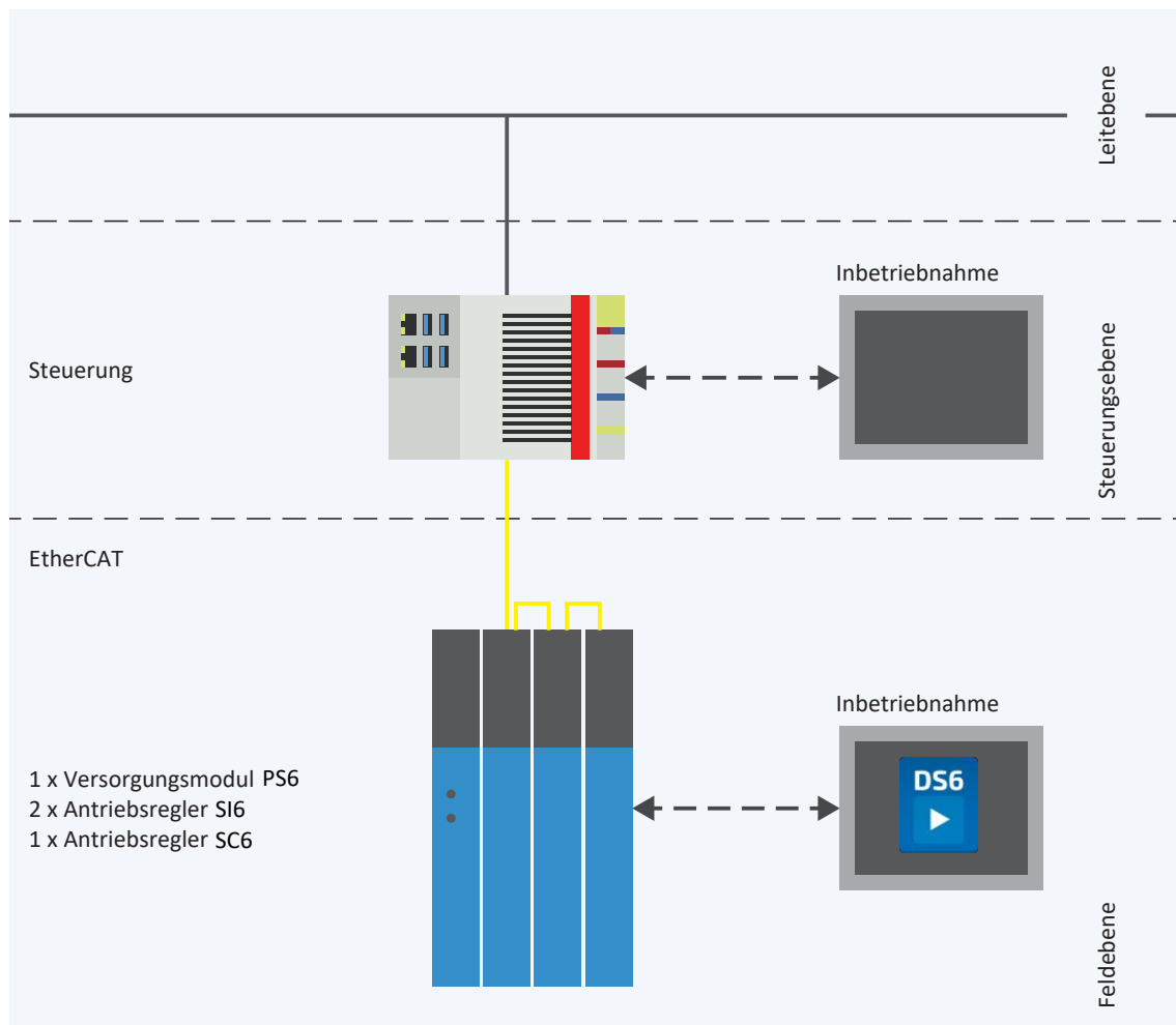
Abb. 1: EtherCAT: Netzwerkaufbau
