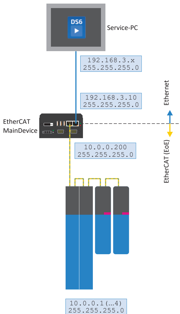
Abb. 10: Netzwerkübersicht: Topologie 2
