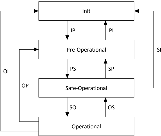
Abb. 11: EtherCAT State Machine: Zustände und Zustandswechsel
