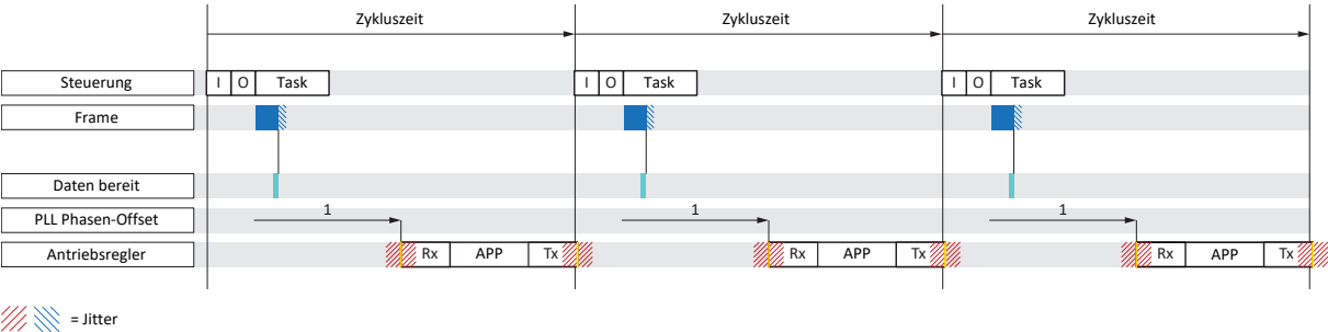
Abb. 12: SM-Sync: Synchronisation durch SyncManager-Event
