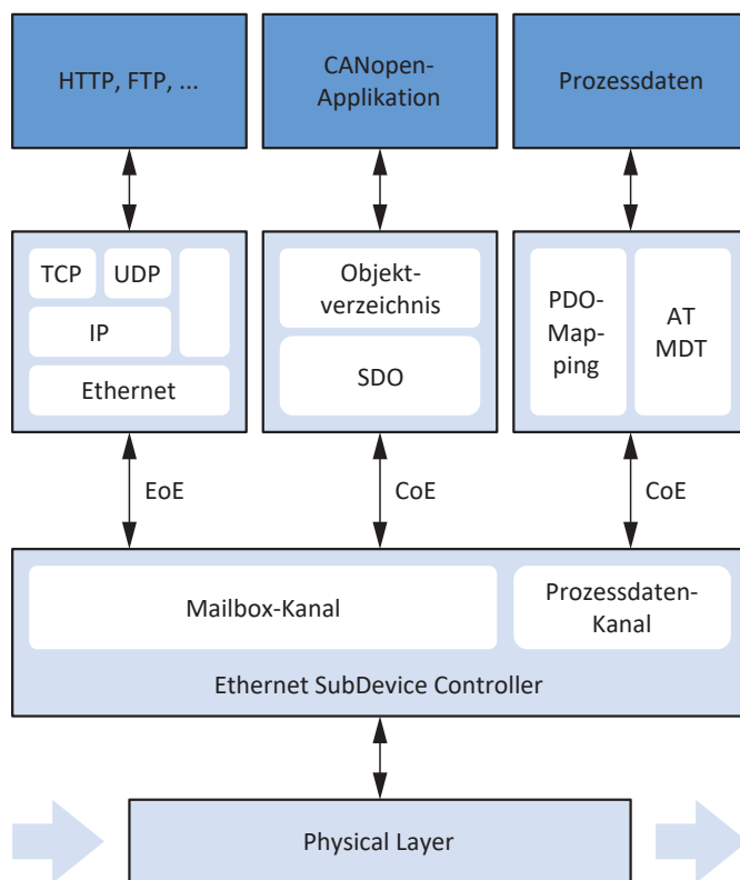
Abb. 8: EtherCAT: Kommunikationsprotokolle
