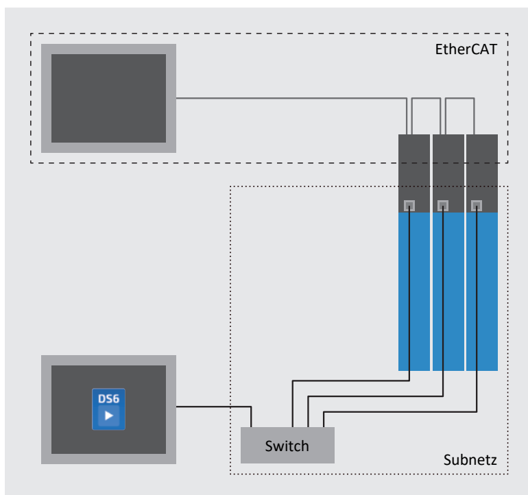
Abb. 76: Multiachs-Scope: Netzwerkaufbau
