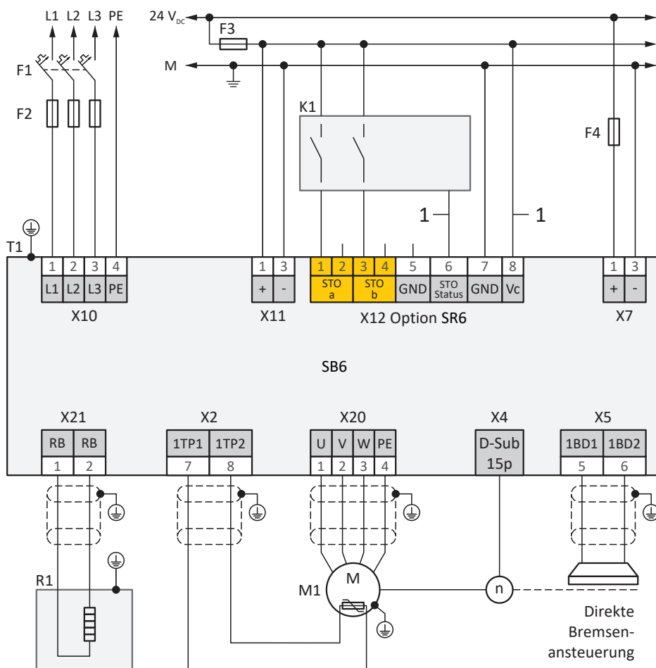
Abb. 77: Verschaltungsbeispiel mit direkter Bremsenansteuerung
