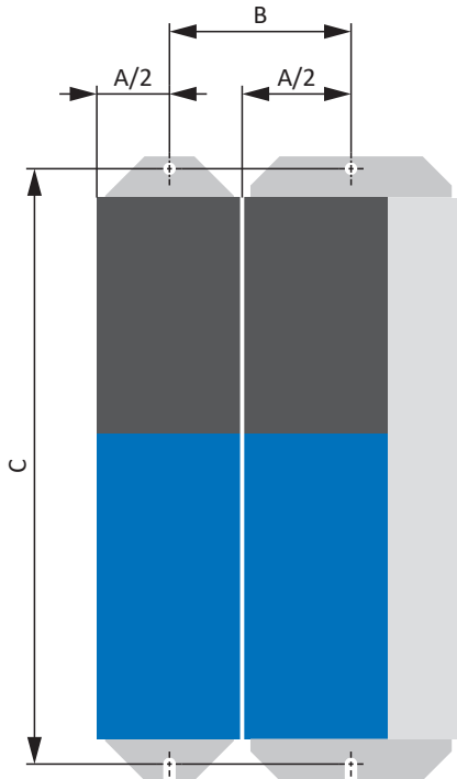
Abb. 17: Bohrplan SB6
