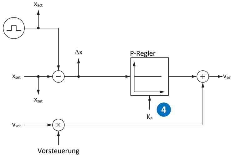
Abb. 48: Positionsregler – Proportionalbeiwert
