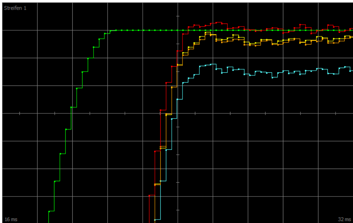
Abb. 47: Scope – Integrierbeiwert des Geschwindigkeitsreglers (C32)
