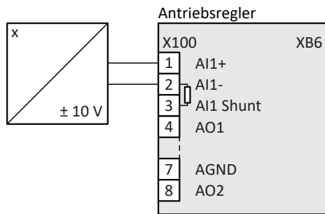
Abb. 27: X100: Anschlussbeispiel Sensor 2
