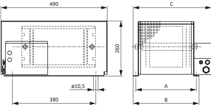
Abb. 6: Maßzeichnung FGFKU
