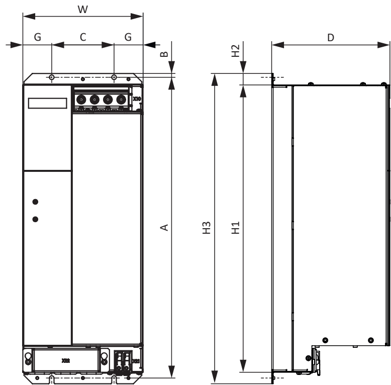
Abb. 4: Maßzeichnung PS6A44
