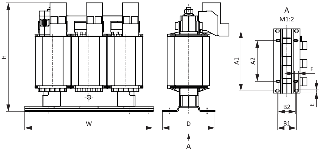
Abb. 5: Maßzeichnung TEP
