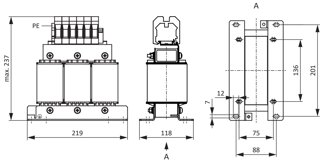
Abb. 7: Maßzeichnung Netzdrössel
