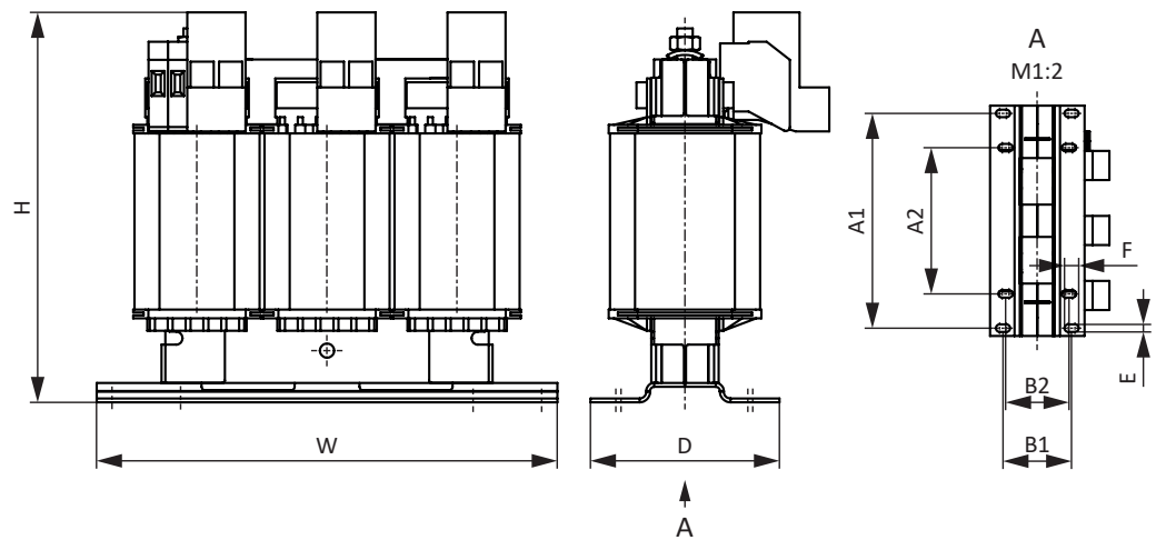
Abb. 8: Maßzeichnung TEP
