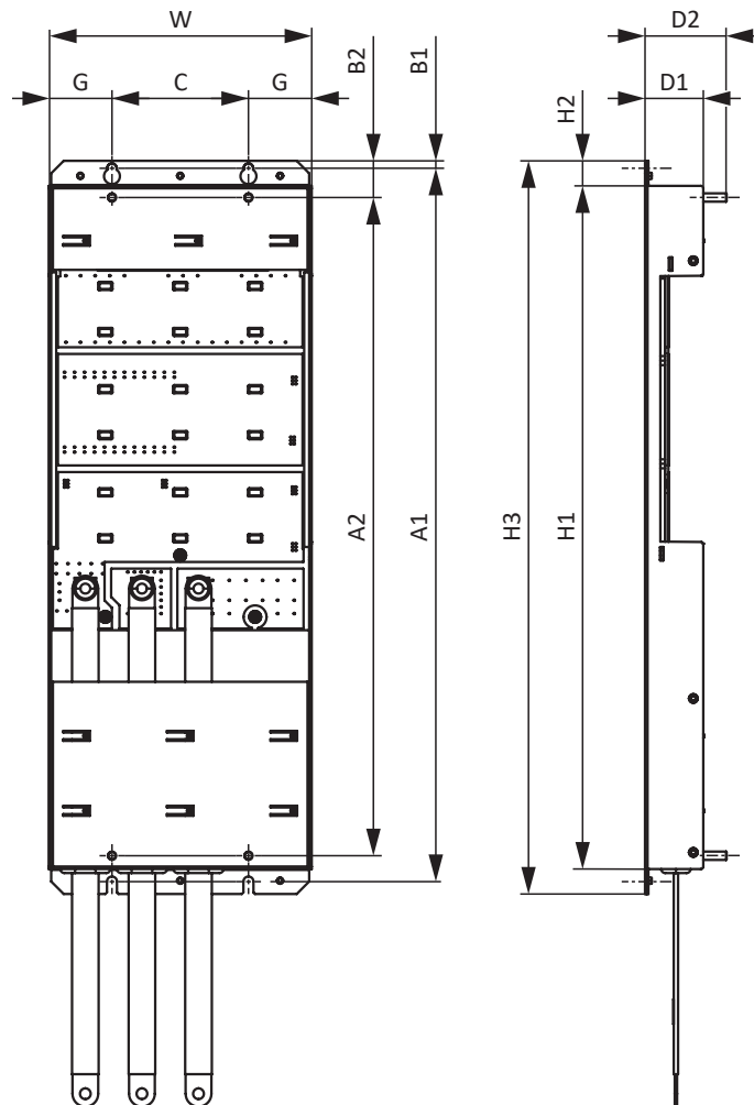
Abb. 6: Maßzeichnung DL6B22
