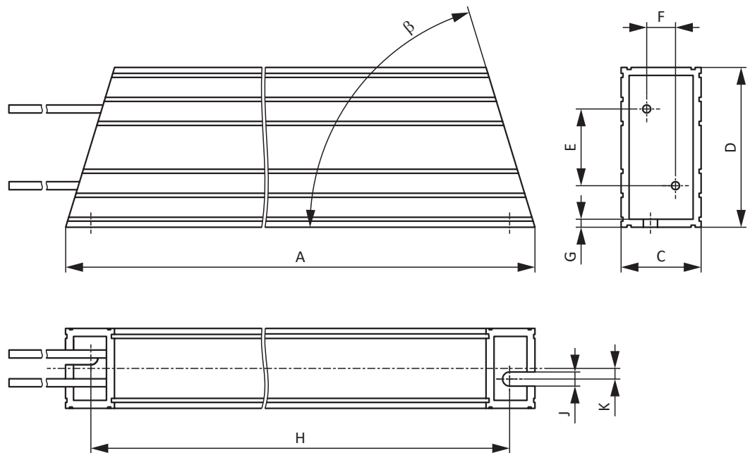
Abb. 5: Maßzeichnung GVADU, GBADU
