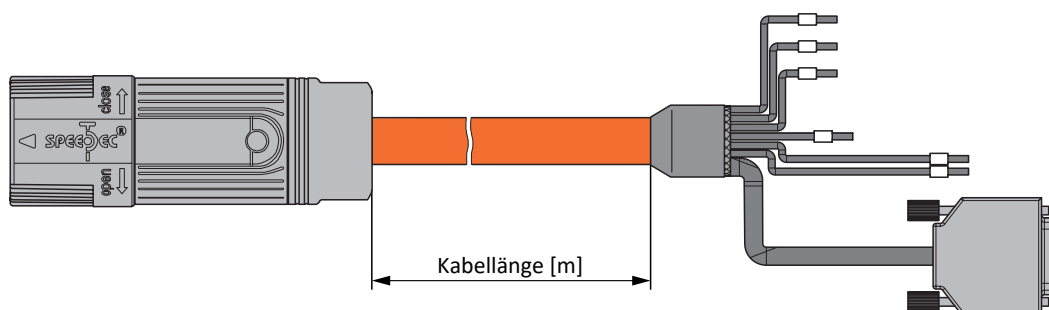
Abb. 4: Längendefinition für konfektionierte Hybridkabel
