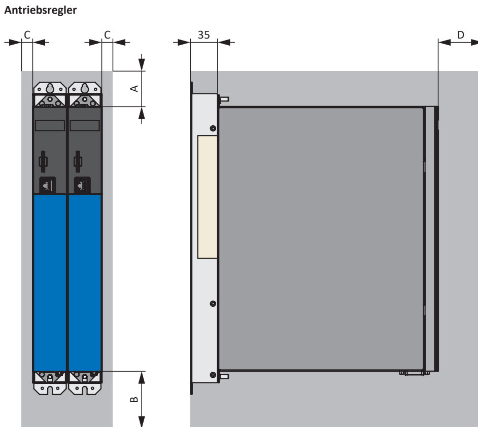
Abb. 3: Mindestfreiräume
