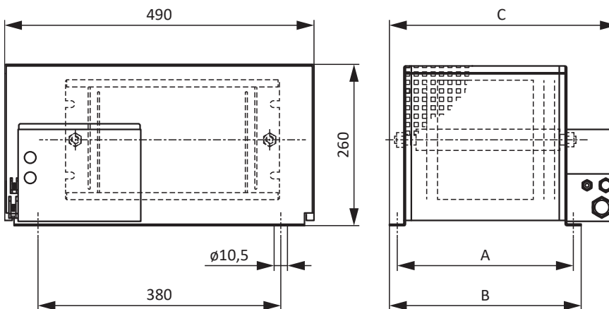
Abb. 6: Maßzeichnung FGFKU
