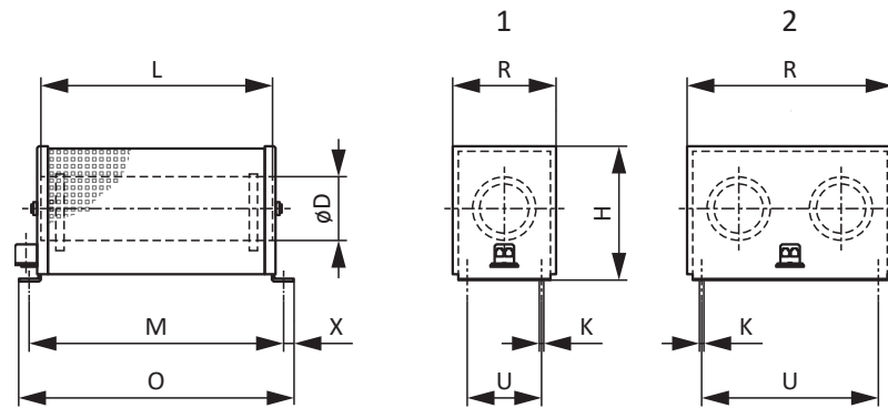
Abb. 3: Maßzeichnung FZMU (1), FZZMU (2)
