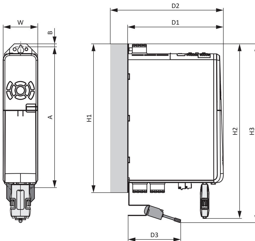
Abb. 1: Maßzeichnung SD6, Baugrößen 0 bis 2
