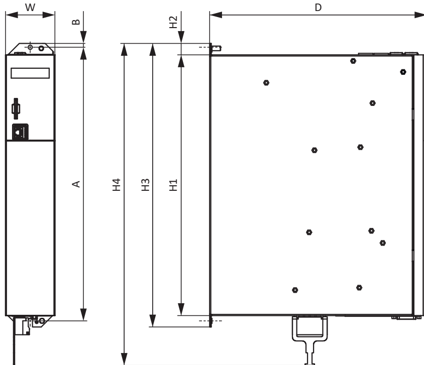
Abb. 2: Maßzeichnung SC6
