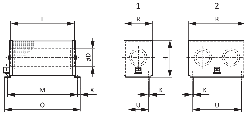
Abb. 4: Maßzeichnung FZMU (1), FZZMU (2)
