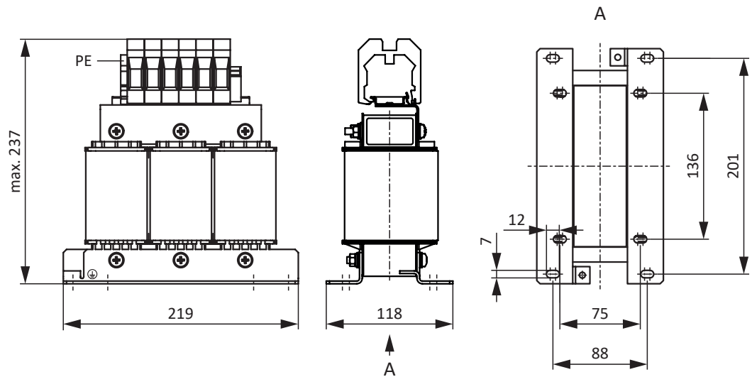
Abb. 13: Maßzeichnung Netzdrössel
