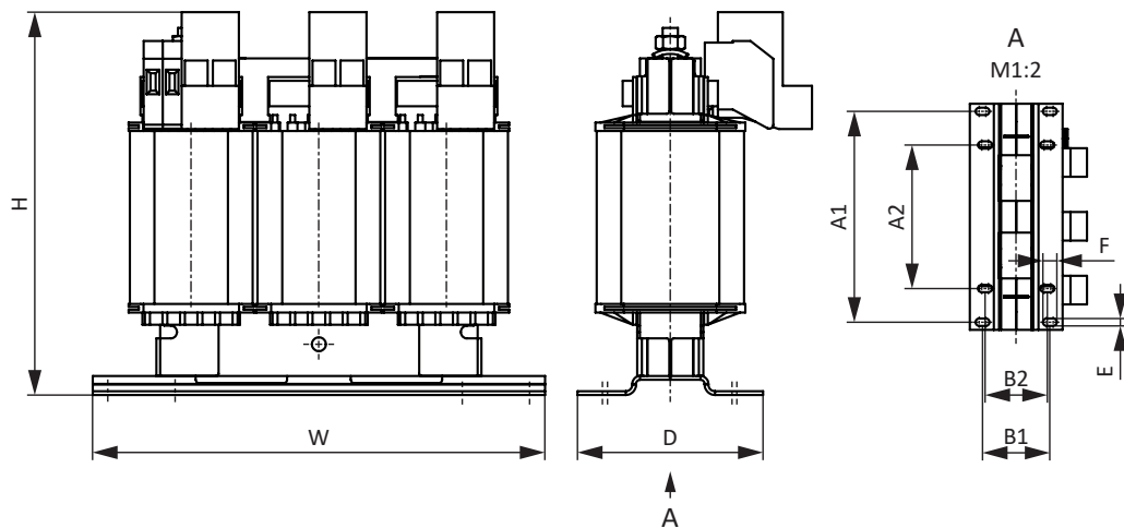
Abb. 6: Maßzeichnung TEP
