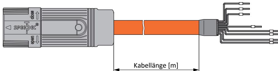
Abb. 2: Längendefinition für konfektionierte Leistungskabel – SC6, SI6
