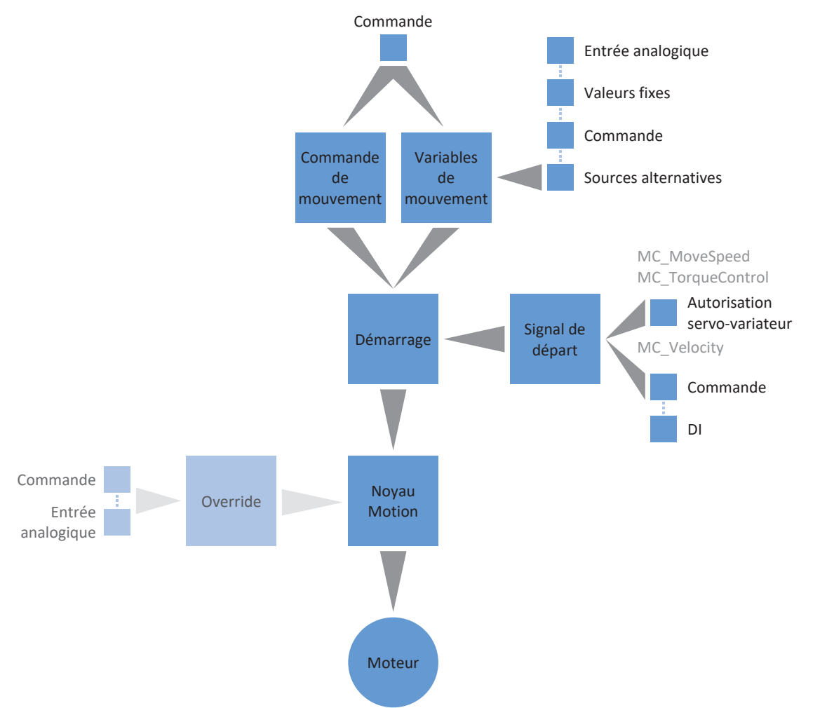
Fig. 3: Mode d'exploitation Vitesse, couple/force : flux de signaux
