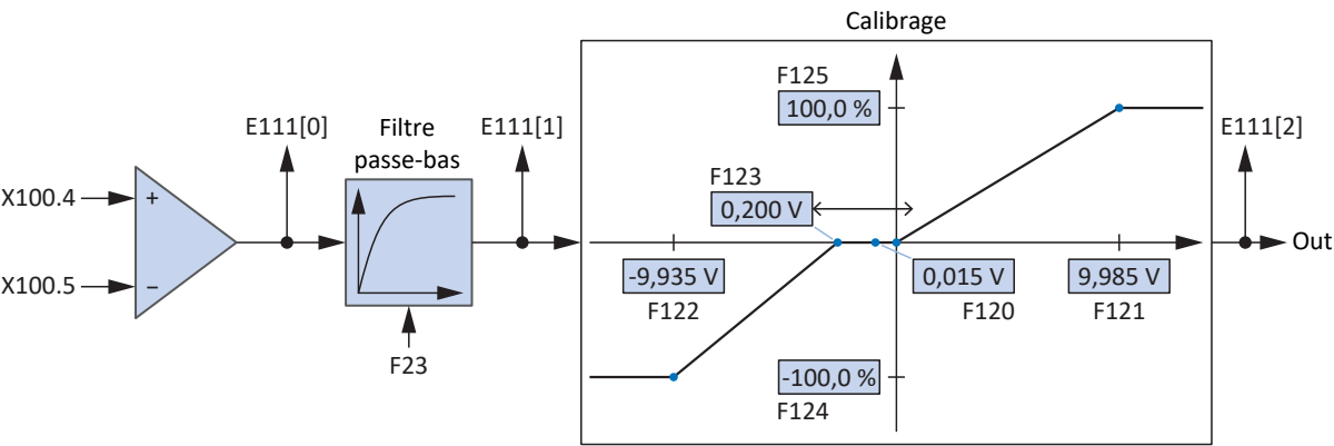
Fig. 10: Organigramme des signaux : entrée analogique AI2
