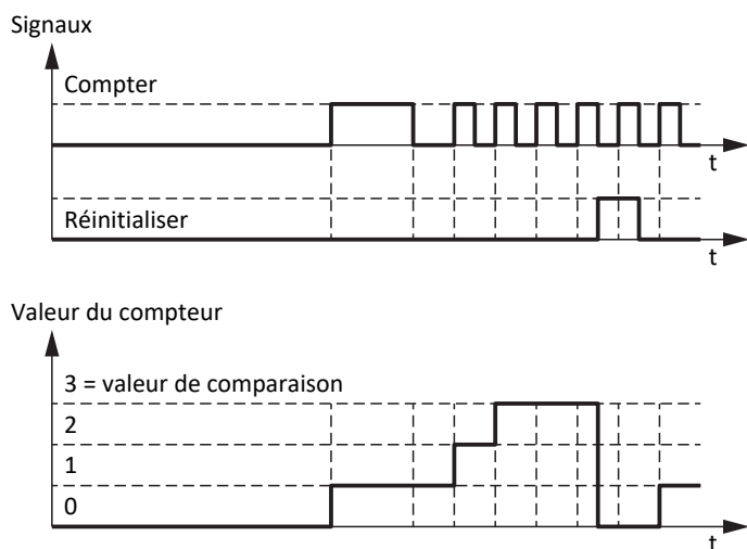
Fig. 10: Fonction additionnelle Compteur : exemple
