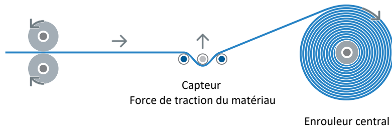
Fig. 16: Structure : enrouleur central avec régulation de la force de traction
