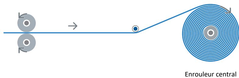
Fig. 18: Enrouleur central : enroulement positif (enroulement par le haut)
