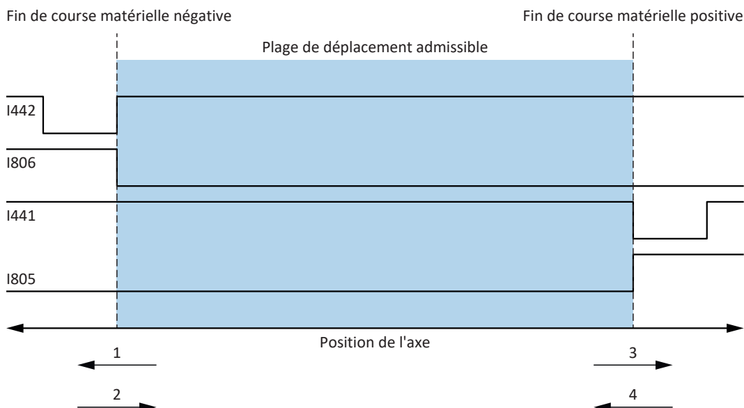
Fig. 25: Fins de course matérielles : mémoire des fins de course
