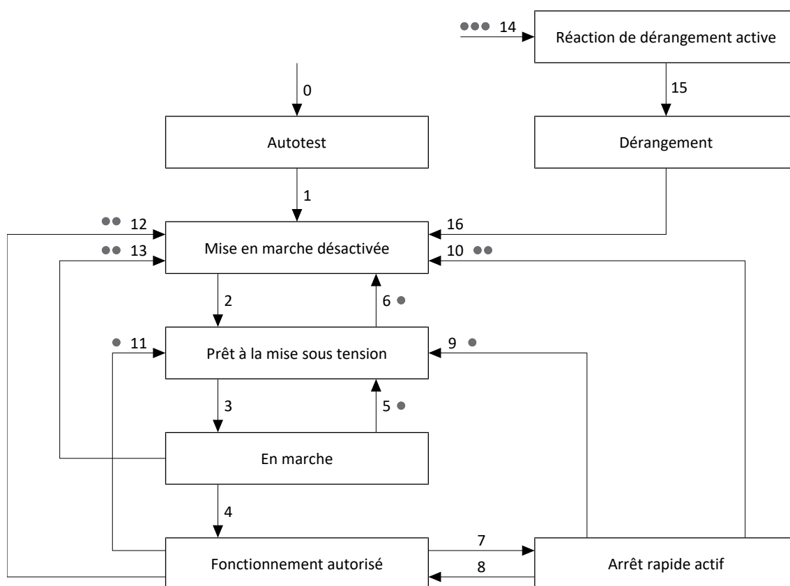
Fig. 26: Machine d'état Drive Based : états de l'appareil et changement d'état
