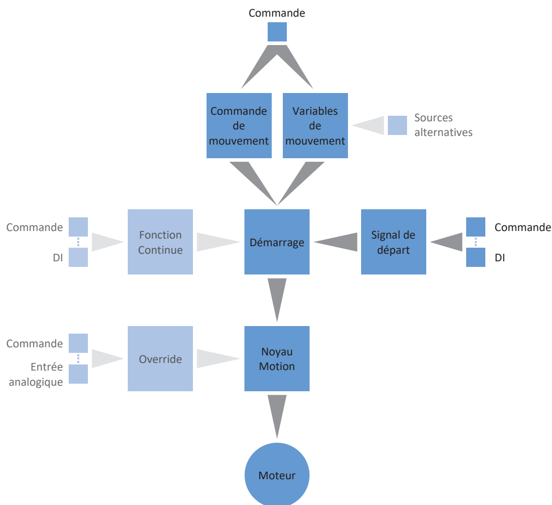
Fig. 6: Mode d'exploitation Commande : flux de signaux
