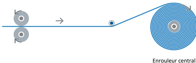
Fig. 15: Structure : enrouleur central avec commande de force de traction
