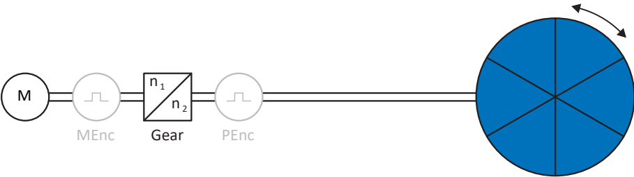
Fig. 24: Mouvement rotatoire sans fin : plateau rotatif indexé
