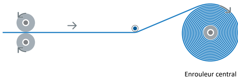
Fig. 13: Structure : enrouleur central avec commande de vitesse
