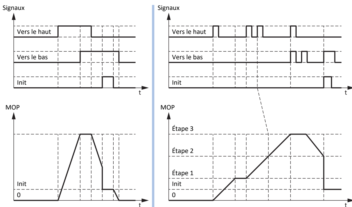
Fig. 11: Potentiomètre moteur : calcul linéaire et incrémentiel
