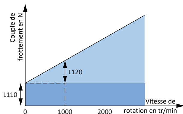
Fig. 22: Enrouleur central : couple de frottement de l'axe
