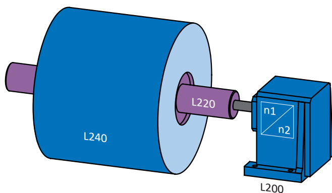
Fig. 23: Enrouleur central : moment d'inertie de masse de l'axe
