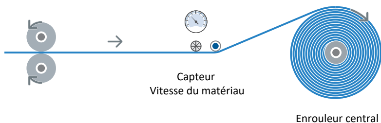
Fig. 14: Structure : enrouleur central avec régulation de vitesse
