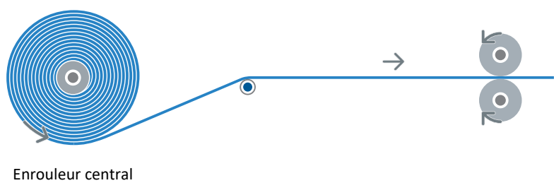
Fig. 20: Enrouleur central : déroulement positif
