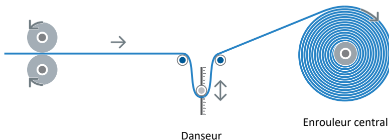
Fig. 17: Structure : enrouleur central avec régulation de la position du danseur
