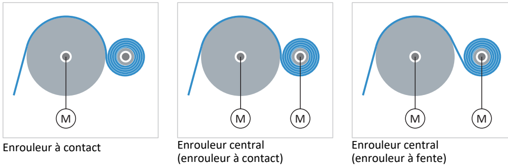
Fig. 12: Enrouleur central : types
