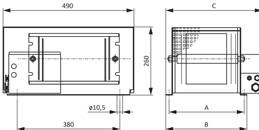
Abb. 16: Maßzeichnung FGFKQU
