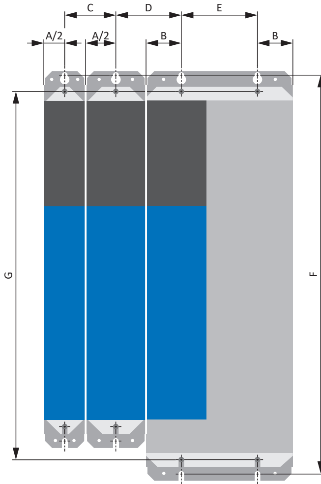
Abb. 36: Bohrplan DL6B22
