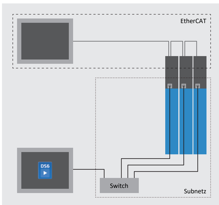
Abb. 98: Multiachs-Scope: Netzwerkaufbau
