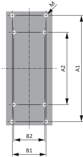
Abb. 42: Bohrplan TEP
