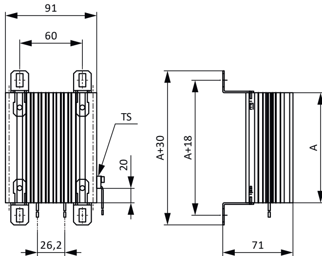
Abb. 13: Maßzeichnung KWADQU mit MWS306L
