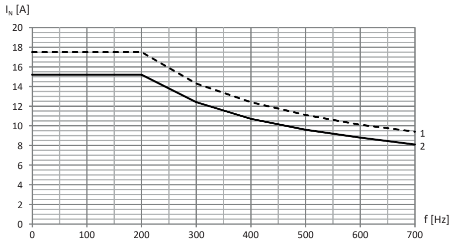
Abb. 24: Derating des Nennstroms in Abhängigkeit von der Taktfrequenz, TEP3820-0CS41
