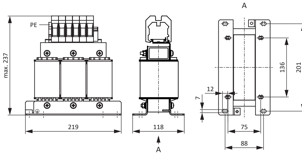
Abb. 17: Maßzeichnung Netzdrössel
