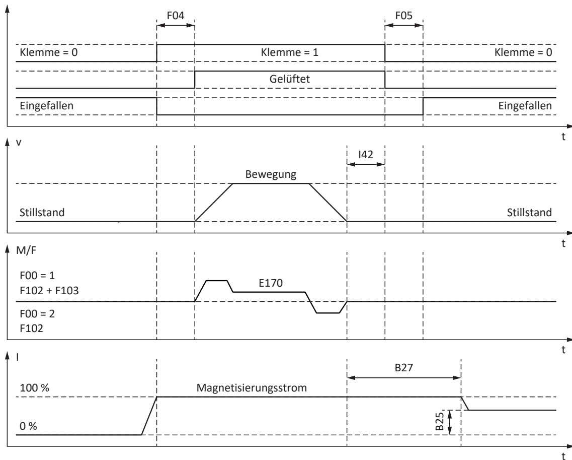
Abb. 76: Bremsenansteuerung bei Steuerart B20 = 2: ASM - Vektorregelung
