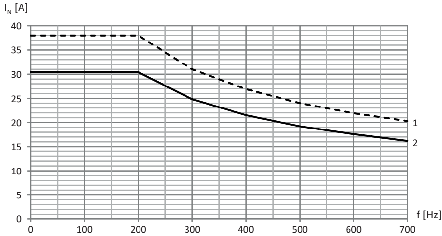
Abb. 25: Derating des Nennstroms in Abhängigkeit von der Taktfrequenz, TEP4020-ORS41
