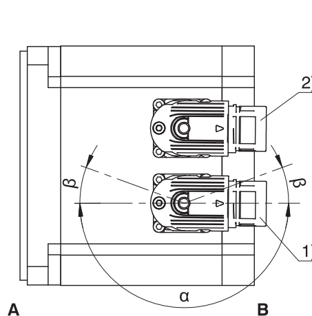
Verdrehbereiche der Steckverbinder (Motoren EZ4 – EZ8)
