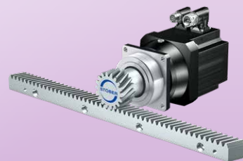
带同步伺服电机的齿轮齿条传动 ZVP 模数：2 - 4 mm 进给力：0.8 - 11 kN 进给速度：0.1 - 4.5 m/s 精确度高，适合各种典型的伺服应用。
