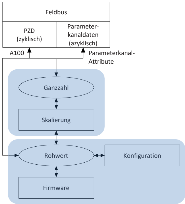
Abb. 14: Feldbusskalierung im Überblick
