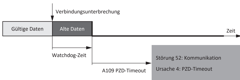
Abb. 6: PROFINET: Verbindungsüberwachung
