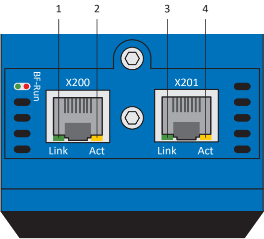
Abb. 8: Leuchtdioden für den Zustand der PROFINET-Netzwerkverbindung
