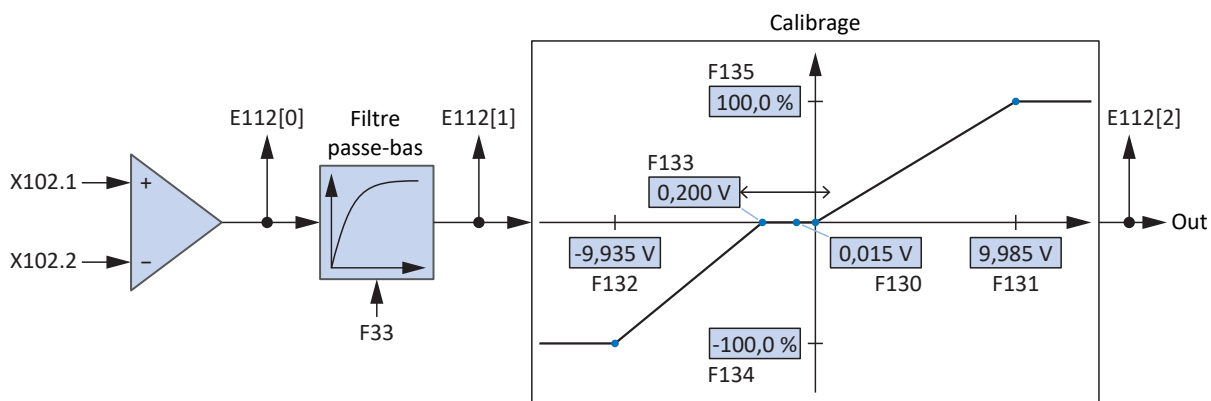
Fig. 11: Organigramme des signaux : entrée analogique AI3
