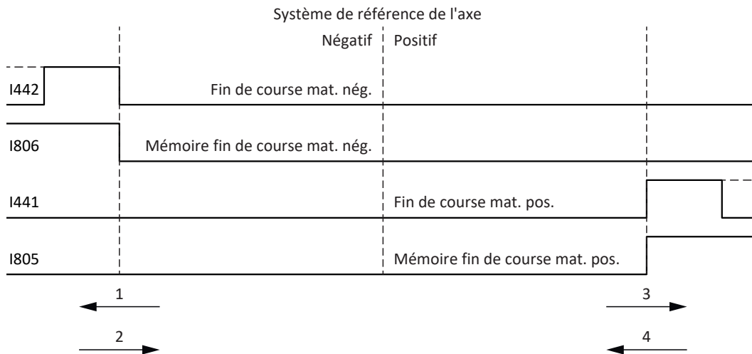
Fig. 19: Mémoire des fins de course matérielles
