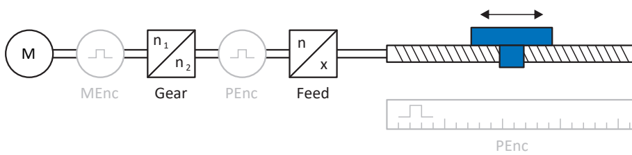
Fig. 17: Mouvement translatore limité : chariot porte-outils
