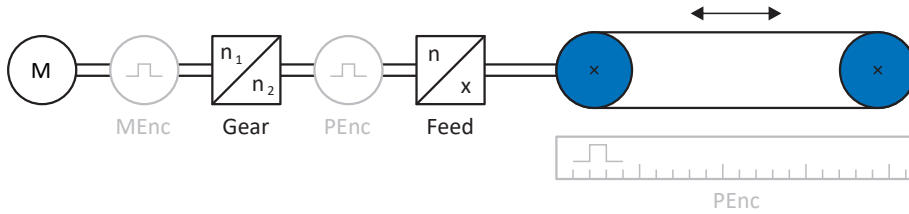
Fig. 16: Mouvement translatore sans fin : convoyeur
