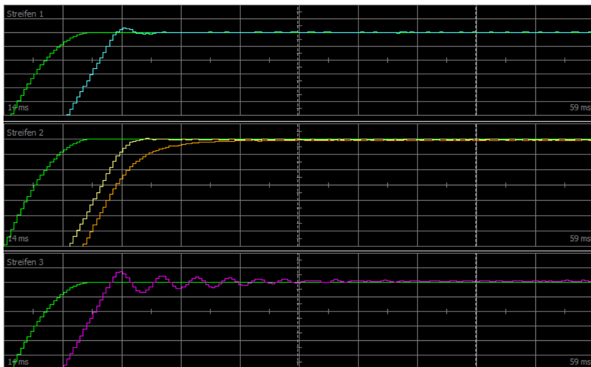
Abb. 45: Scope – Proportionalbeiwert des Geschwindigkeitsreglers (C31), Überschwingen
