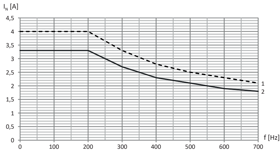
Abb. 9: Derating des Nennstroms in Abhängigkeit von der Taktfrequenz, TEP3720-0ES41
