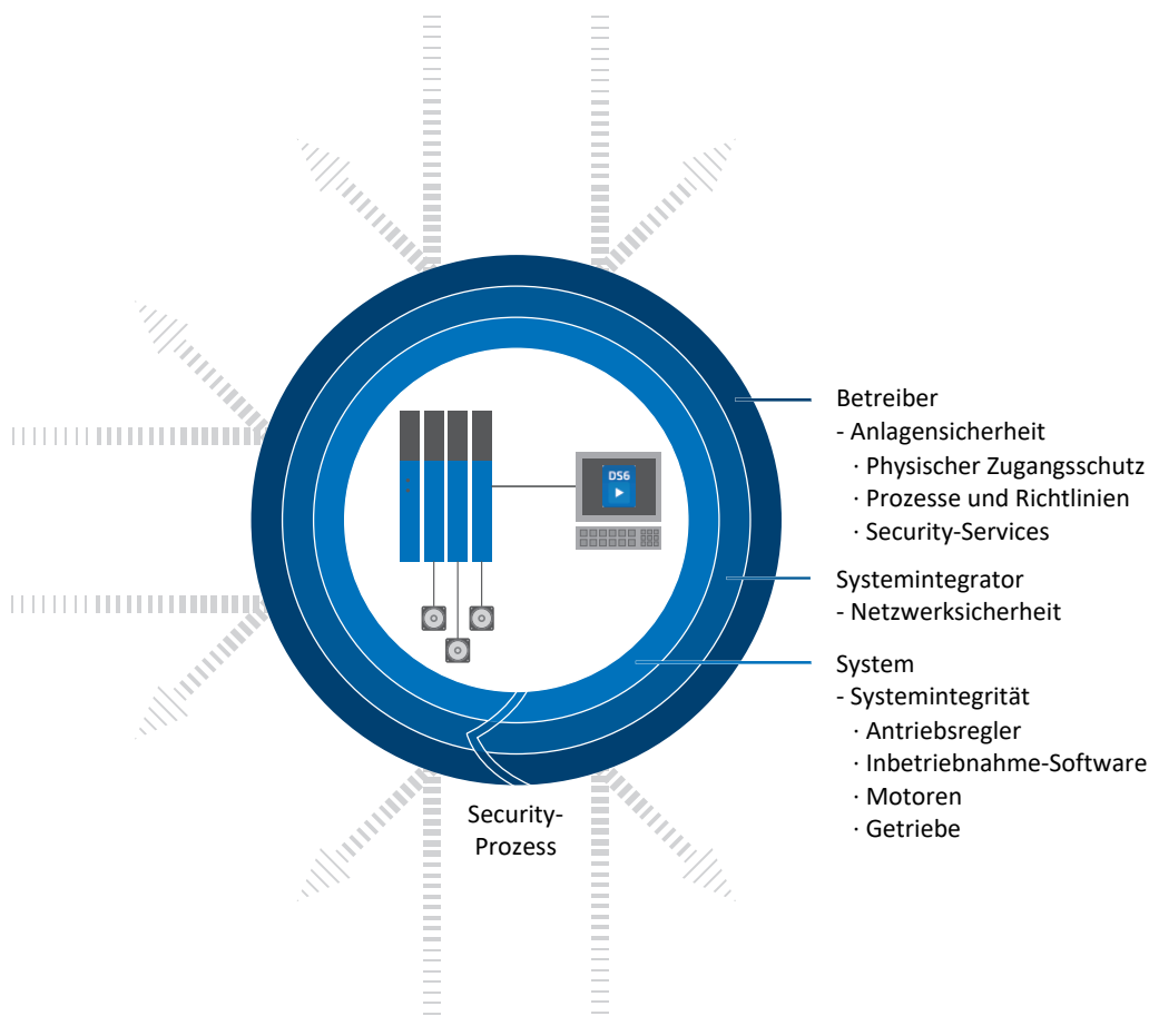
Abb. 1: Defense-in-Depth-Konzept
