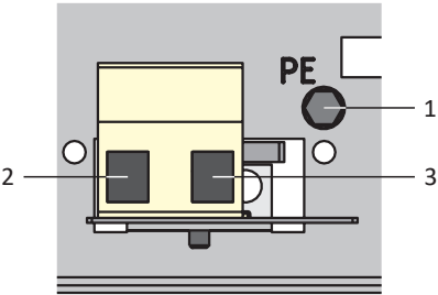
Abb. 29: Anschlussübersicht FZMU
