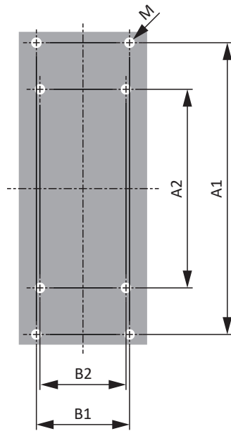
Abb. 20: Bohrplan TEP
