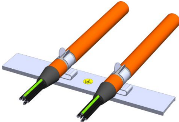
Abb. 32: Geschirmter Anschluss des Leistungskabels
