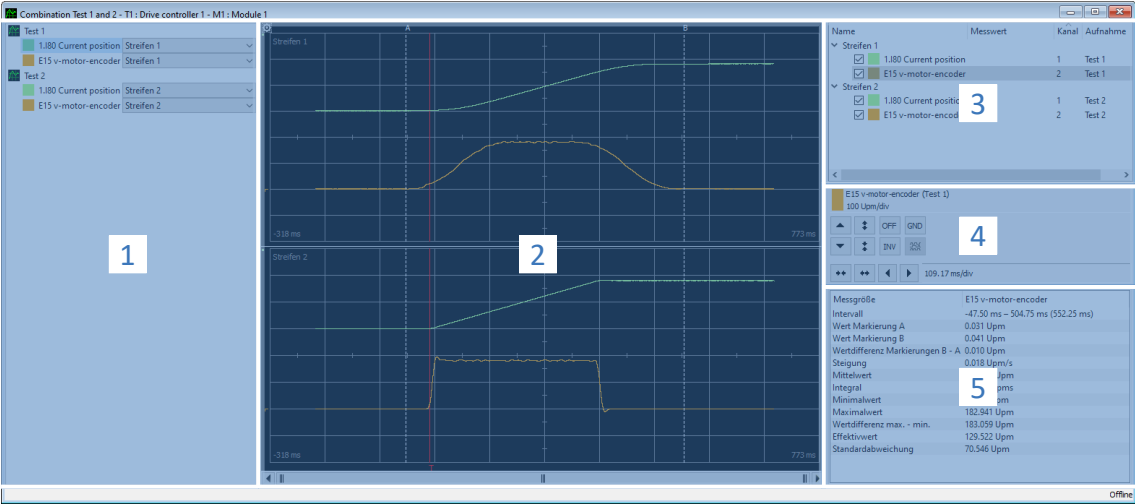
Abb. 73: Scope und Multiachs-Scope: Aufnahmeneditor
