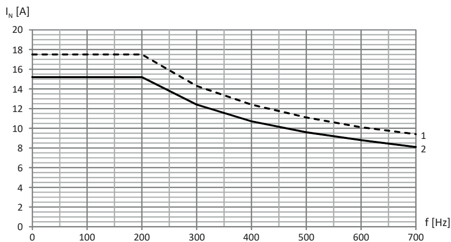
Abb. 10: Derating des Nennstroms in Abhängigkeit von der Taktfrequenz, TEP3820-0CS41
