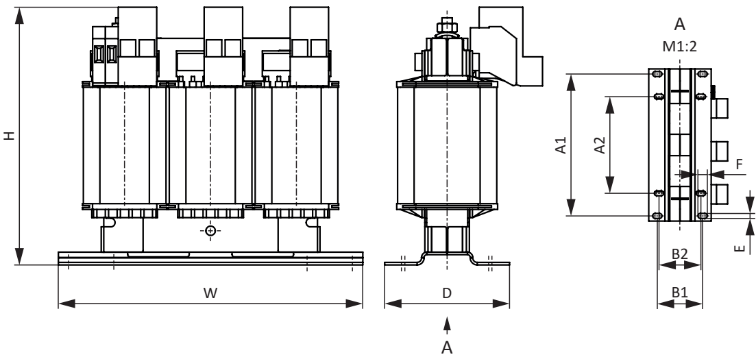
Abb. 8: Maßzeichnung TEP
