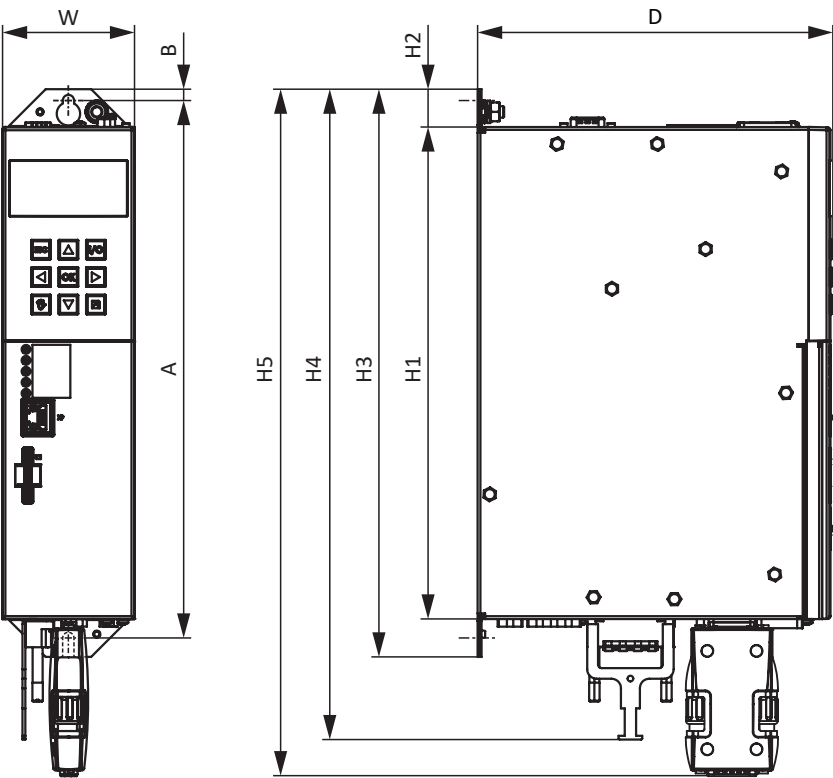
Abb. 5: Maßzeichnung SB6
