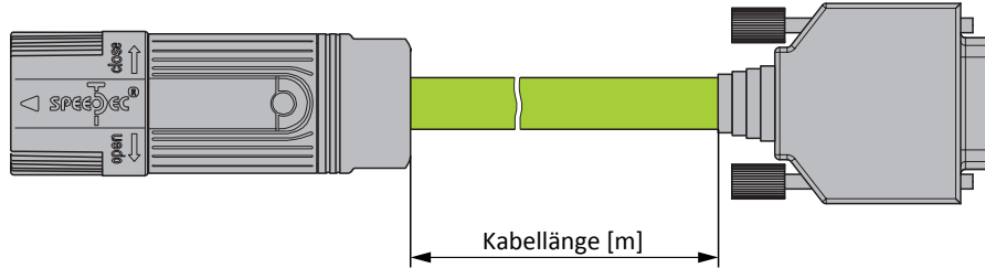
Abb. 1: Längendefinition für konfektionierte Encoderkabel
