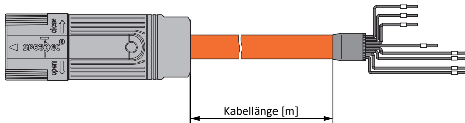
Abb. 2: Längendefinition für konfektionierte Leistungskabel – SB6, SC6, SI6
