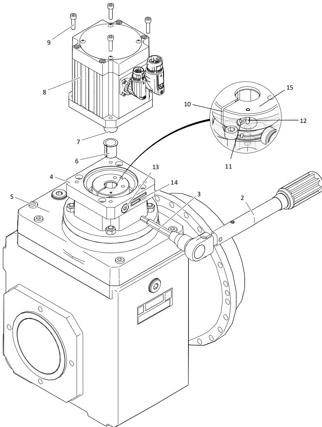
Abb. 2: Montage eines Motors an ein Planetenwinkelgetriebes mit Flanschelle und Motoradapter ME (Beispiel)
