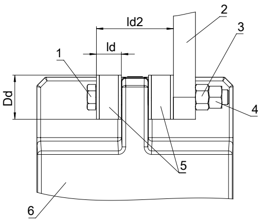
Fig. 5: Montaje de un soporte de par en el reductor F (ejemplo)
