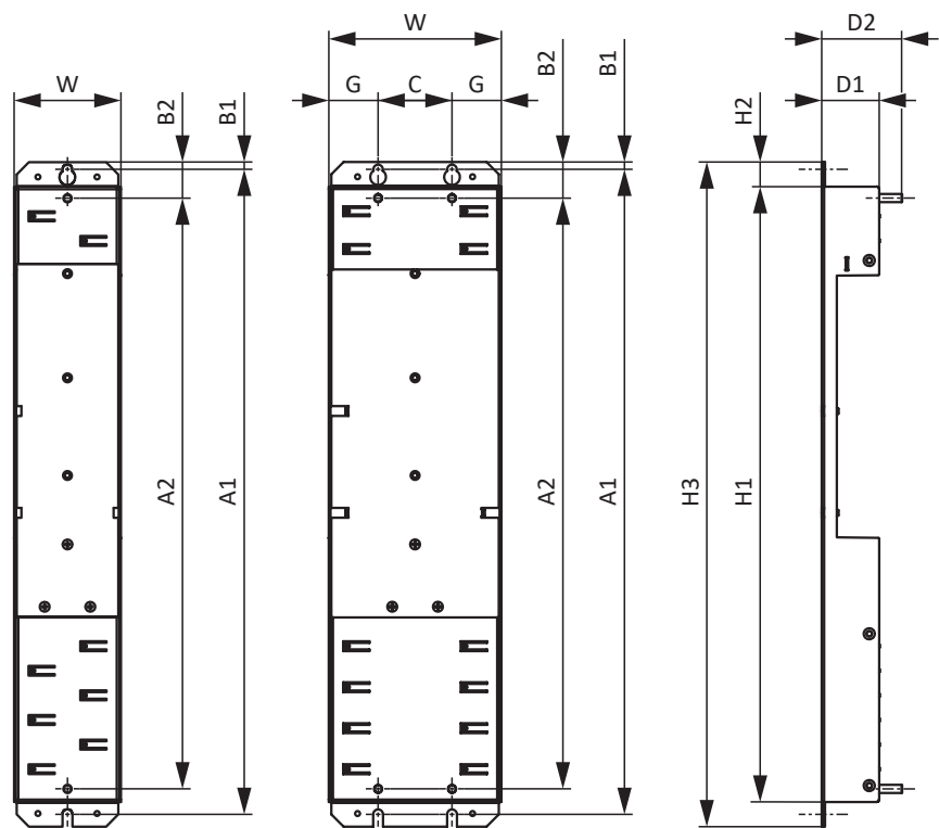
Fig. 5: Croquis coté DL6B10 à DL6B21
