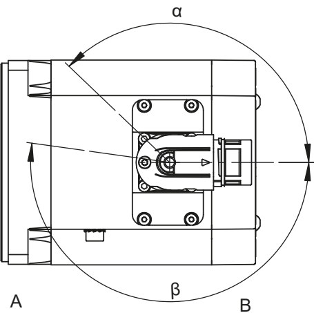
Plages de rotation des connecteurs enfichables (moteurs EZ4 – EZ7)
