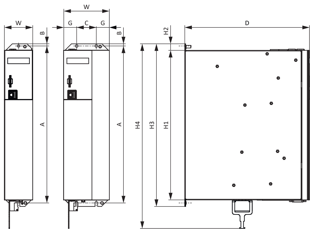
Fig. 2: Croquis coté SI6
