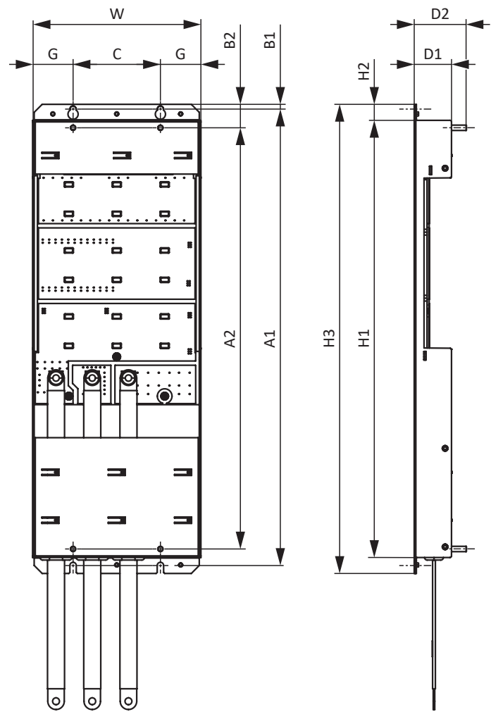
Fig. 6: Croquis coté DL6B22
