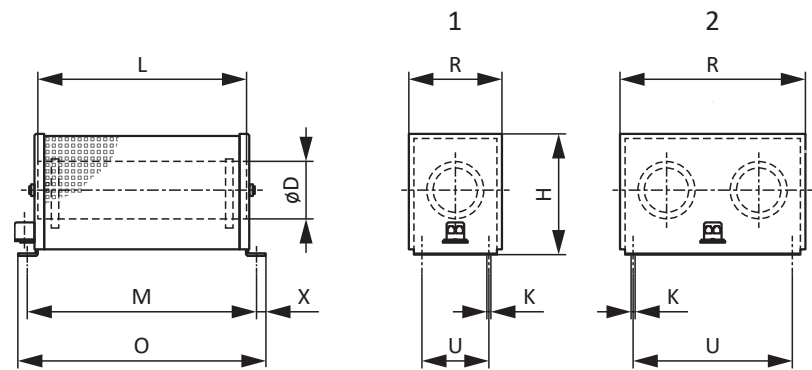
Fig. 4: Croquis coté FZMU (1), FZZMU (2)
