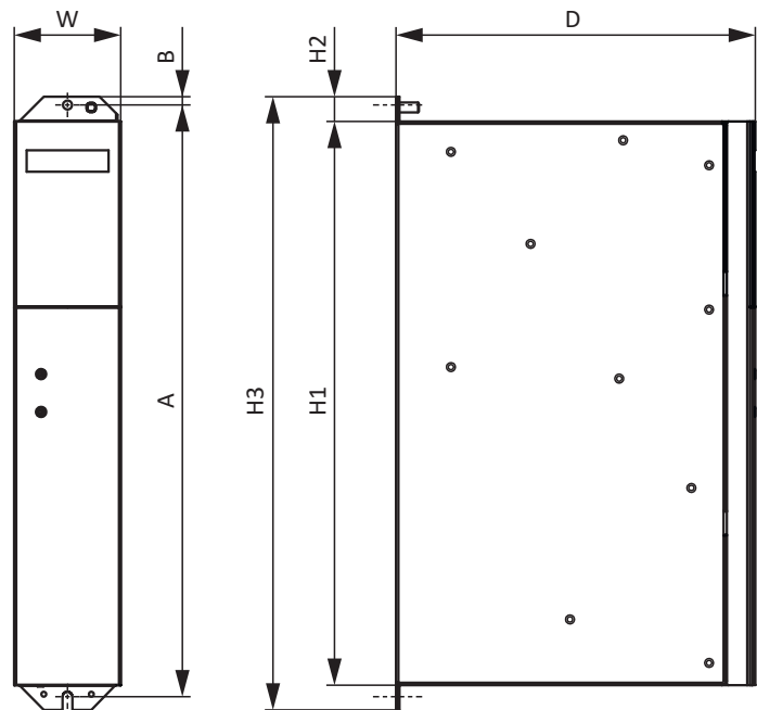
Fig. 3: Croquis coté PS6A24, PS6A34
