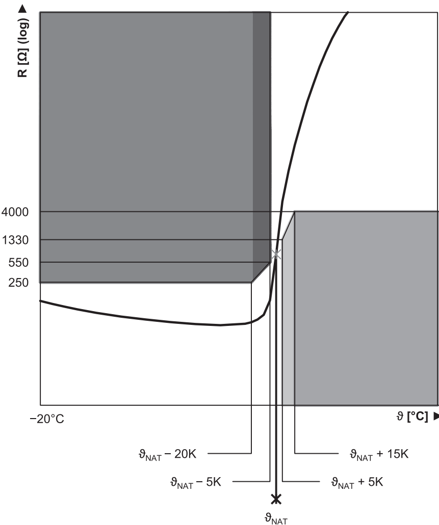
Fig. 2: Courbe caract ristique r sistance CTP (thermistance simple)
