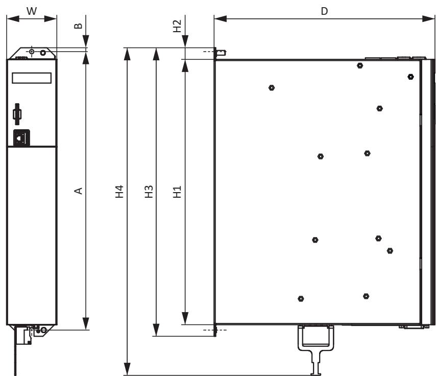
Fig. 2: Croquis coté SC6
