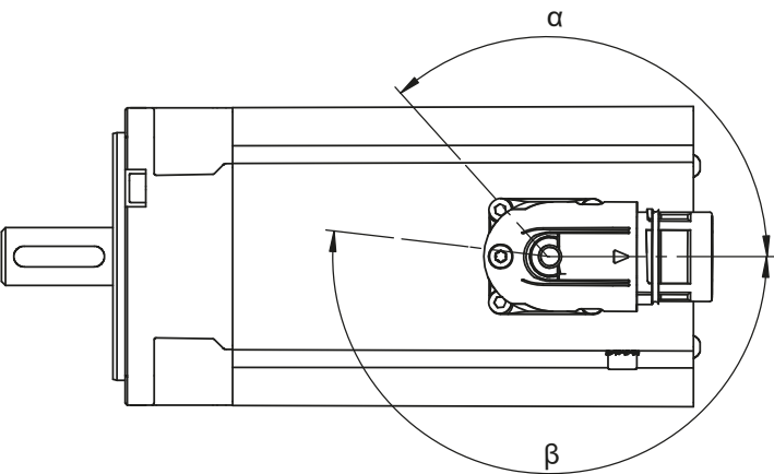
Plages de rotation des connecteurs enfichables (moteurs EZ2 – EZ3)
