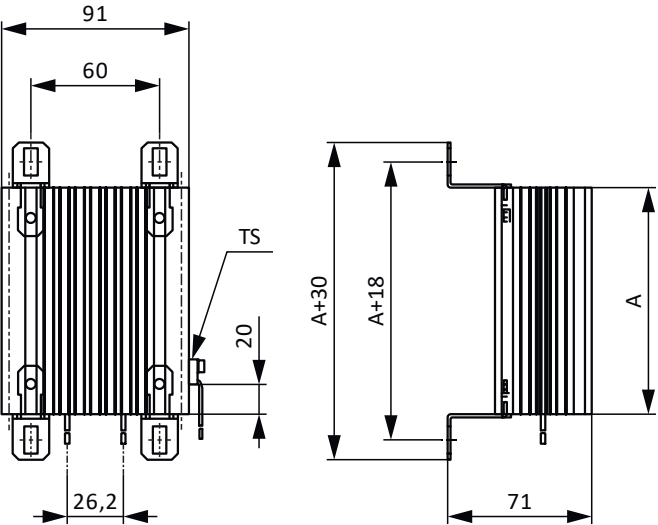
Fig. 9: Croquis coté KWADQU avec MWS306L
