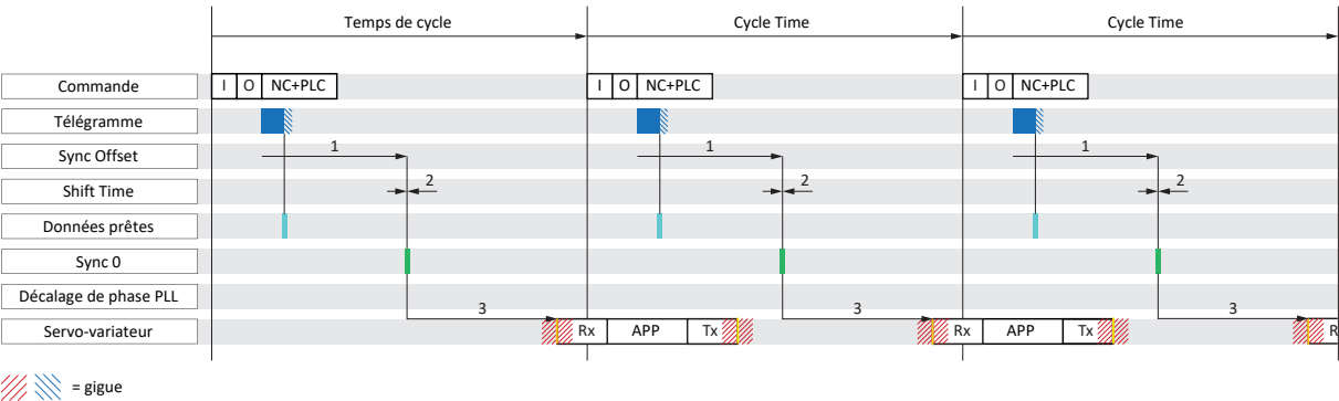
Fig. 17: CODESYS V3 : DC-Sync – Réglages
