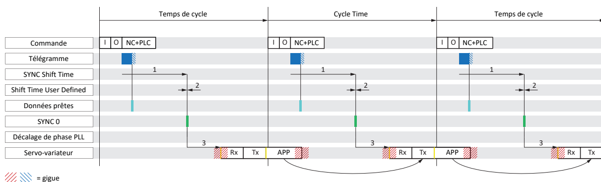
Fig. 16: TwinCAT 3 : DC-Sync – synchronisation stable, temps de cycle < 1 ms
