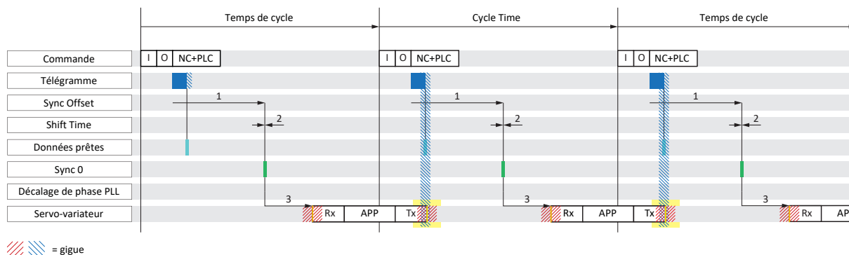
Fig. 18: CODESYS V3 : DC-Sync – synchronisation instable, temps de cycle < 1 ms
