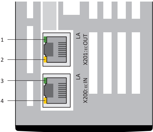
Fig. 7: Diodes électroluminescentes indiquant l'état de la connexion au réseau EtherCAT
