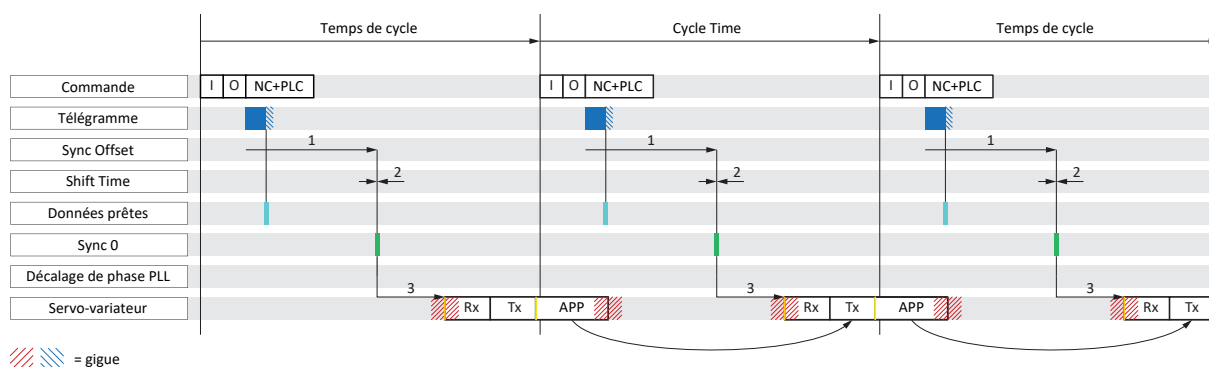
Fig. 19: CODESYS V3 : DC-Sync – synchronisation stable, temps de cycle < 1 ms
