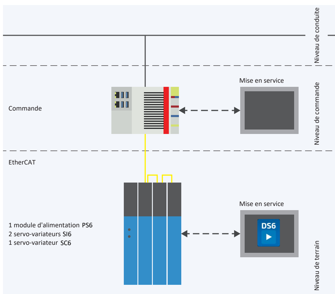
Fig. 1: EtherCAT : structure du réseau
