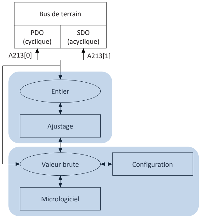
Fig. 20: Aperçu de l'ajustage du bus de terrain
