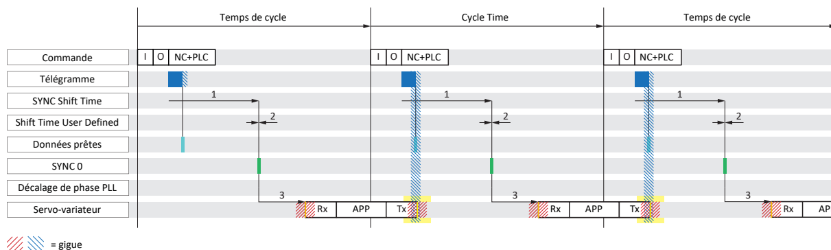
Fig. 15: TwinCAT 3 : DC-Sync – synchronisation instable, temps de cycle < 1 ms
