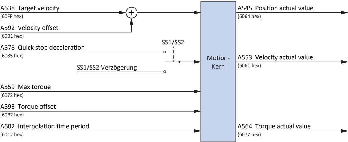
Abb. 14: Cyclic synchronous velocity mode: Ein- und Ausgangssignale
