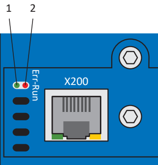
Abb. 6: SD6: Leuchtdioden für den EtherCAT-Zustand
