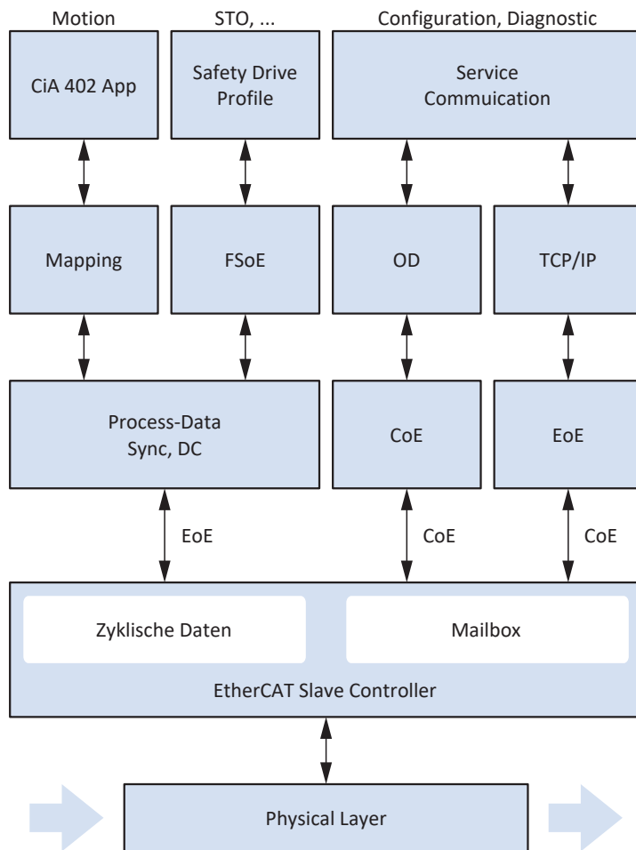
Abb. 8: EtherCAT: Kommunikationsprotokolle
