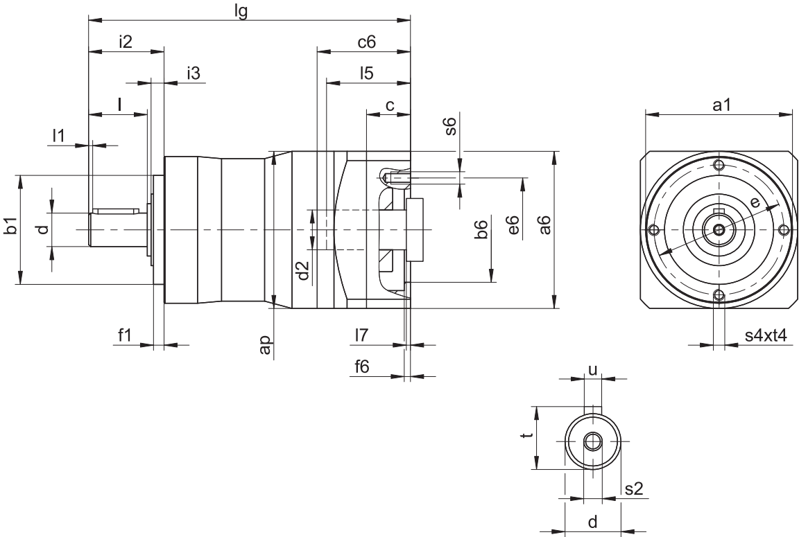
Maße Getriebe
