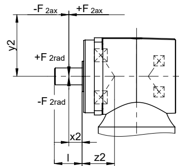
Abb. 5: Kraftangriffspunkte für die Vollwelle
