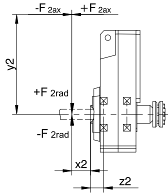
Abb. 4: Kraftangriffspunkte für die Hohlwelle
