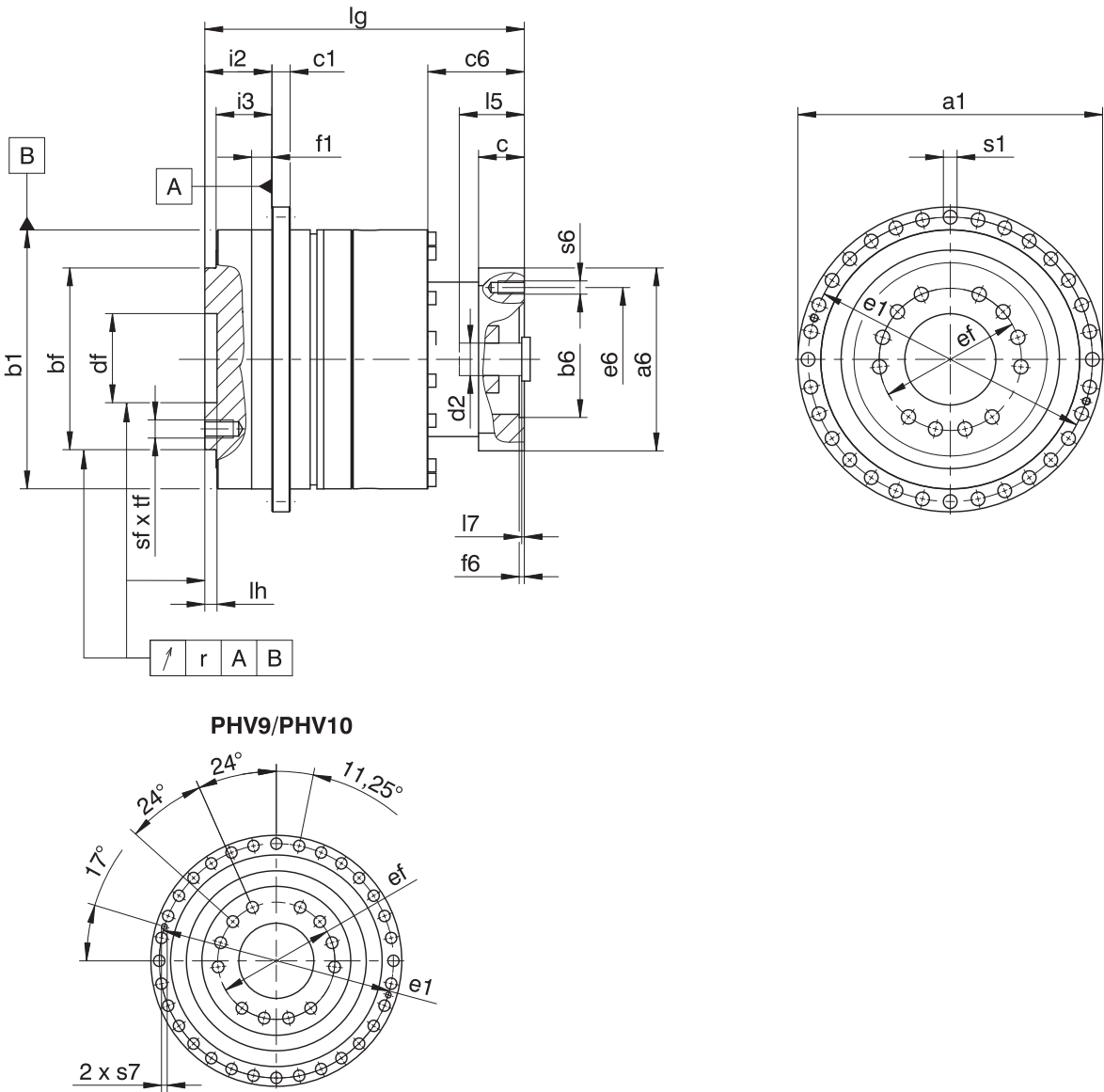
Maße Getriebe
