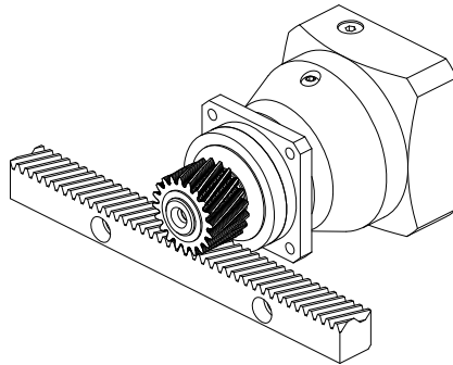
Abb. 4: Empfehlung Lagerzuordnung D (z. B. bei Schrägverzahnung)
