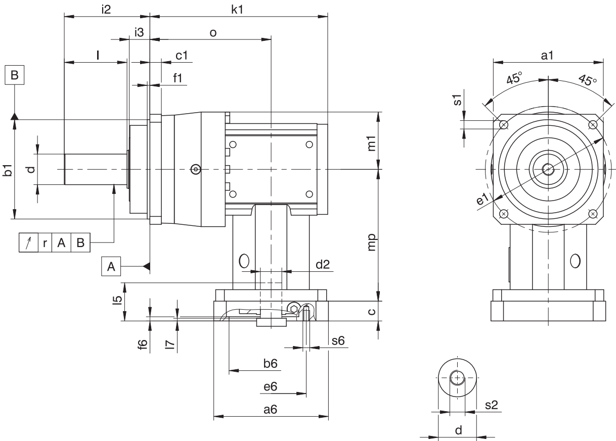
Maße Getriebe
