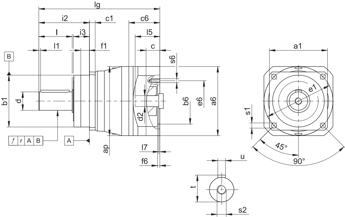
Maße Getriebe
