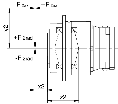
Abb. 3: Kraftangriffspunkte
