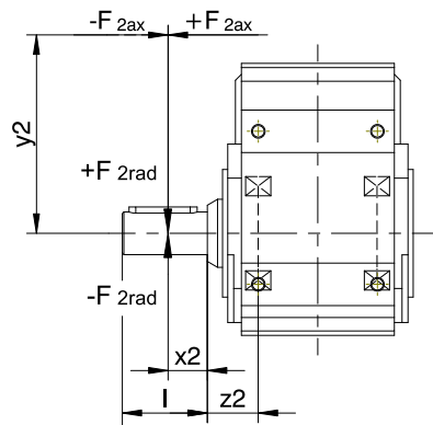
Abb. 3: Kraftangriffspunkte für die Vollwelle
