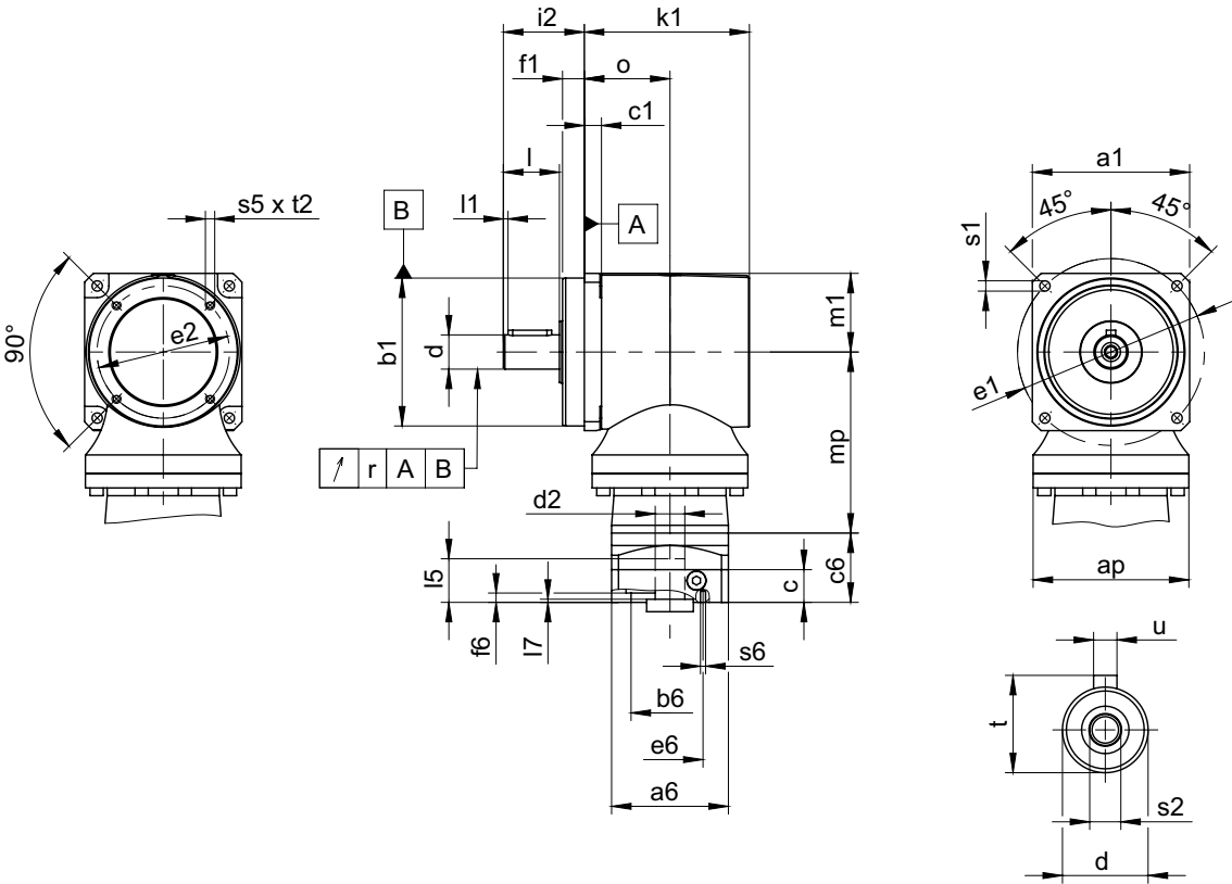
Maße Getriebe
