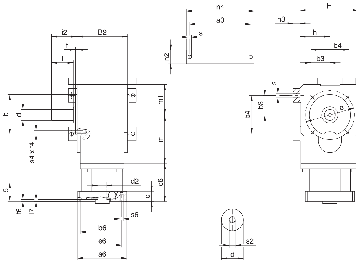
Maße Getriebe
