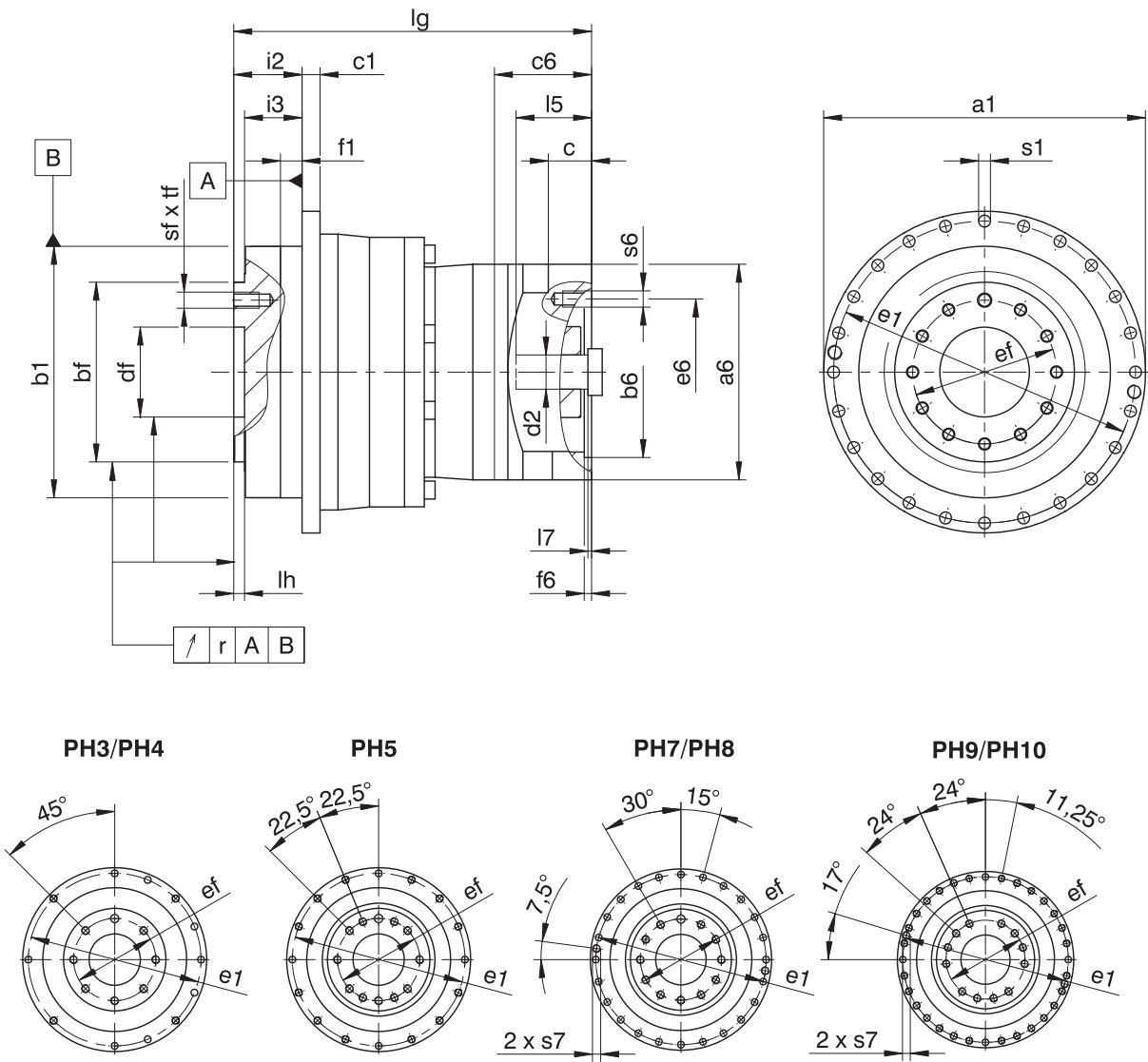
Maße Getriebe
