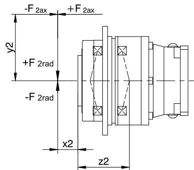
Abb. 2: Kraftangriffspunkte
