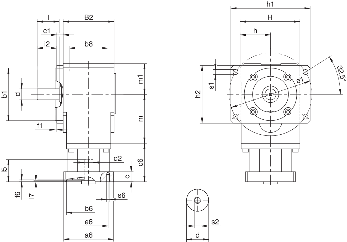
Maße Getriebe
