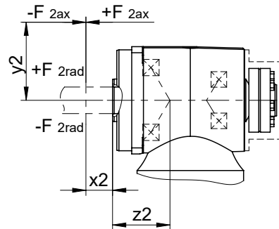
Abb. 4: Kraftangriffspunkte für die Hohlwelle mit Schrumpfscheibe
