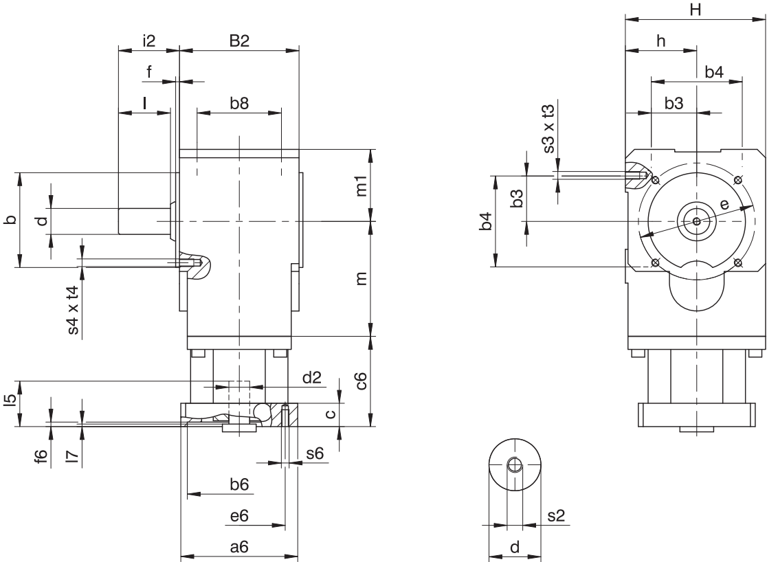
Maße Getriebe
