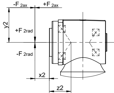
Abb. 3: Kraftangriffspunkte für die Flanschhohlwelle
