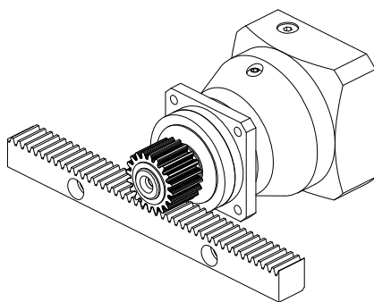
Abb. 3: Empfehlung Lagerzuordnung S (z. B. bei Geradverzahnung)
