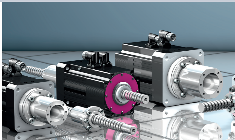
Moteurs brushless pour vis à billes EZS / EZM
