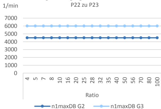
Vergleich Eingangsdrehzahl n1maxDB P22 zu P23
