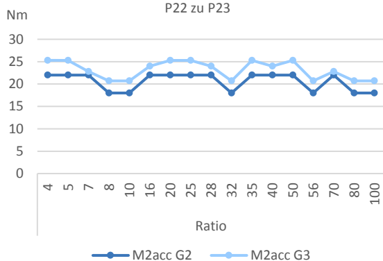
Vergleich Beschleunigungsmomente P22 zu P23
