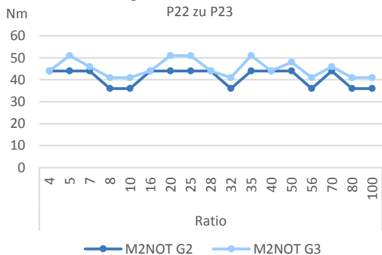
Vergleich NOT-AUS Momente P22 zu P23
