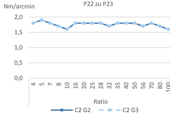
Vergleich Getriebesteifigkeit P22 zu P23
