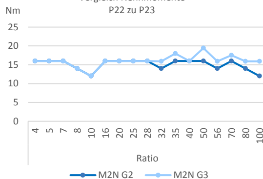
Vergleich Nennmomente P22 zu P23
