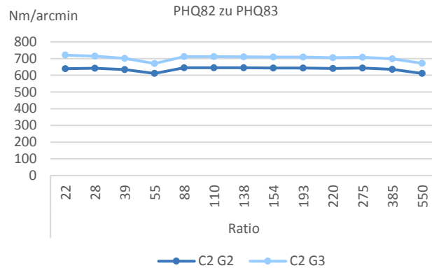
Vergleich Getriebesteifigkeit PHQ82 zu PHQ83
