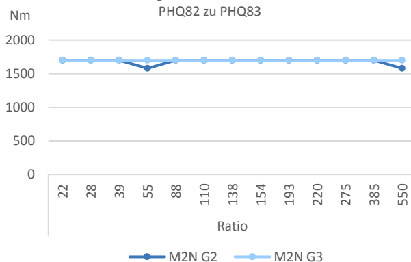
Vergleich Nennmomente PHQ82 zu PHQ83
