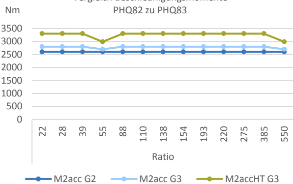
Vergleich Beschleunigungsmomente PHQ82 zu PHQ83
