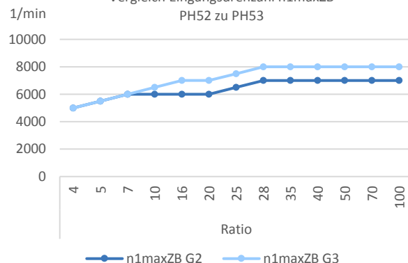
Vergleich Eingangsrehzahl n1maxZB PH52 zu PH53
