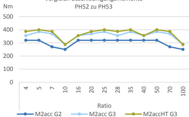
Vergleich Beschleunigungsmomente PH52 zu PH53
