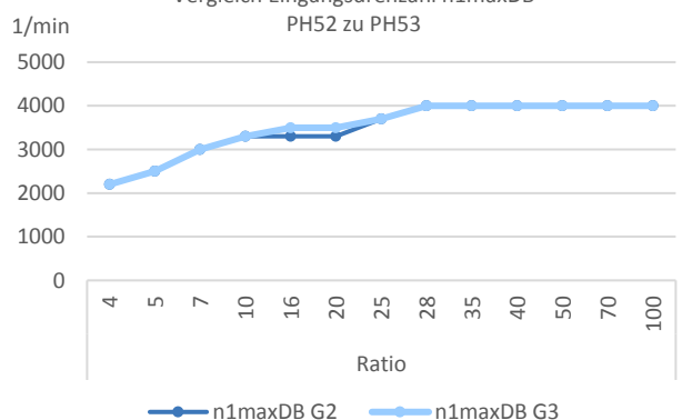
Vergleich Eingangsrehzahl n1maxDB PH52 zu PH53
