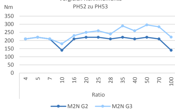
Vergleich Nennmomente PH52 zu PH53
