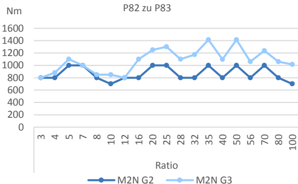
Vergleich Nennmomente P82 zu P83
