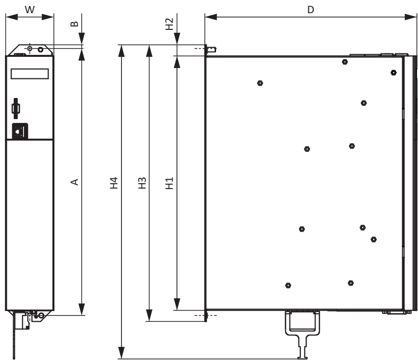
Abb. 6: Maßzeichnung SC6
