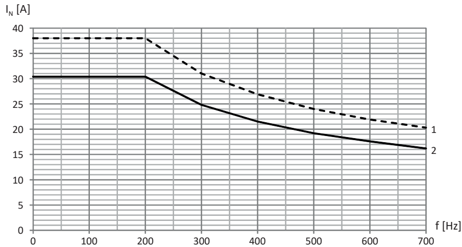
Abb. 14: Derating des Nennstroms in Abhängigkeit von der Taktfrequenz, TEP4020-ORS41
