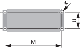
Abb. 22: Bohrplan FZMU, FZZMU
