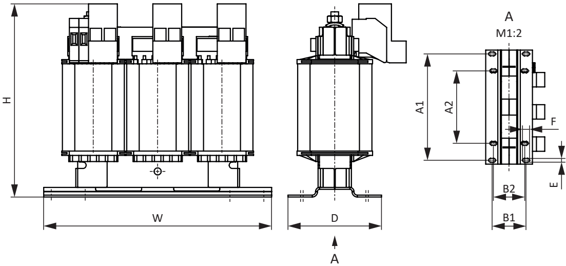
Abb. 10: Maßzeichnung TEP
