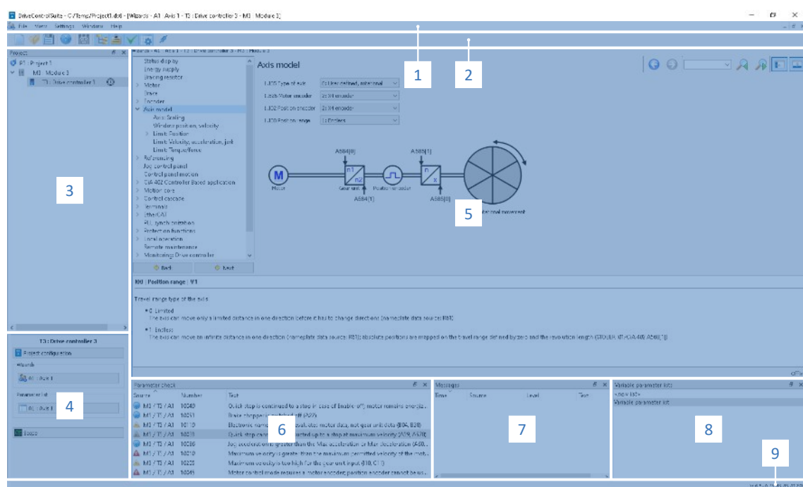
Abb. 34: DS6: Programmoberfläche
