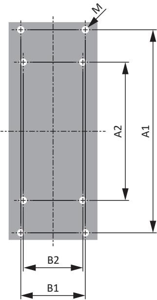
Abb. 24: Bohrplan TEP
