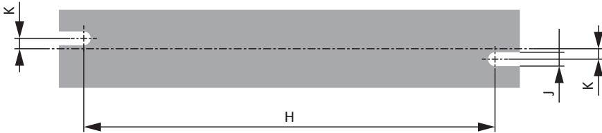
Abb. 23: Bohrplan GVADU, GBADU
