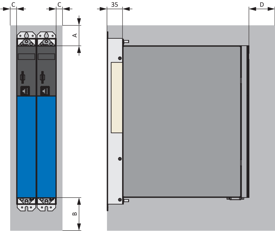
Abb. 20: Mindestfreiräume
