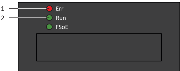
Abb. 63: Leuchtdioden für den EtherCAT-Zustand
