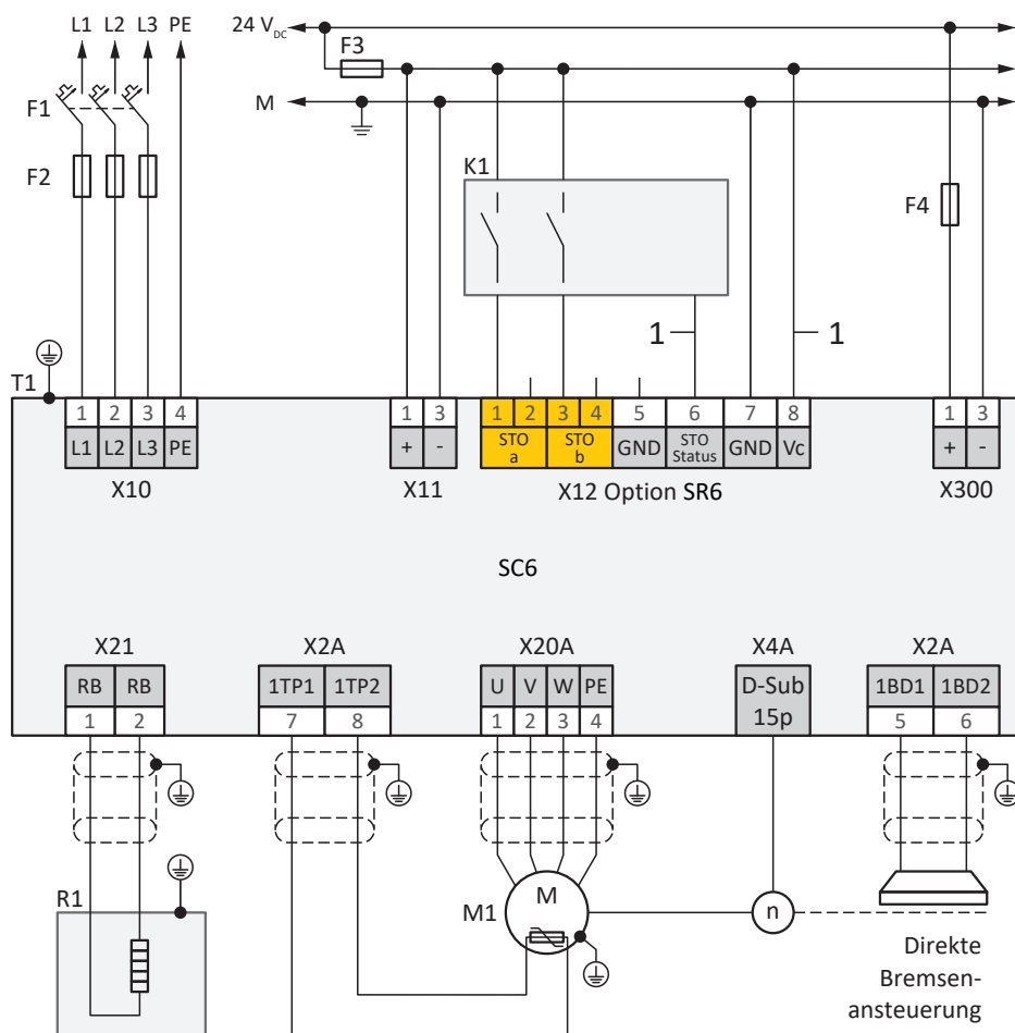
Abb. 74: Verschaltungsbeispiel mit direkter Bremsenansteuerung
