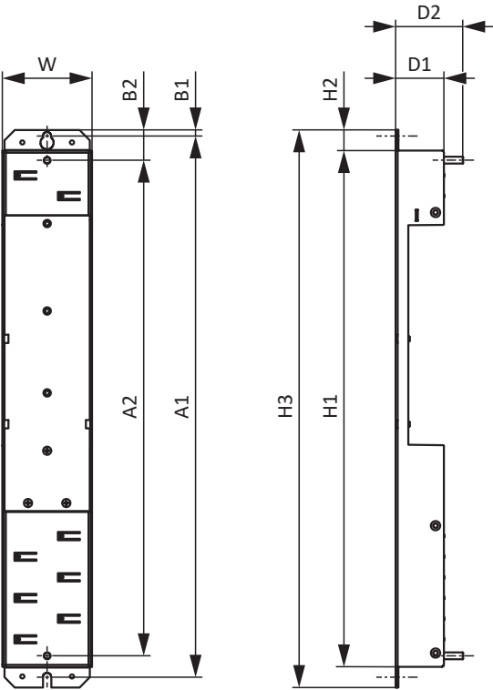
Abb. 7: Maßzeichnung DL6B
