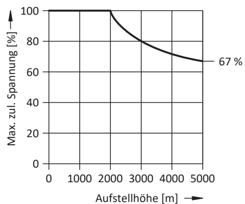
Abb. 17: Derating der Spannung in Abhängigkeit von der Aufstellhöhe
