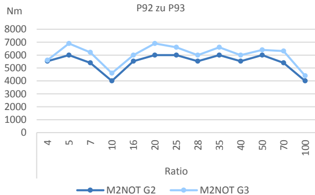
Vergleich NOT-AUS Momente P92 zu P93
