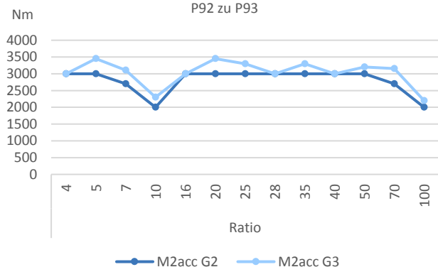
Vergleich Beschleunigungsmomente P92 zu P93
