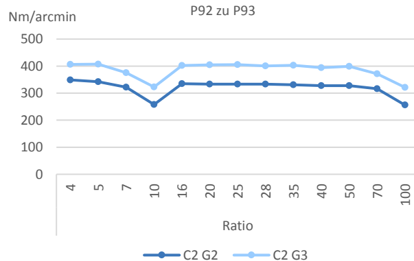
Vergleich Getriebesteifigkeit P92 zu P93
