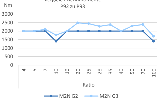
Vergleich Nennmomente P92 zu P93
