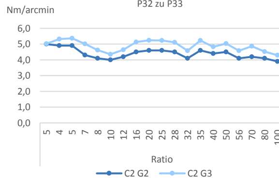
Vergleich Getriebesteifigkeit P32 zu P33
