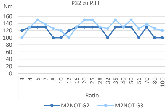
Vergleich NOT-AUS Momente P32 zu P33
