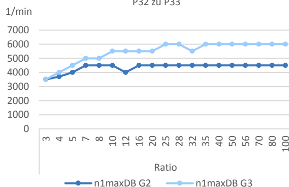
Vergleich Eingangs-drehzahl n1maxDB P32 zu P33
