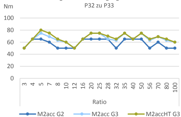
Vergleich Beschleunigungsmomente P32 zu P33
