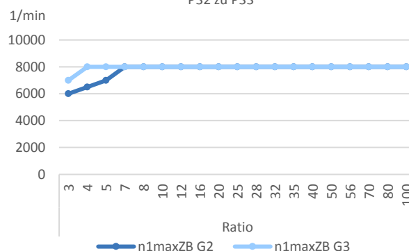
Vergleich Eingangs-drehzahl n1maxZB P32 zu P33
