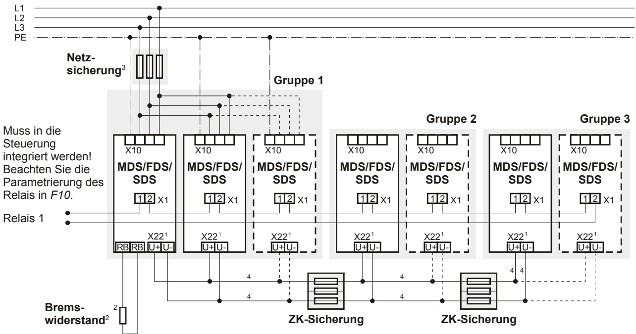
Abb. 5-1 Prinzipschaltbild der Zwischenkreiskopplung
