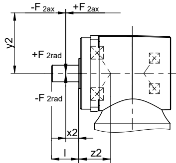
图 5: 实心轴受力点
