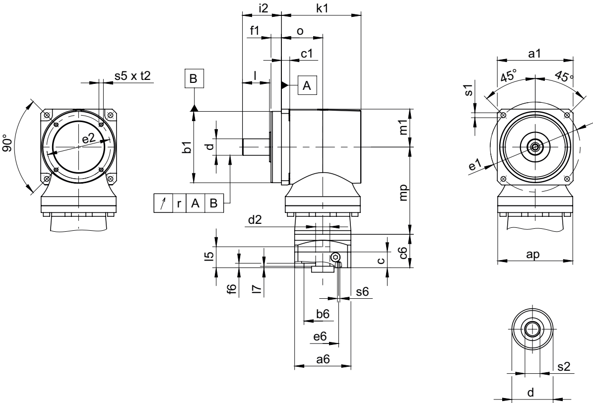
减速器尺寸
