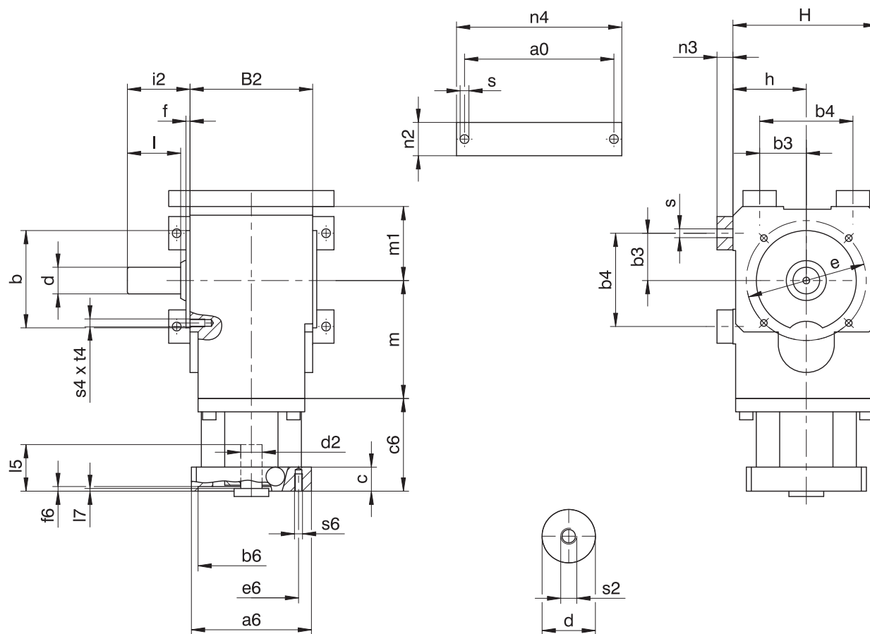
减速器尺寸
