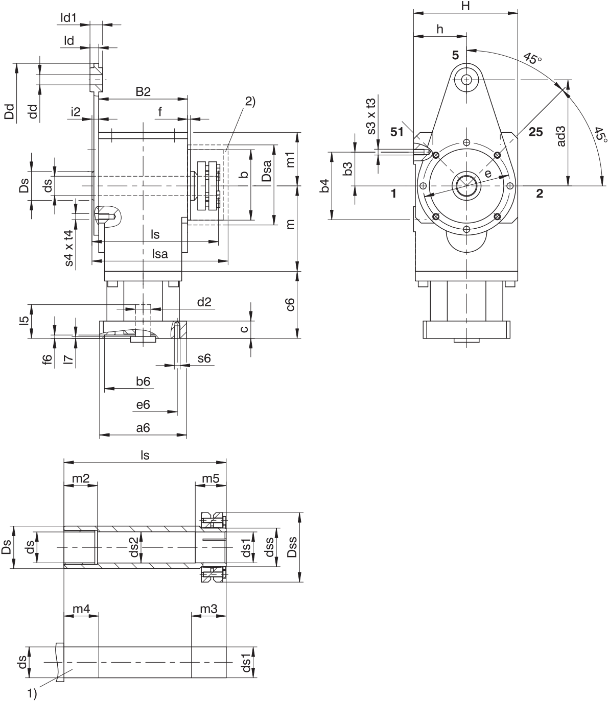
1) 机器轴：不得低于尺寸 ls。 2) 顶盖（选配）
