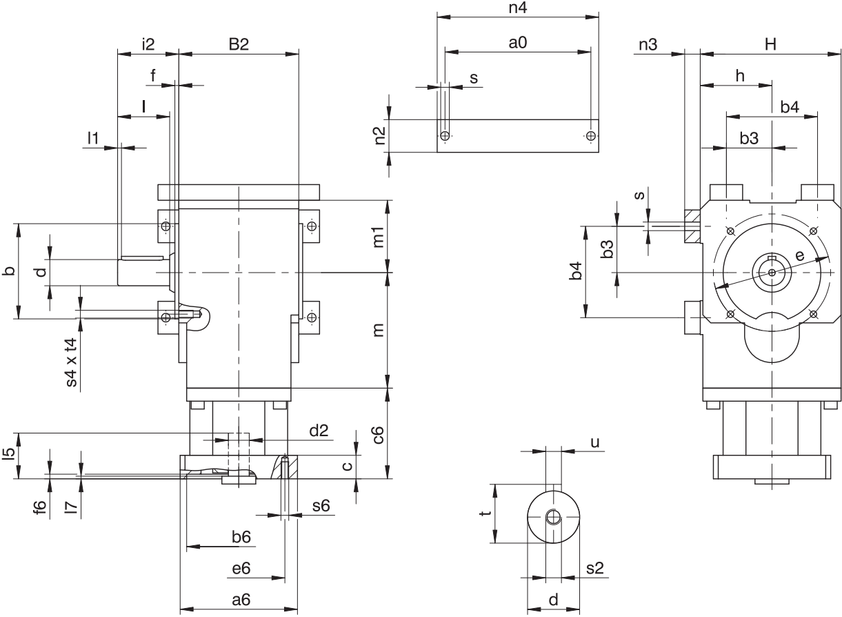
减速器尺寸
