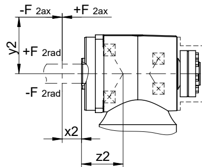
图 4: 带有收缩盘的空心轴的受力点
