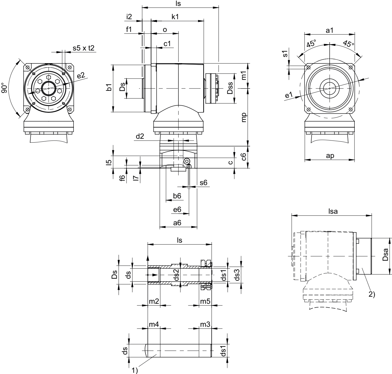
1) 机器轴：不得低于尺寸 ls。 2) 顶盖（选配）
