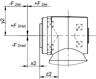
图 3: 法兰空心轴受力点
