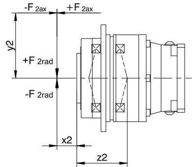
图 2: 受力点
