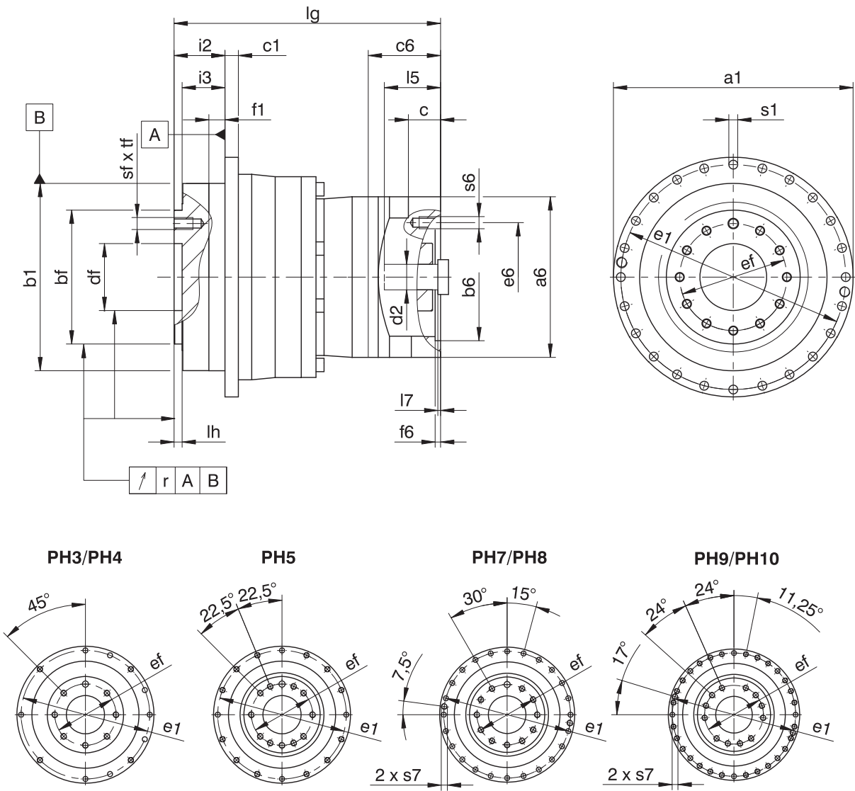
减速器尺寸
