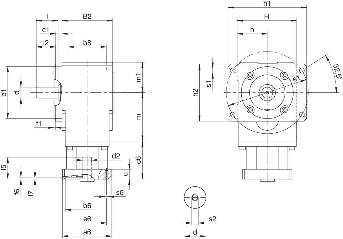
减速器尺寸
