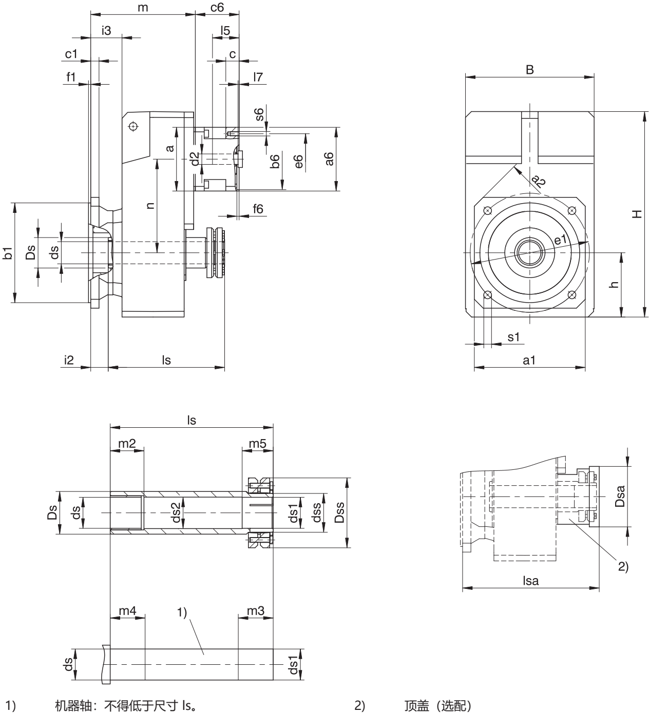
减速器尺寸
