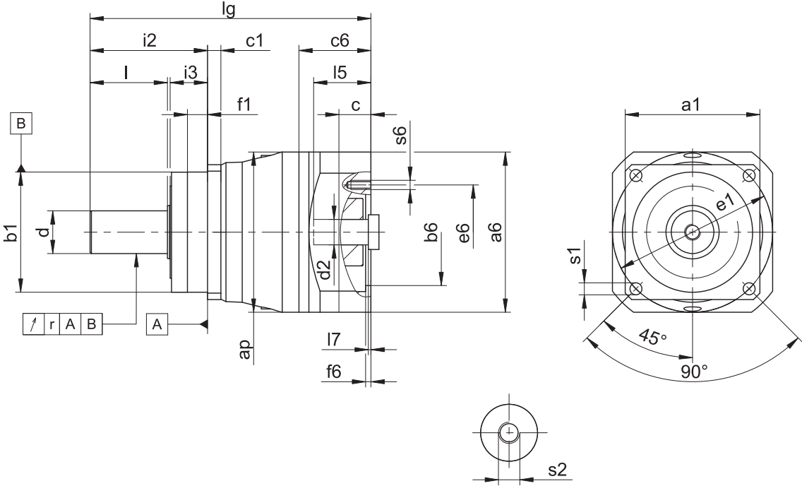
减速器尺寸
