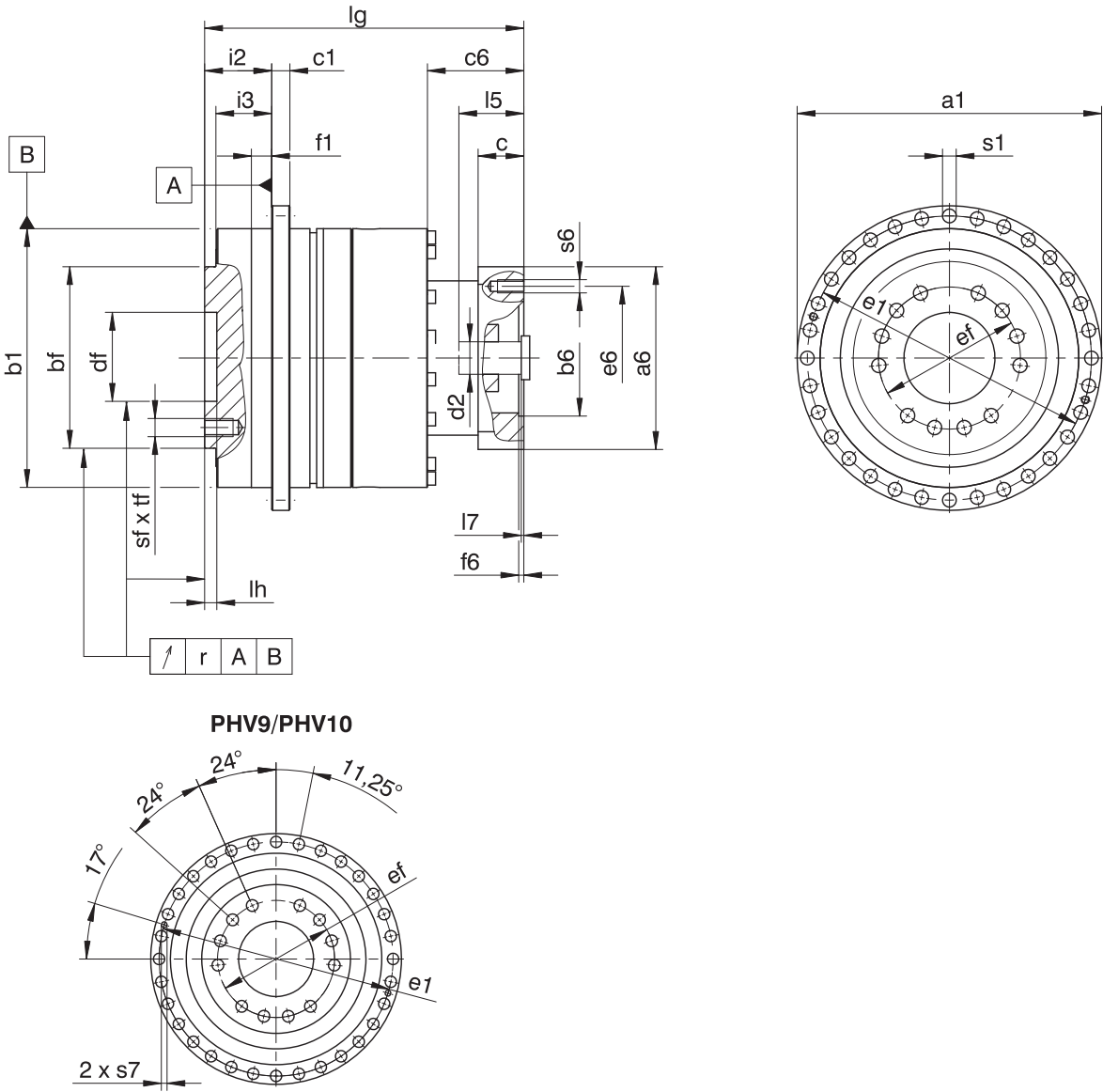
减速器尺寸
