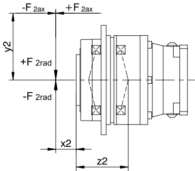
图 2: 受力点
