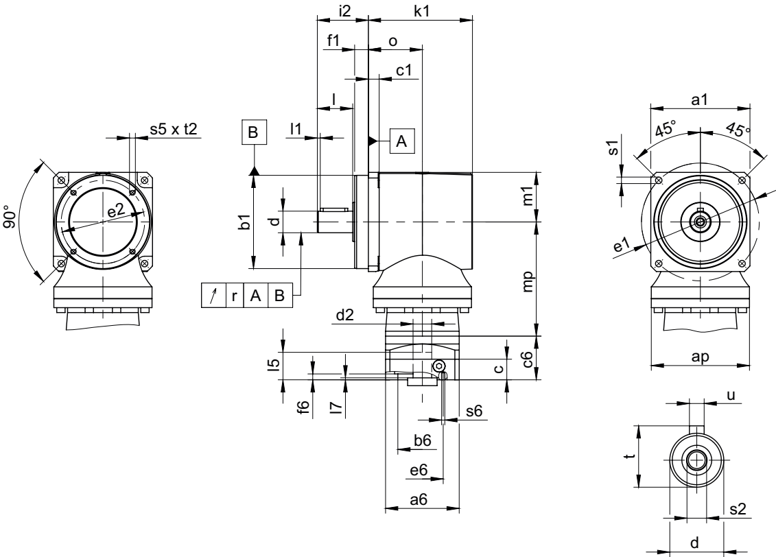
减速器尺寸
