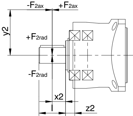
图 2: 受力点
