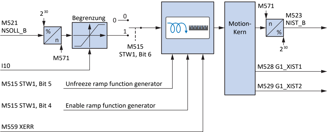
Abb. 35: Standardtelegramm 5 in AC4: Ein- und Ausgangssignale
