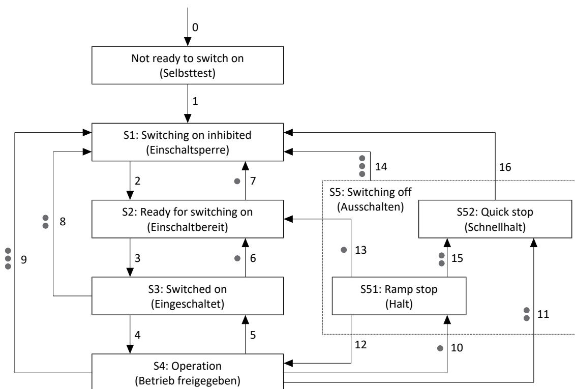
Abb. 45: Gerätezustandsmaschine PROFIdrive: Gerätezustände und Zustandswechsel
