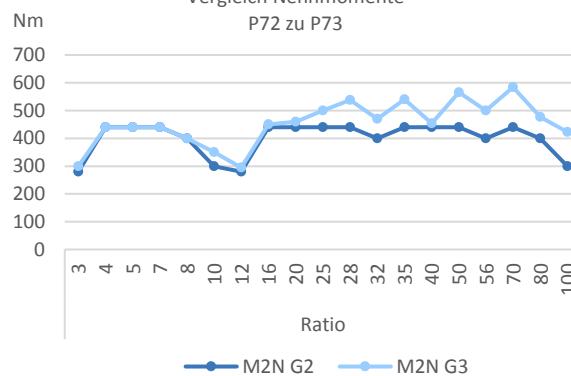
Vergleich Nennmomente P72 zu P73
