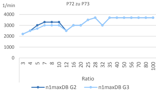
Vergleich Eingangsdrehzahl n1maxDB P72 zu P73
