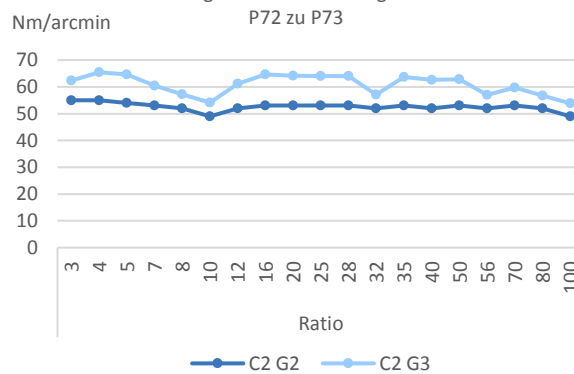
Vergleich Getriebebesteifigkeit P72 zu P73
