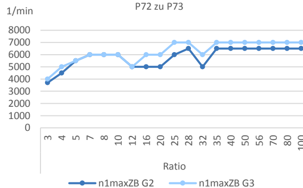
Vergleich Eingangsdrehzahl n1maxZB P72 zu P73
